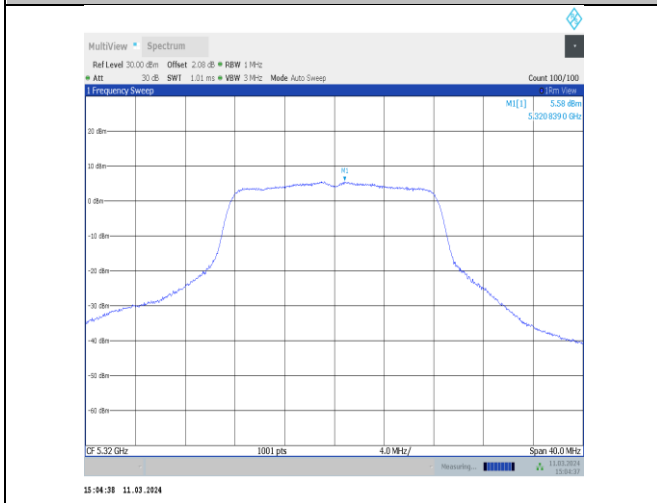
11a-CDD-Ant11-5320-PASS
