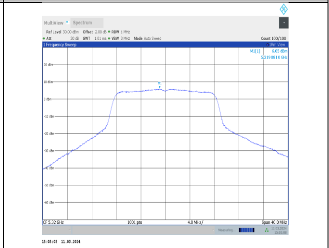
11a-CDD-Ant12-5320-PASS
