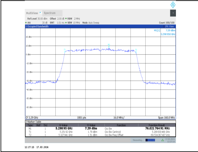
11ac80MIMO-Ant11-5290
