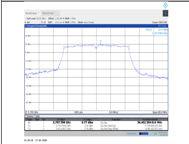
11ac40MIMO-Ant11-5795
