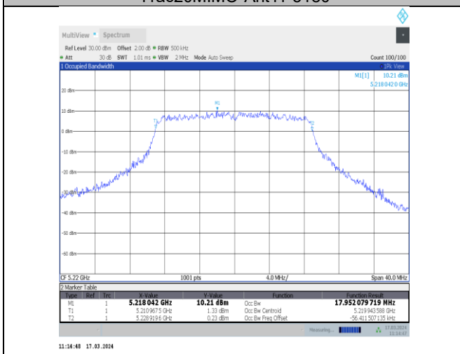
11ac20MIMO-Ant11-5220
