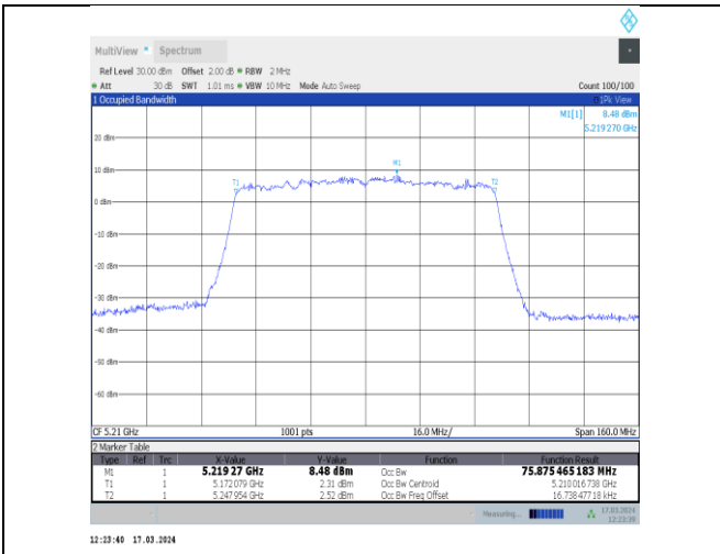
11ac80MIMO-Ant11-5210
