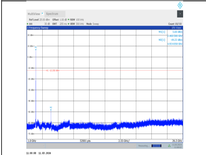
11b-CDD-Ant10-2462-1000~26500-PASS
