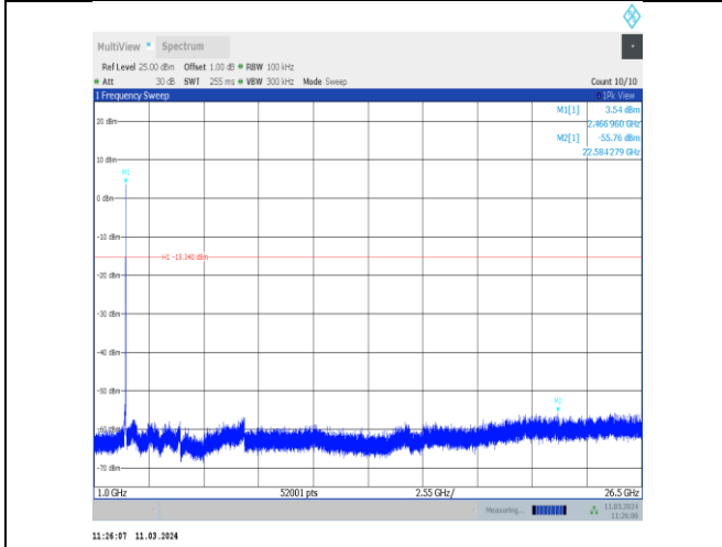
11n20MIMO-Ant10-2462-1000~26500-PASS
