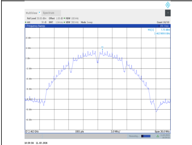
11b-CDD-Ant10-2462-0~Reference-PASS
