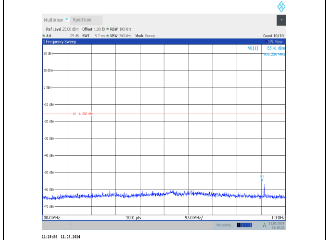
11n20MIMO-Ant10-2412-30~1000-PASS
