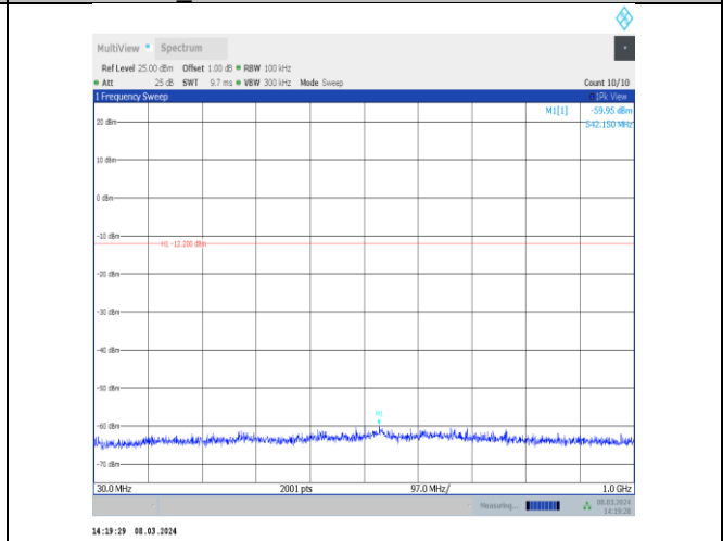
BLE_1M-Ant10-2480-30~1000-PASS
