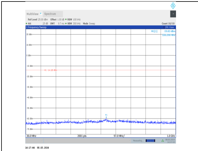
BLE_1M-Ant10-2440-30~1000-PASS
