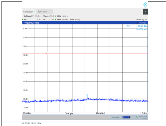
2DH5-Ant10-2402-30~1000-PASS
