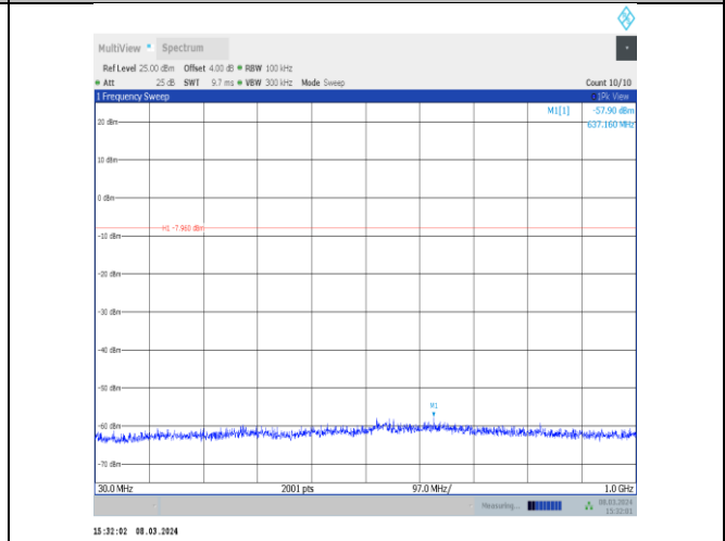
2DH5-Ant10-2441-30~1000-PASS
