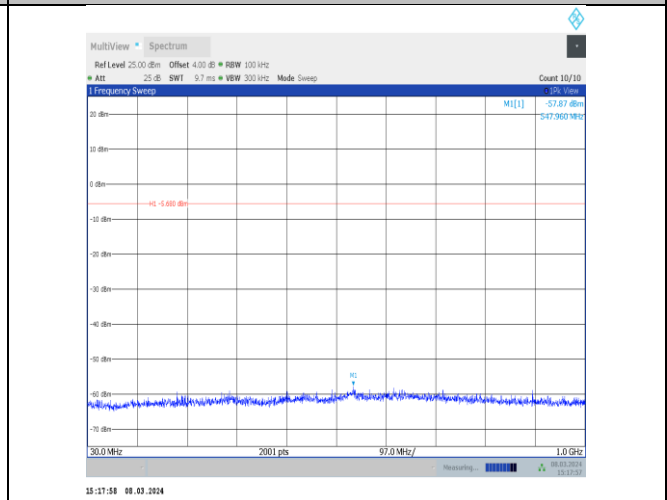
DH5-Ant10-2480-30~1000-PASS
