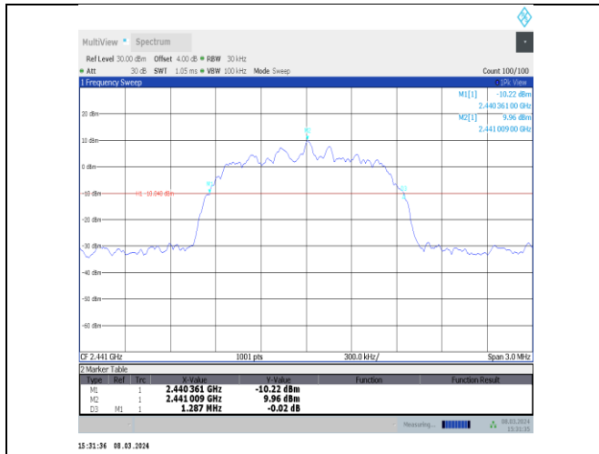
2DH5-Ant10-2441
