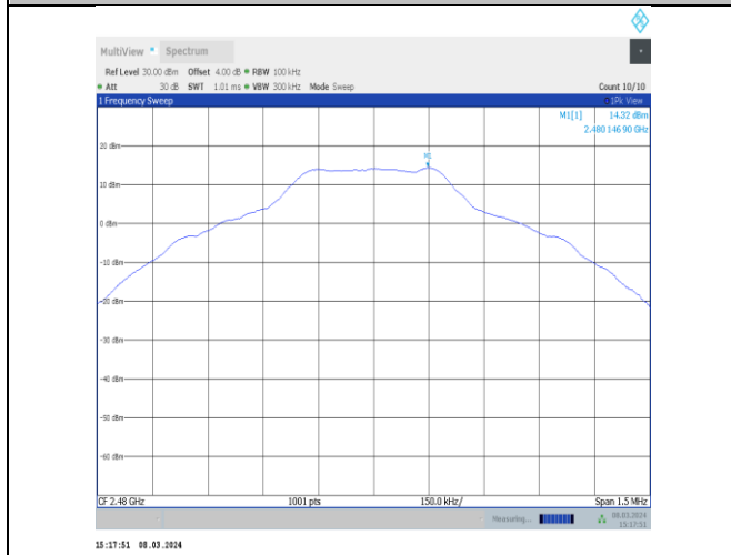
DH5-Ant10-2480-0~Reference-PASS
