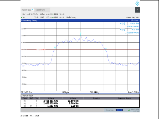
2DH5-Ant10-2402
