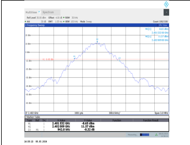
DH5-Ant10-2402
