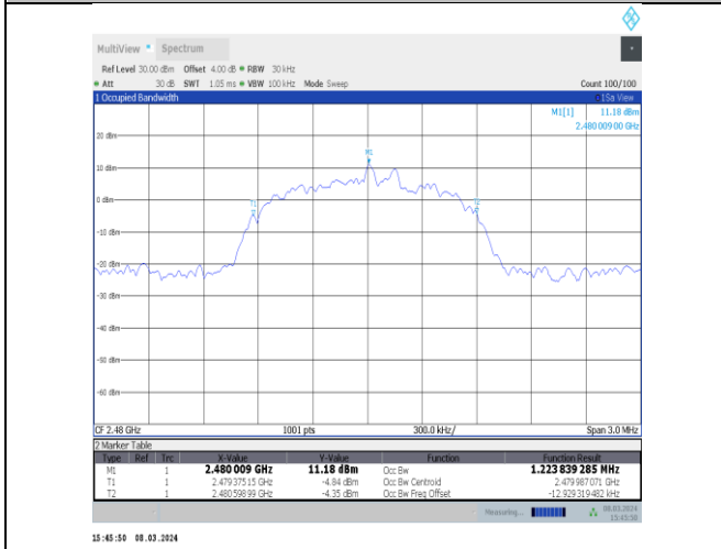
3DH5-Ant10-2480
