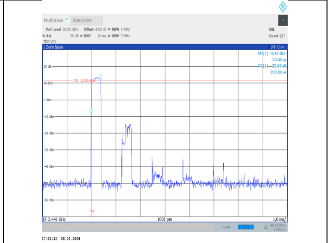
2DH1-Ant10-Hop-PASS
