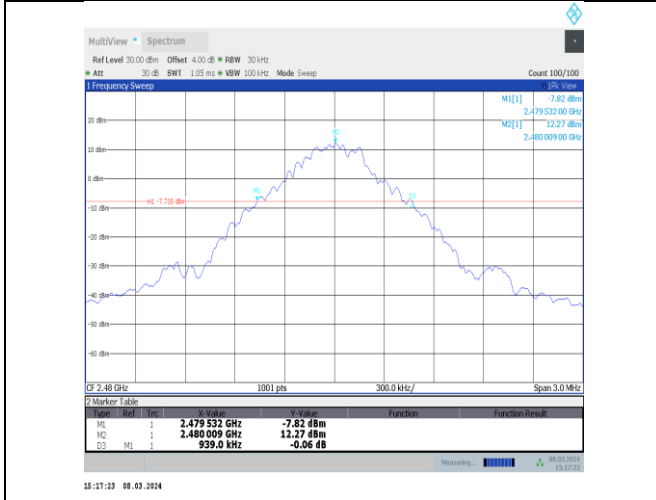
DH5-Ant10-2480
