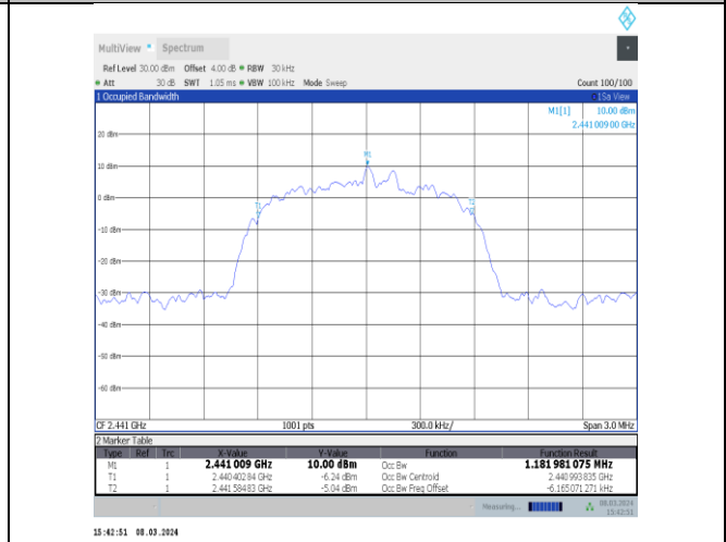
3DH5-Ant10-2441
