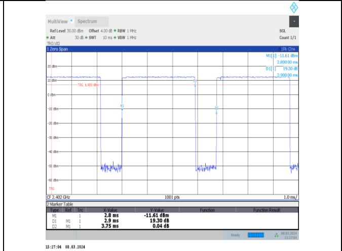
NTNV-2DH5-Ant10-2402
