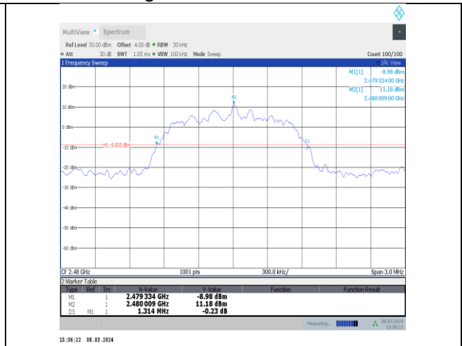
2DH5-Ant10-2480
