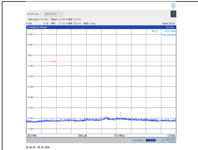
DH5-Ant10-2441-30~1000-PASS
