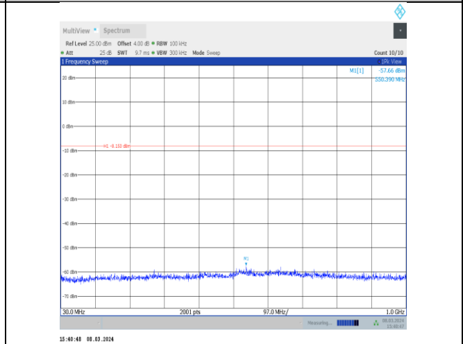
3DH5-Ant10-2402-30~1000-PASS
