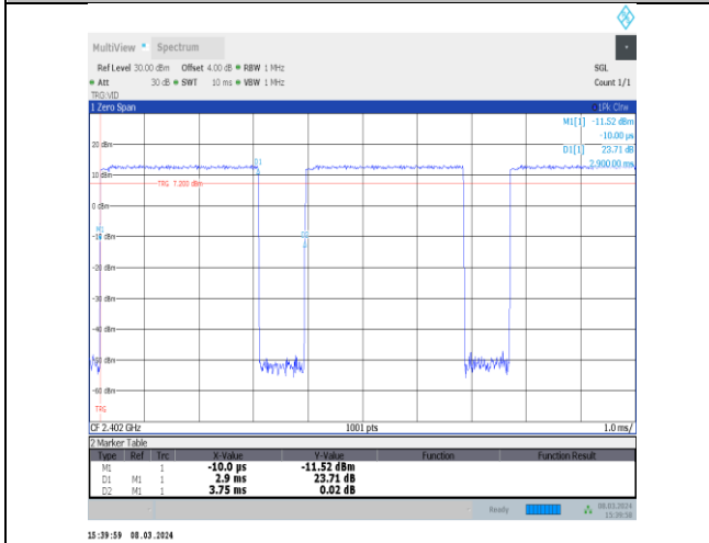
NTNV-3DH5-Ant10-2402
