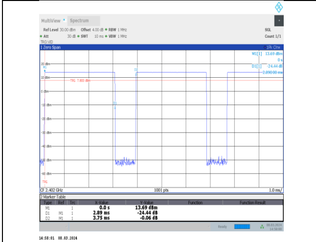
NTNV-DH5-Ant10-2402
