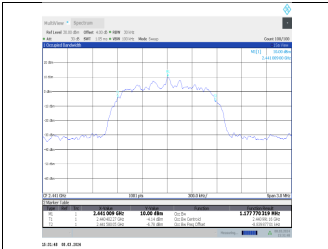
2DH5-Ant10-2441
