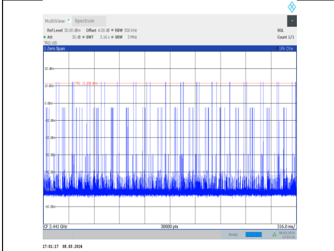
2DH1-Ant10-Hop-PASS
