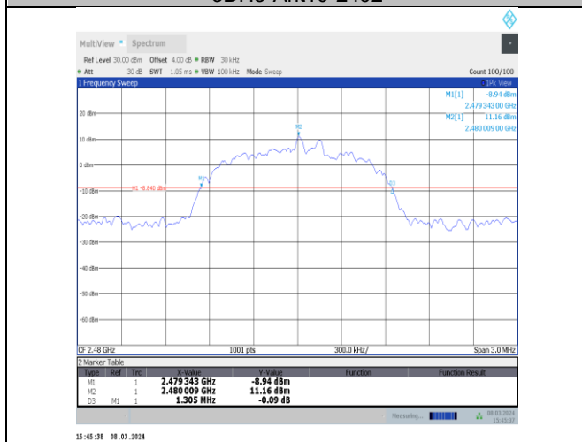
3DH5-Ant10-2480
