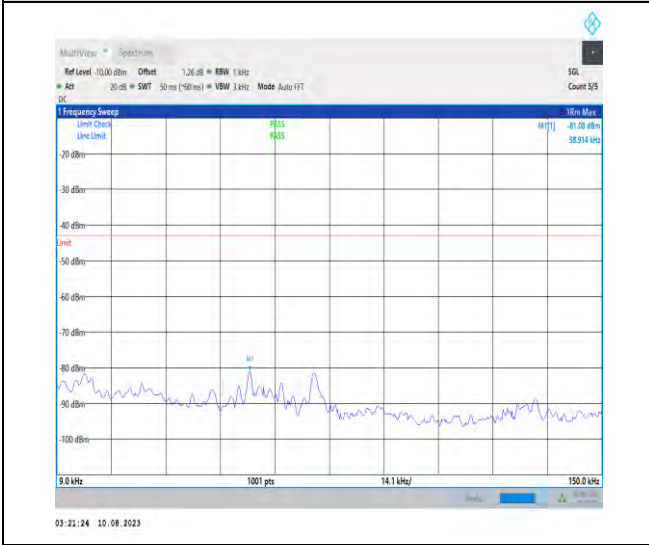
1-N66-PC3-15-40-H-1-N/A-DFT-PI2BPSK-Inner_1R B_Left-1@1-0.009-0.15-Ant1-0.01--81.08--43-PASS
