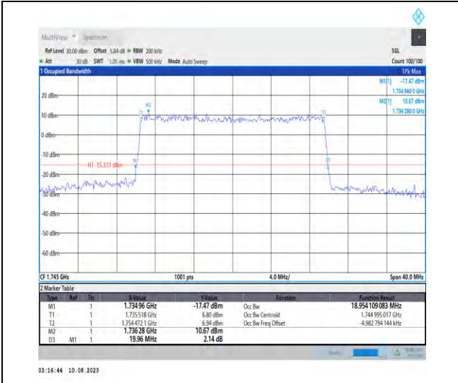
1-N66-PC3-15-20-M-6-CP-QPSK-Outer_Full-106@ 0-Ant1-18.954-19.960-≤20-PASS
