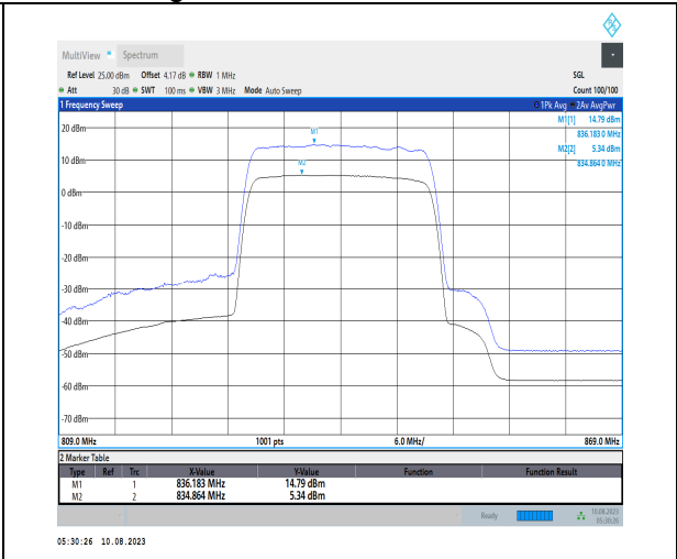
1-N5-PC3-15-20-H-2-CP-256QAM-Outer_Full-106@ 0-Ant1-9.45-100%-0.00-9.45-PASS-≤13
