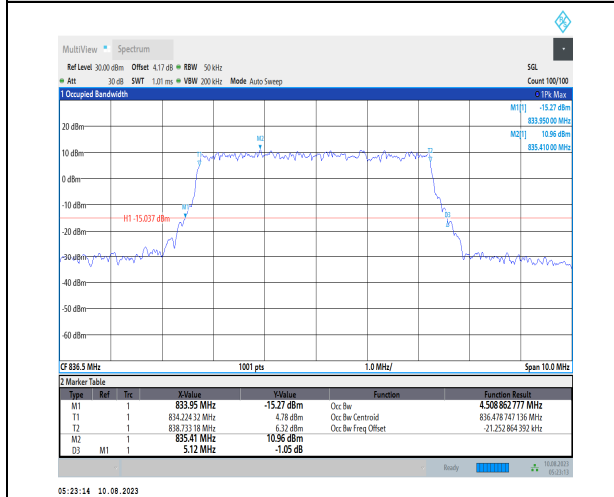
1-N5-PC3-15-5-M-7-CP-16QAM-Outer_Full-25@0-A nt1-4.509-5.120-≤5-PASS
