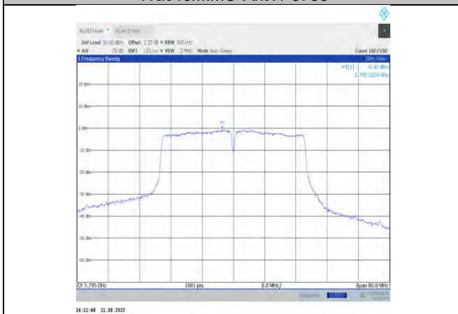
11ac40MIMO-Ant11-5795
