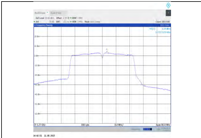
11ac40MIMO-Ant11-5270
