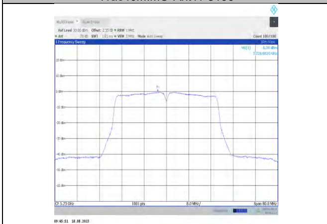
11ac40MIMO-Ant11-5230
