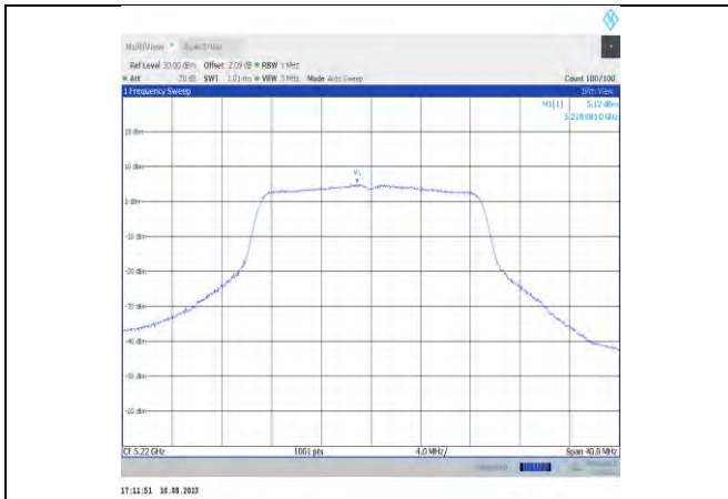
11ac20MIMO-Ant11-5220
