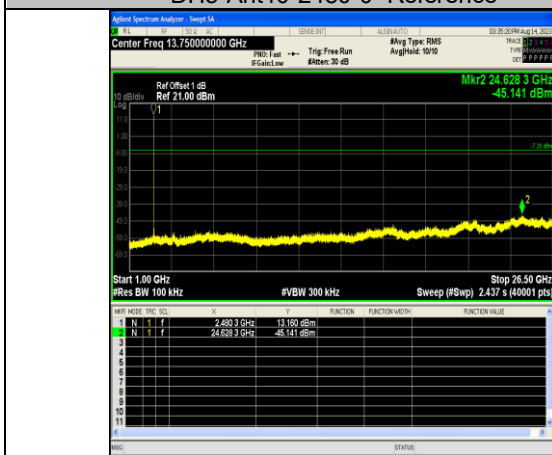
DH5-Ant10-2480-1000~26500
