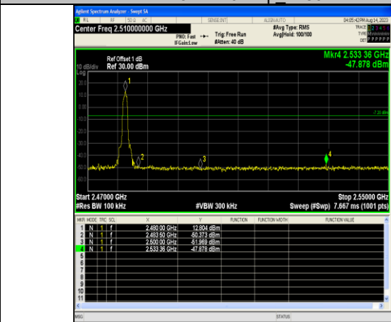
3DH5-Ant10-2480
