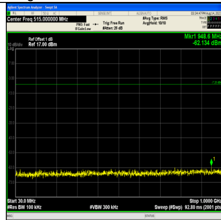
DH5-Ant10-2480-30~1000
