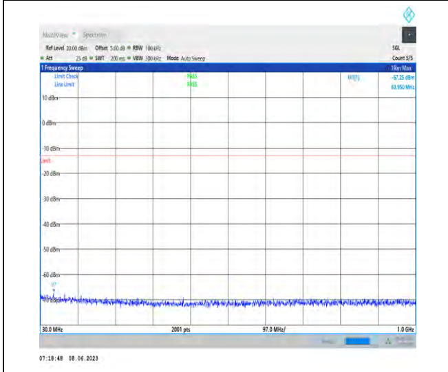
1-N78-3700-3800-PC3-30-100-H-1-N/A-DFT-PI2BP SK-Inner_1RB_Left-1@1-30-1000-Ant1-63.95--67.2 5--13-PASS
