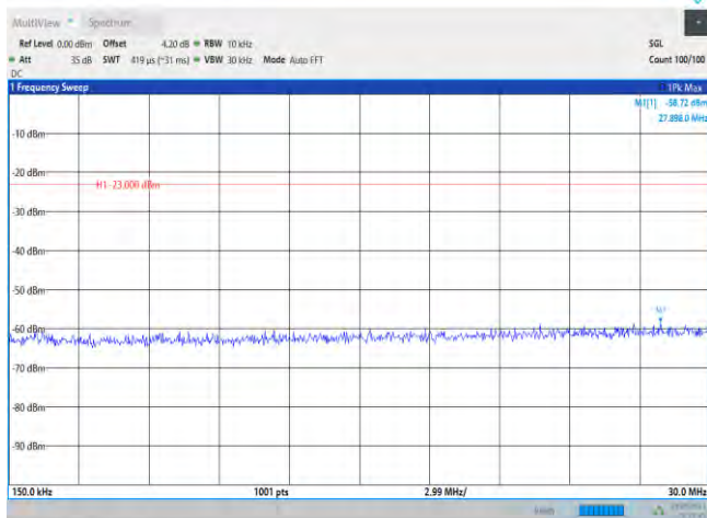
Band42-20MHz-QPSK-42190-1RB#0-Range2:0.15~30MHz
