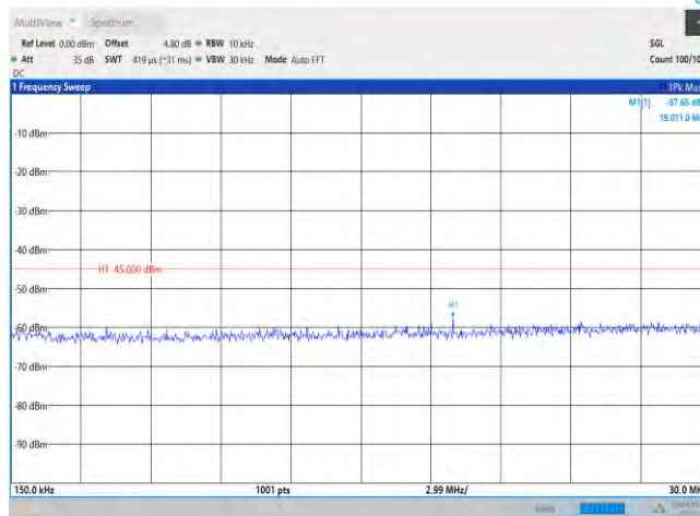
Band38-20MHz-QPSK-37850-1RB#0-Range2:0.15~30MHz
