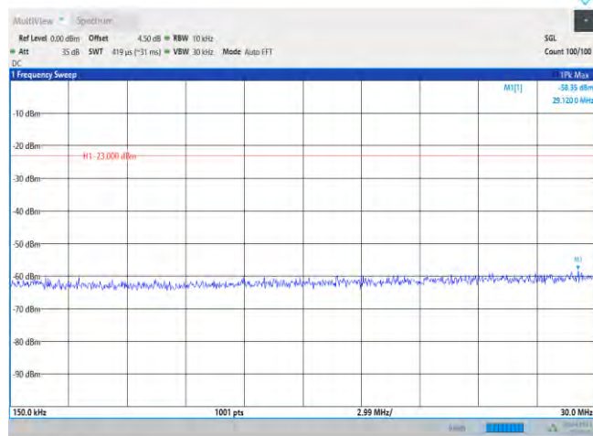
Band2-20MHz-QPSK-18700-1RB#0-Range2:0.15~30MHz
