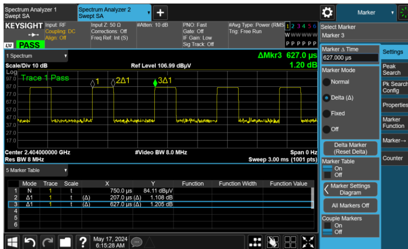
Bluetooth LE 2Mbps Ant. 9
