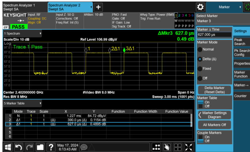
Bluetooth LE 1Mbps Ant. 9
