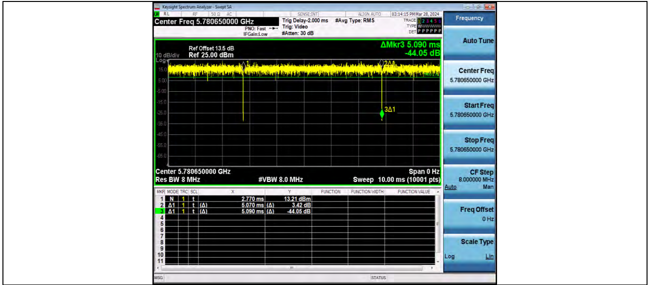
11AX20MIMO_Ant2_5785_106Tone_RU53
