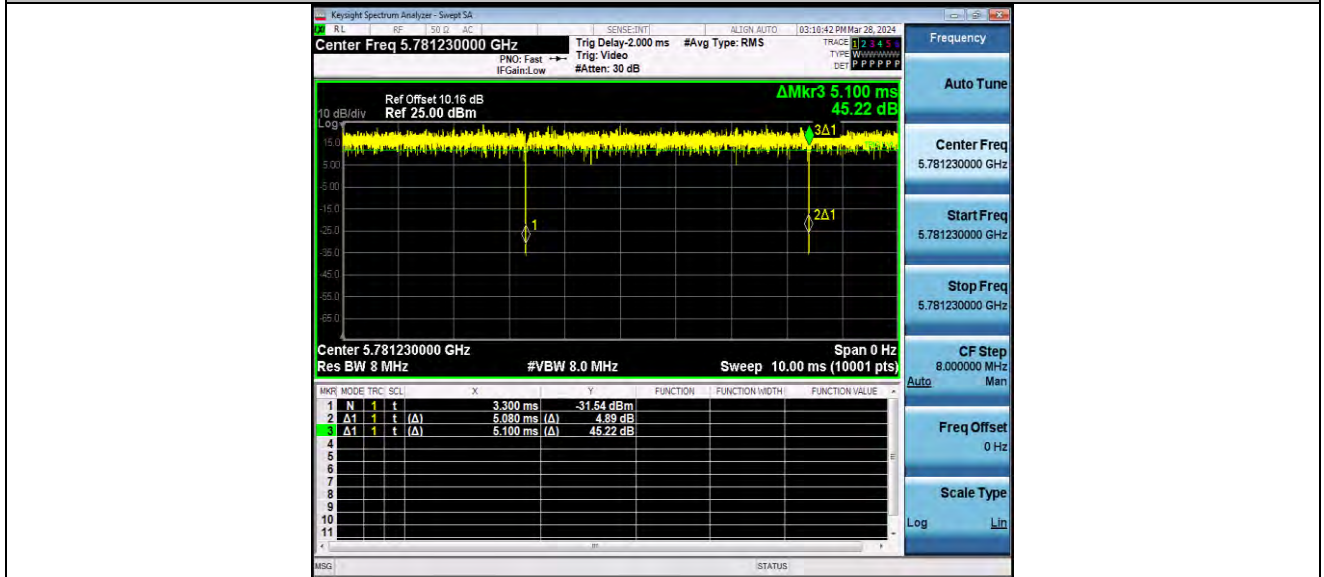
11AX20MIMO_Ant1_5785_106Tone_RU53
