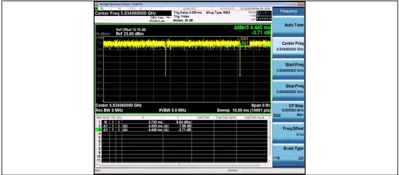
11AX20MIMO_Ant1_5825_52Tone_RU40
