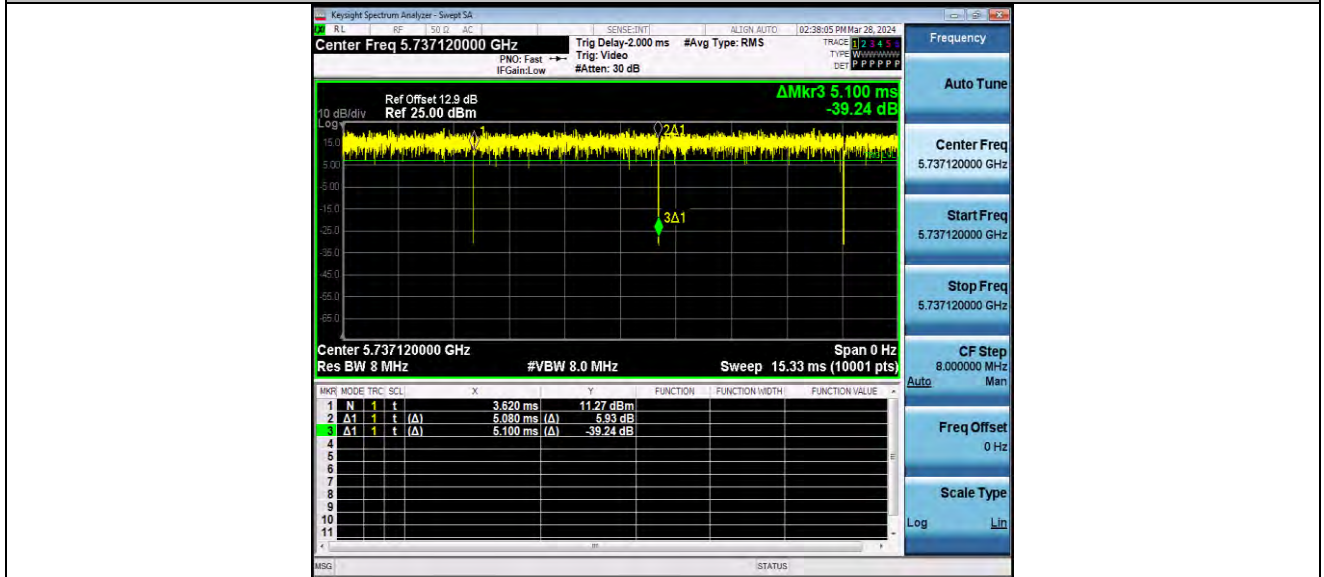
11AX20MIMO_Ant2_5745_52Tone_RU37
