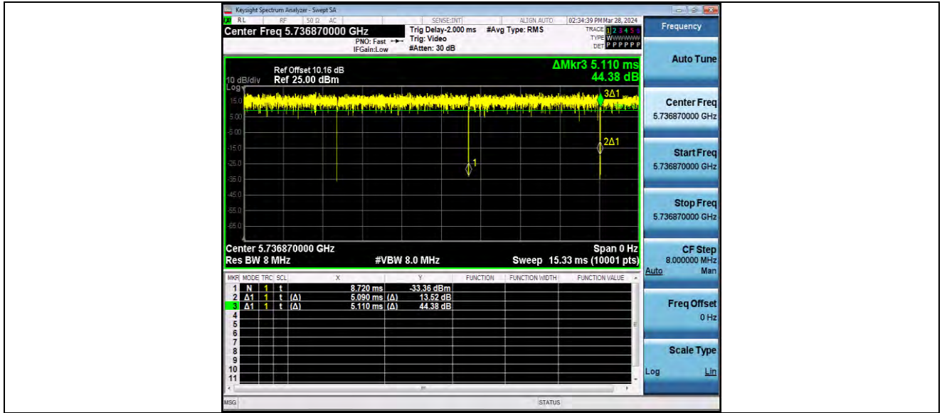
11AX20MIMO_Ant1_5745_52Tone_RU37
