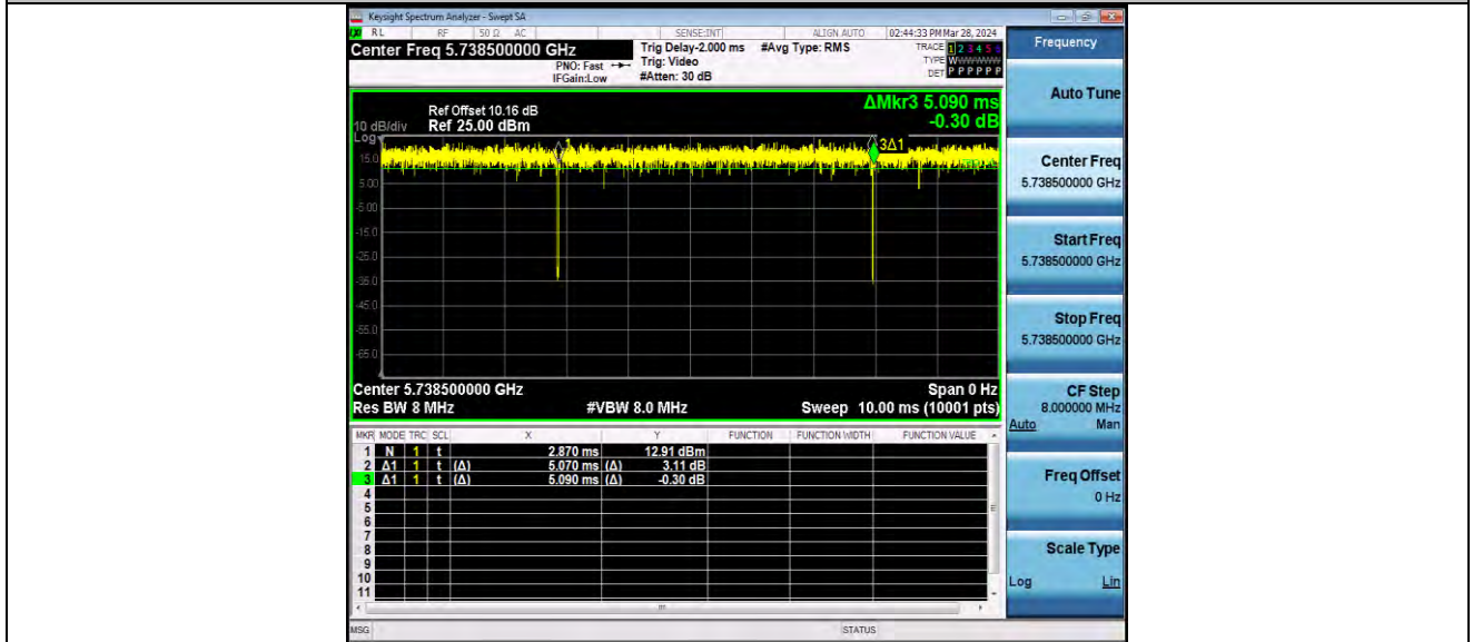
11AX20MIMO_Ant1_5745_106Tone_RU53
