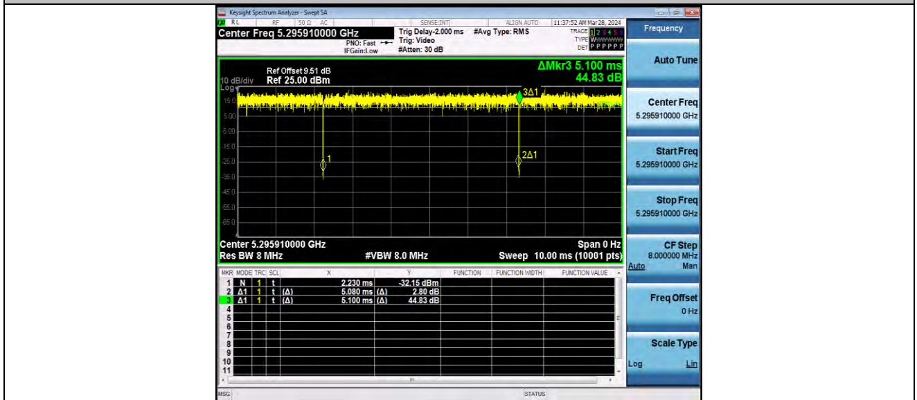
11AX20MIMO_Ant1_5300_106Tone_RU53
