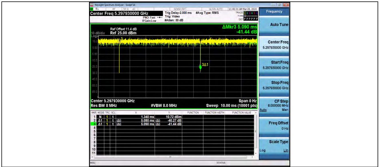
11AX20MIMO_Ant2_5300_106Tone_RU53
