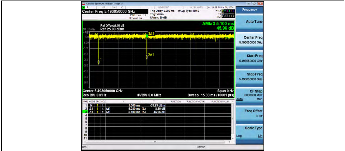
11AX20MIMO_Ant2_5500_26Tone_RU0
