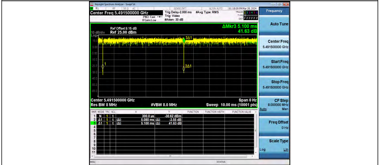
11AX20MIMO_Ant1_5500_106Tone_RU53
