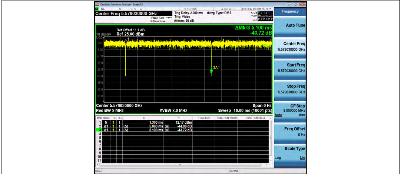
11AX20MIMO_Ant2_5580_52Tone_RU38
