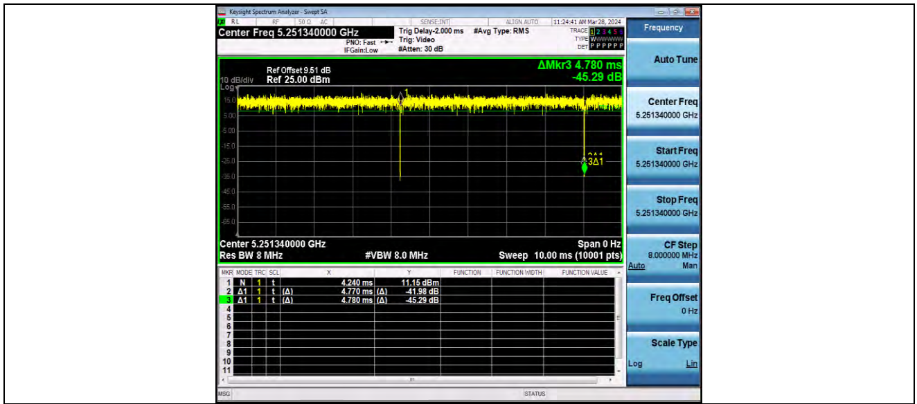
11AX20MIMO_Ant2_5260_26Tone_RU0
