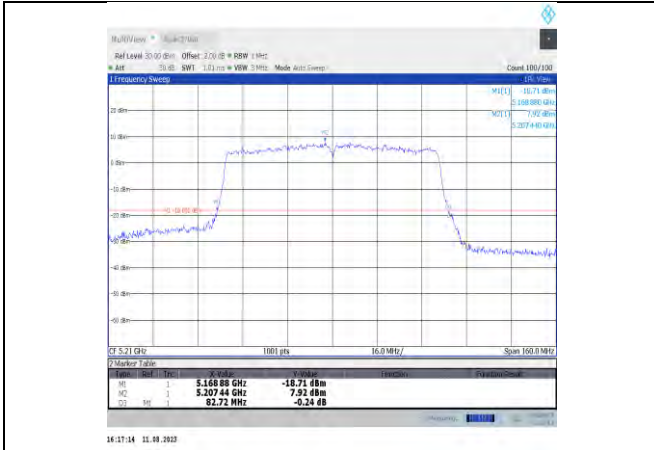
11ac80MIMO-Ant11-5210
