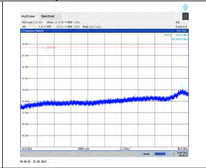
1-N78-3700-3800-PC2-30-100-L-1-N/A-DFT-PI2BPS K-Inner_1RB_Left-1@1-18000-40000-Ant1-18000.00 --58.31--13-PASS
