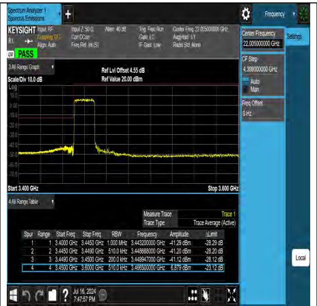
Band42 20MHz QPSK 42190 100RB#0
