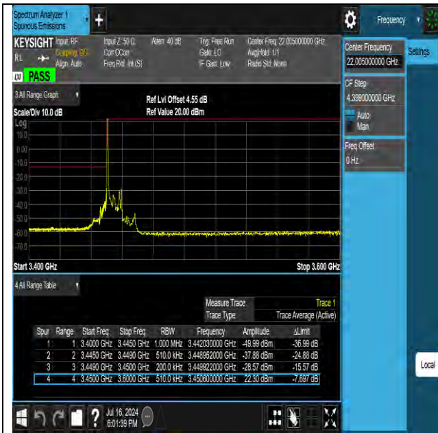
Band42 10MHz QPSK 42140 1RB#0
