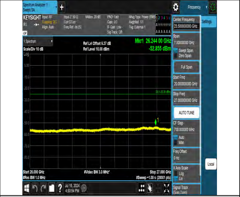
Band41 10MHz QPSK 41540 1RB#0 20000~27000 20000~27000
