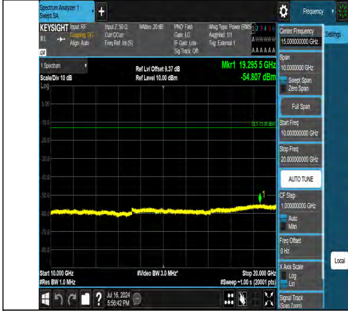
Band42 5MHz QPSK 42115 1RB#0 10000~20000 10000~20000
