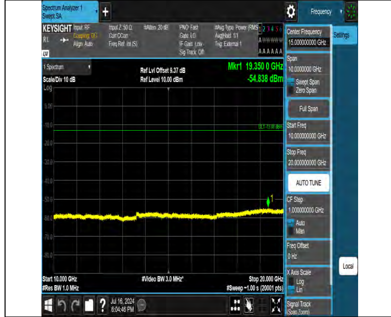
Band42 10MHz QPSK 42140 1RB#0 10000~20000 10000~20000
