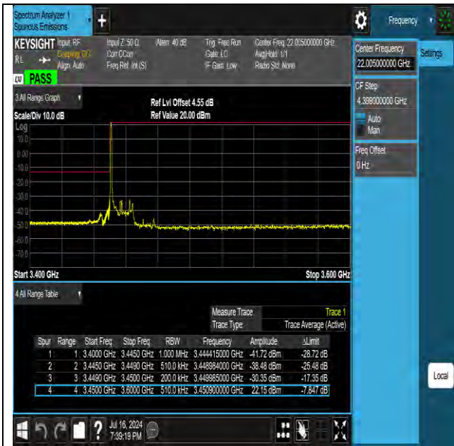
Band42 15MHz QPSK 42165 1RB#0
