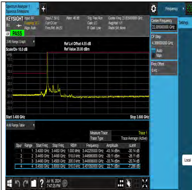
Band42 20MHz QPSK 42190 1RB#0
