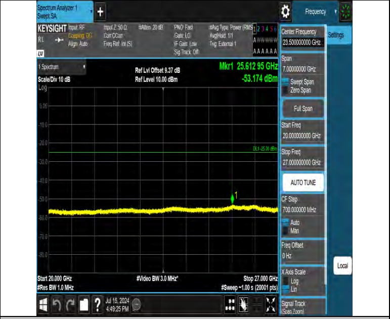
Band41 10MHz QPSK 40620 1RB#0 20000~27000 20000~27000
