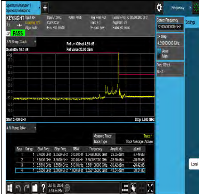
Band42 20MHz QPSK 42990 1RB#99
