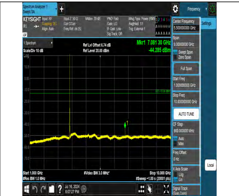
Band42 10MHz QPSK 43040 1RB#0 1000~10000 1000~10000
