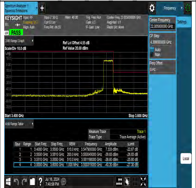
Band42 15MHz QPSK 43015 75RB#0
