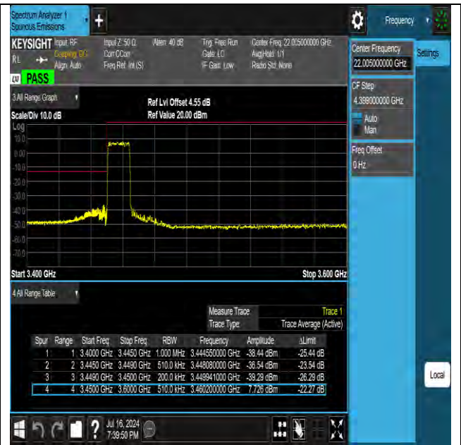
Band42 15MHz QPSK 42165 75RB#0
