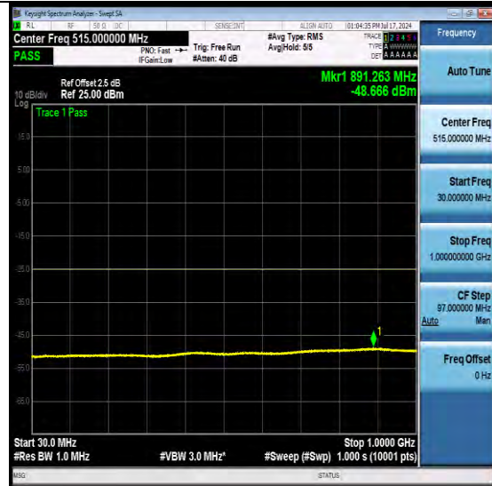
NTNV-N7-PC3-15-25-L-DFT-QPSK-Edge_1RB_L eft-Ant1-PASS
