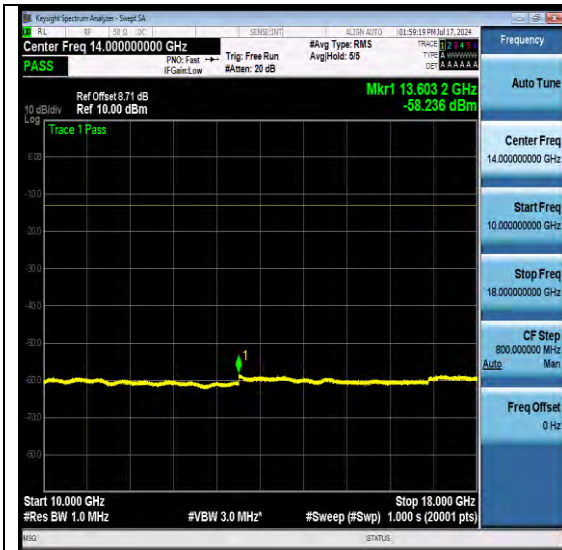
NTNV-N66-PC3-15-40-M-DFT-QPSK-Edge_1RB_Left-Ant1-PASS
