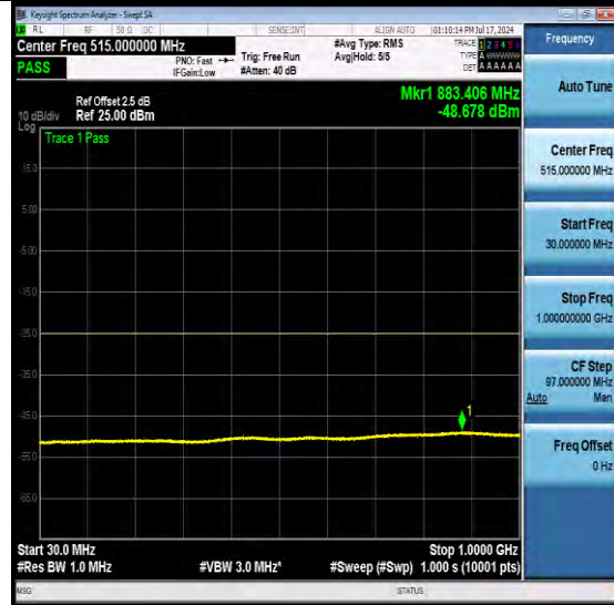
NTNV-N7-PC3-15-50-M-DFT-QPSK-Edge_1RB_L eft-Ant1-PASS
