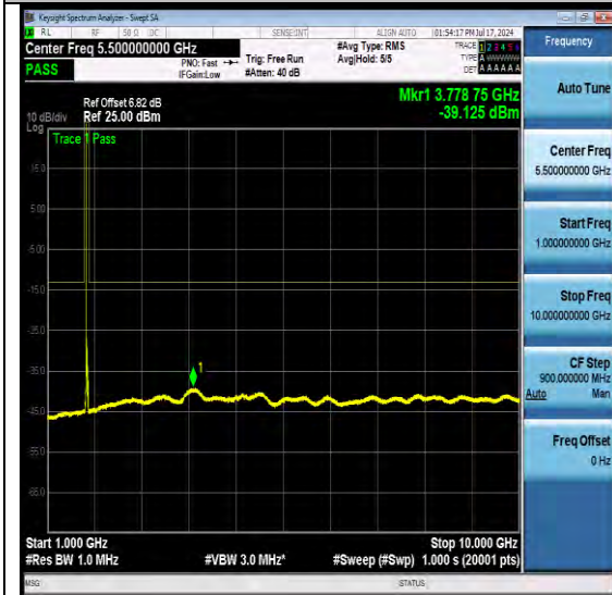
NTNV-N66-PC3-15-20-M-DFT-QPSK-Edge_1RB_Left-Ant1-PASS
