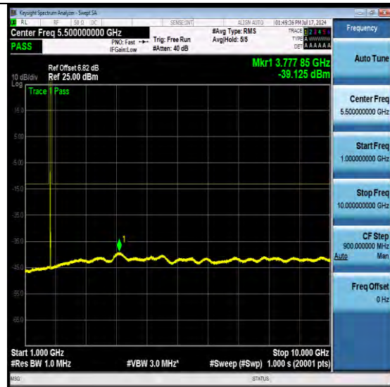
NTNV-N66-PC3-15-5-M-DFT-QPSK-Edge_1RB_L eft-Ant1-PASS
