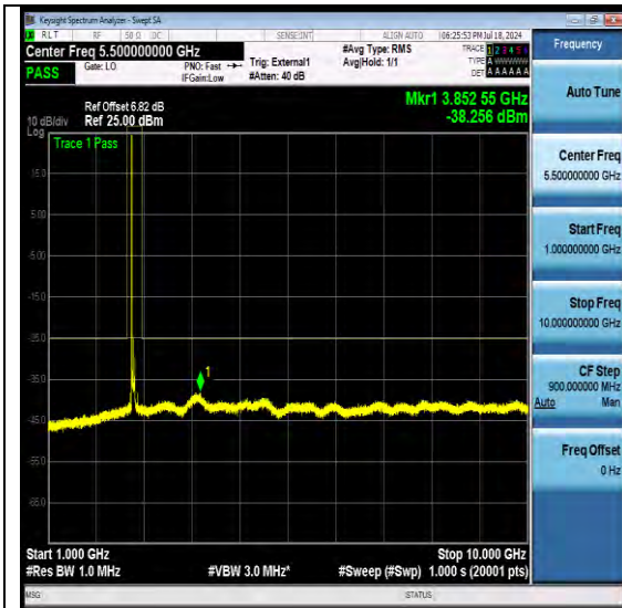
NTNV-N41-PC3-30-60-M-DFT-QPSK-Edge_1RB_Left-Ant1-PASS
