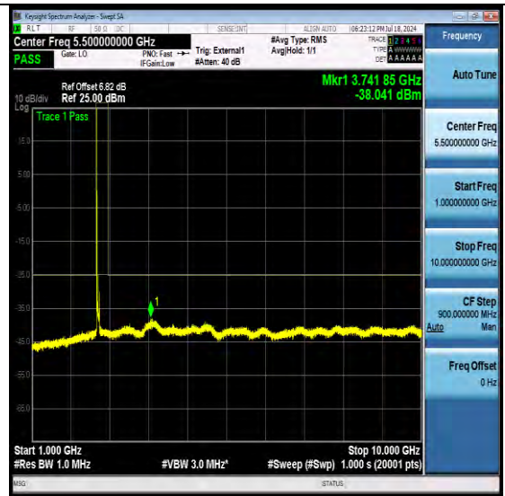
NTNV-N41-PC3-30-60-L-DFT-QPSK-Edge_1RB_Left-Ant1-PASS
