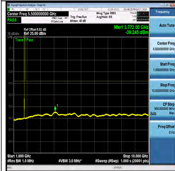
NTNV-N66-PC3-15-5-L-DFT-QPSK-Edge_1RB_L eft-Ant1-PASS
