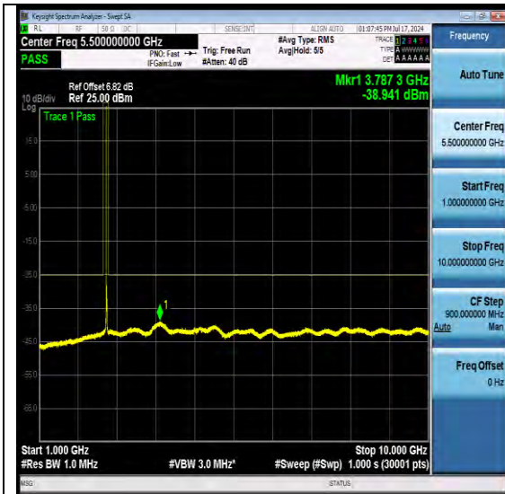
NTNV-N7-PC3-15-25-H-DFT-QPSK-Edge_1RB_L eft-Ant1-PASS
