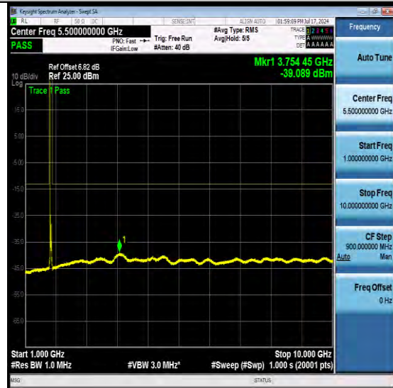
NTNV-N66-PC3-15-40-M-DFT-QPSK-Edge_1RB_Left-Ant1-PASS
