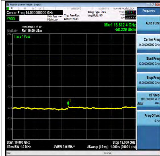
NTNV-N66-PC3-15-5-M-DFT-QPSK-Edge_1RB_L eft-Ant1-PASS
