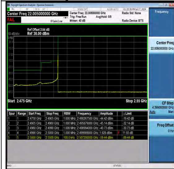
NTNV-N7-PC3-15-50-L-DFT-QPSK-Edge_1RB_L eft-Ant1-FAIL
