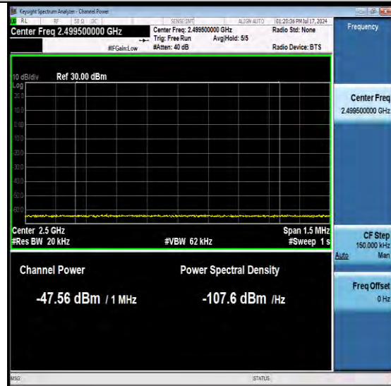
NTNV-N7-PC3-15-50-L-DFT-QPSK-Edge_1RB_L eft-Ant1-PASS
