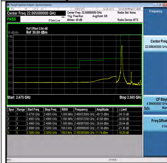
NTNV-N7-PC3-15-5-L-DFT-QPSK-Edge_1RB_Lef t-Ant1-PASS
