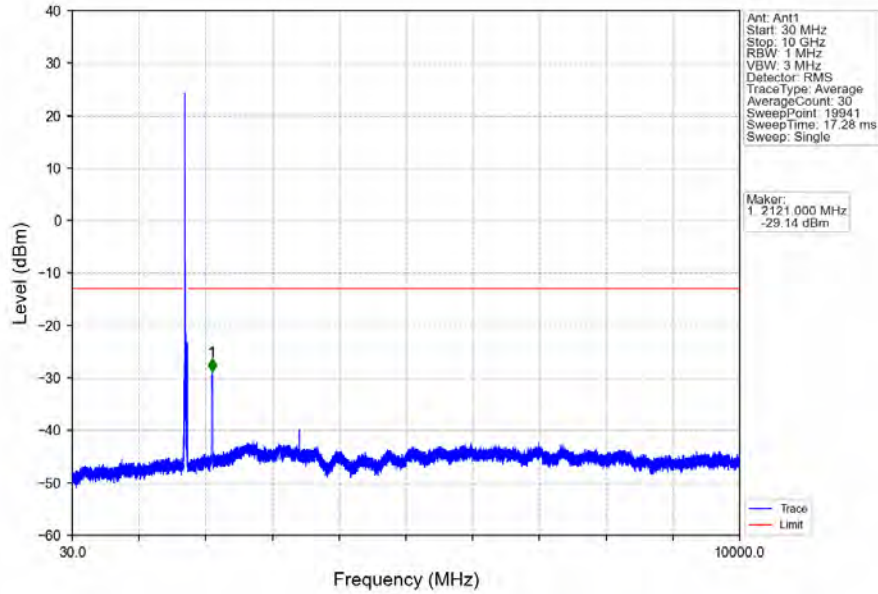
Band66_20MHz_QPSK_LCH_1720MHz_RB_1_0_NTNV
