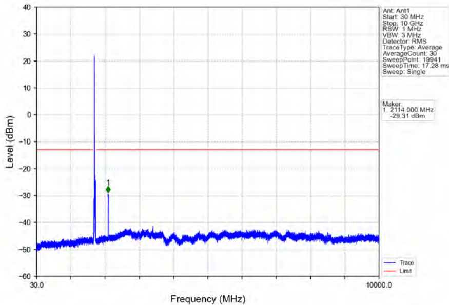
Band66_20MHz_16QAM_LCH_1720MHz_RB_1_0_NTNV
