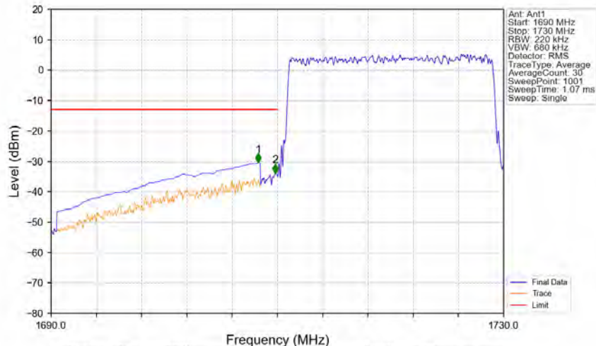
Band66_20MHz_16QAM_LCH_1720MHz_RB_100_0_NTNV
