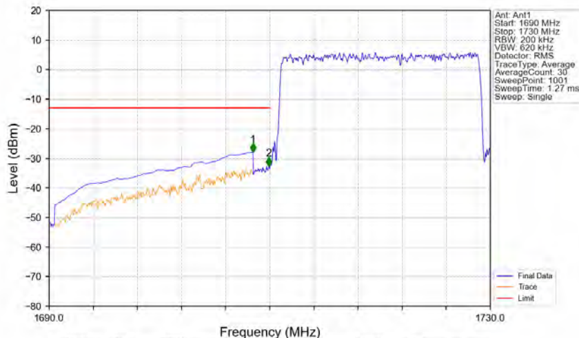
Band66_20MHz_QPSK_LCH_1720MHz_RB_100_0_NTNV
