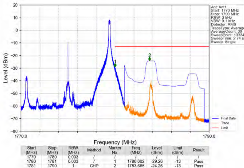
Band66_10MHz_QPSK_HCH_1775MHz_RB_1_49_NTNV
