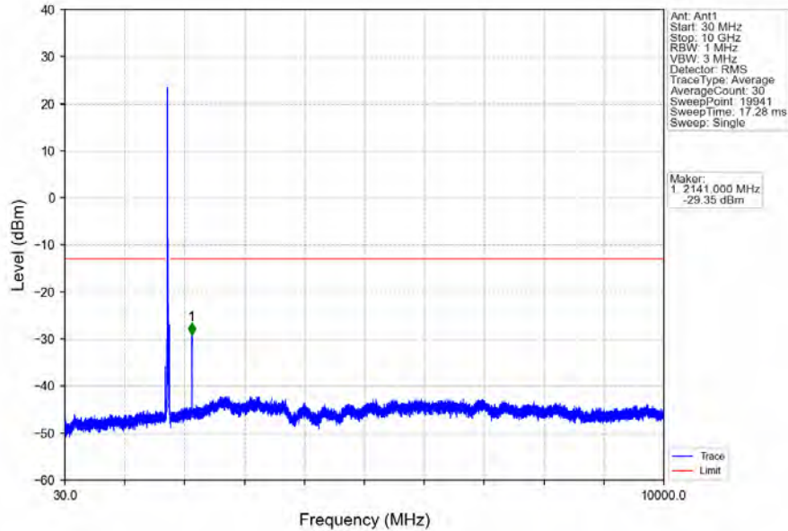
Band66_20MHz_QPSK_MCH_1745MHz_RB_1_0_NTNV
