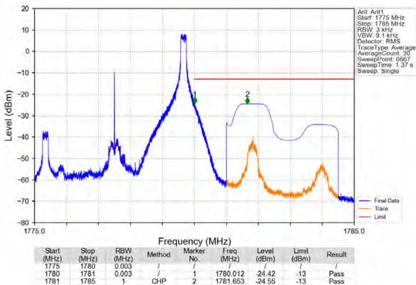
Band66_5MHz_QPSK_HCH_1777.5MHz_RB_1_24_NTNV
