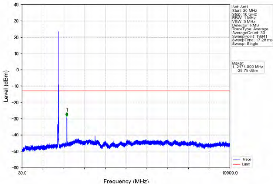
Band66_20MHz_QPSK_HCH_1770MHz_RB_1_0_NTNV
