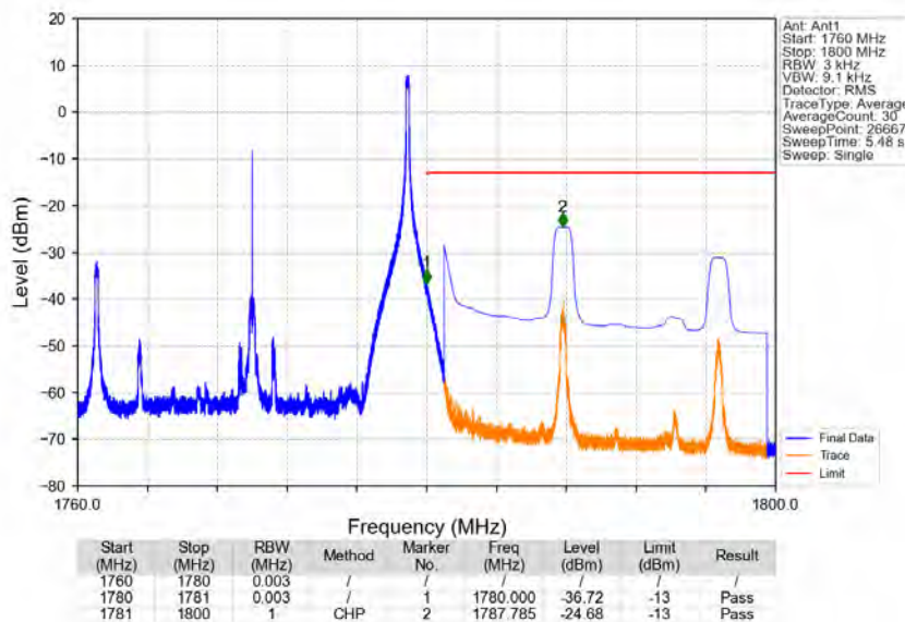
Band66_20MHz_QPSK_HCH_1770MHz_RB_1_99_NTNV
