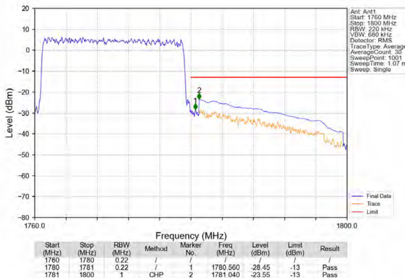
Band66_20MHz_QPSK_HCH_1770MHz_RB_100_0_NTNV
