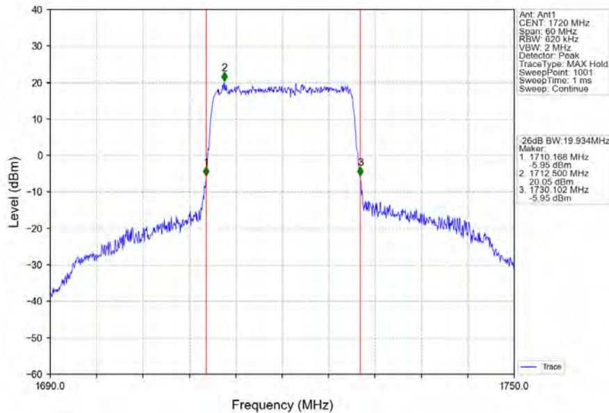
Band66_20MHz_QPSK_LCH_1720MHz_RB_100_0_NTNV
