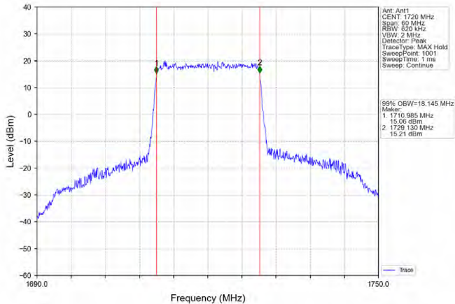
Band66_20MHz_QPSK_LCH_1720MHz_RB_100_0_NTNV
