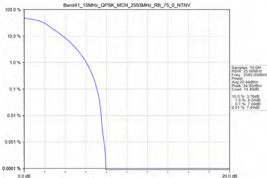
Band41_15MHz QPSK MCH_2593MHz_RB_75_0_NTNV
