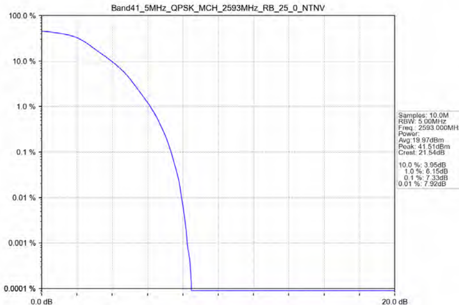
Band41_5MHz_QPSK_MCH_2593MHz_RB_25_0_NTNV
