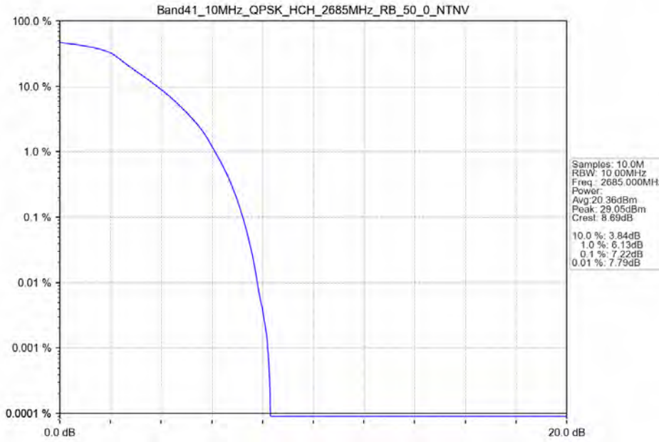
Band41_10MHz QPSK HCH_2685MHz_RB_50_0_NTNV
