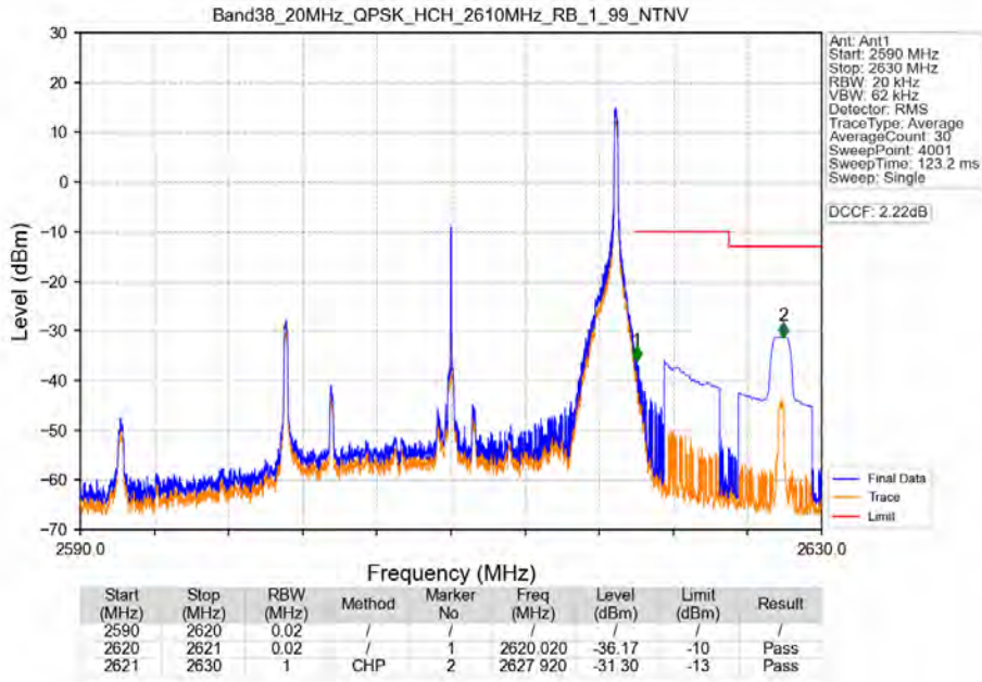
Band38_20MHz_QPSK_HCH_2610MHz_RB_1_99_NTNV
