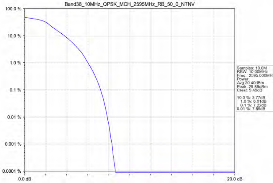
Band38_10MHz QPSK MCH_2595MHz_RB_50_0_NTNV
