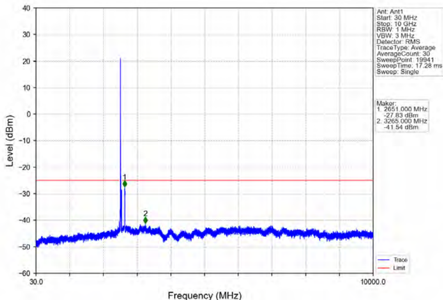
Band7_20MHz_64QAM_MCH_2535MHz_RB_1_0_NTNV
