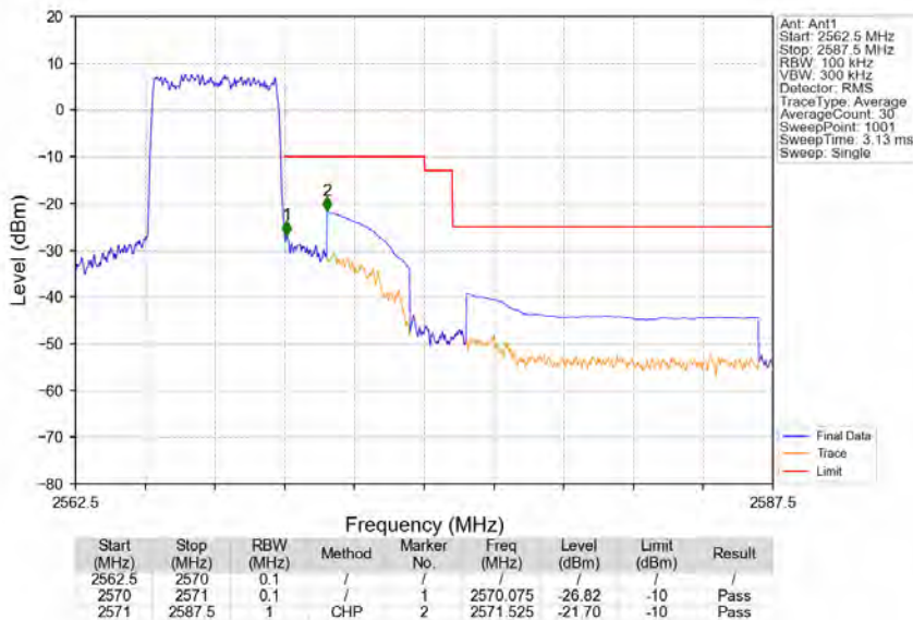
Band7_5MHz_QPSK_HCH_2567.5MHz_RB_25_0_NTNV
