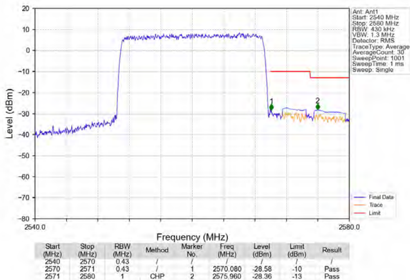
Band7_20MHz_QPSK_HCH_2560MHz_RB_100_0_NTNV
