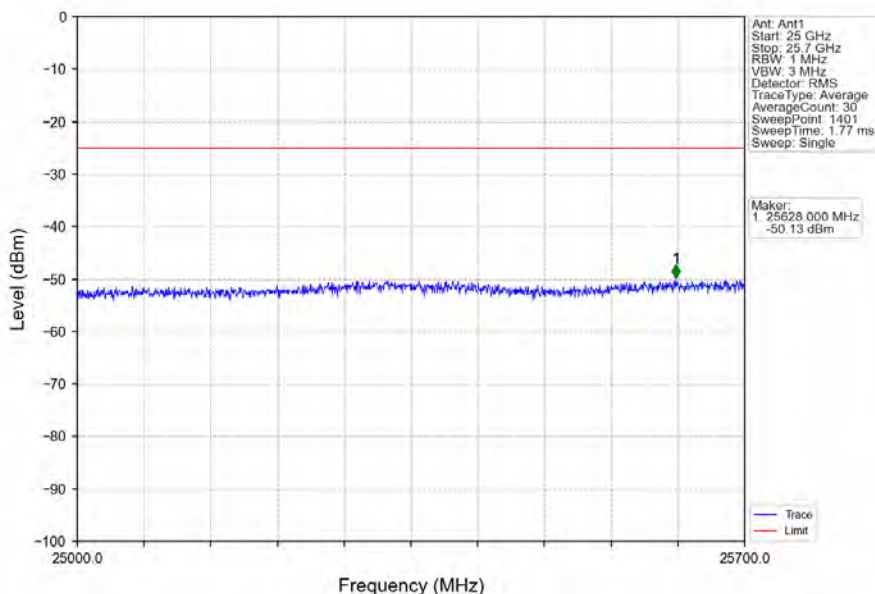
Band7_20MHz_64QAM_HCH_2560MHz_RB_1_99_NTNV
