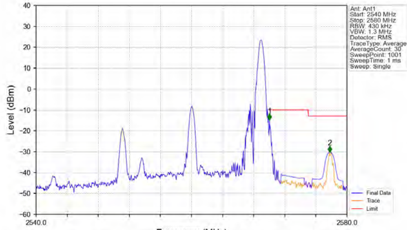
Band7_20MHz_QPSK_HCH_2560MHz_RB_1_99_NTNV
