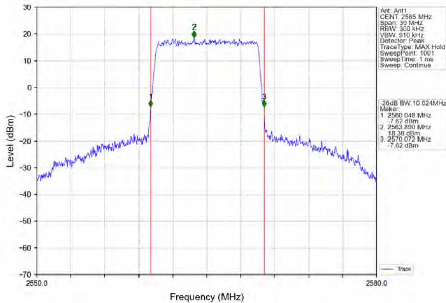
Band7_10MHz_QPSK_HCH_2565MHz_RB_50_0_NTNV
