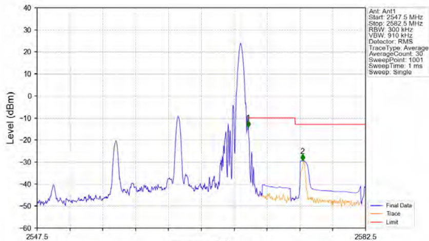
Band7_15MHz_QPSK_HCH_2562.5MHz_RB_1_74_NTNV
