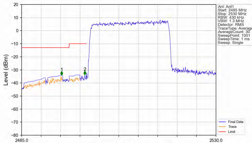
Band7_20MHz_16QAM_LCH_2510MHz_RB_100_0_NTNV
