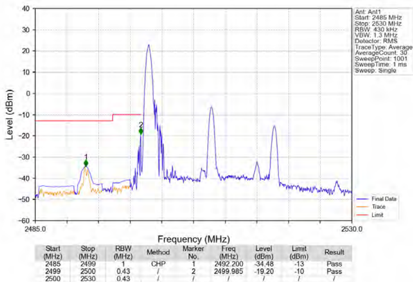
Band7_20MHz_16QAM_LCH_2510MHz_RB_1_0_NTNV
