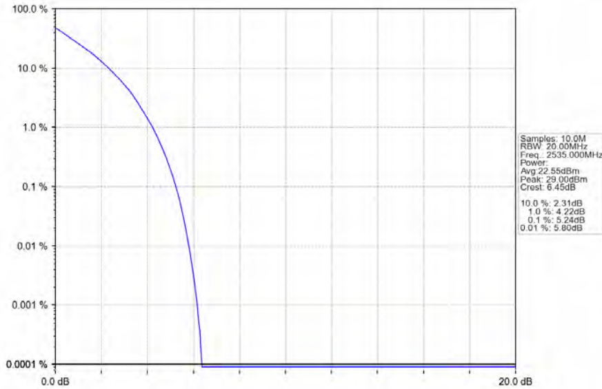
Band7_20MHz_QPSK_MCH_2535MHz_RB_100_0_NTNV
