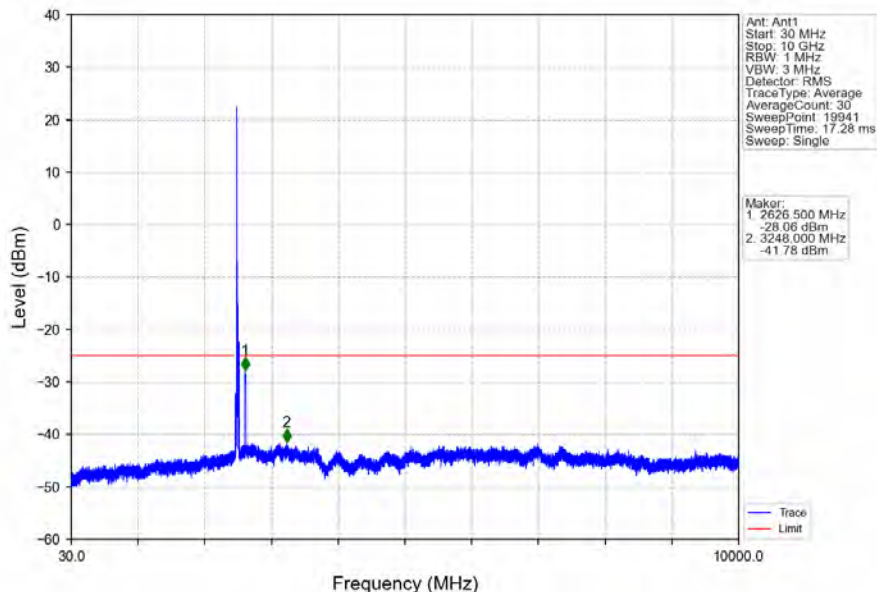
Band7_20MHz_QPSK_LCH_2510MHz_RB_1_0_NTNV
