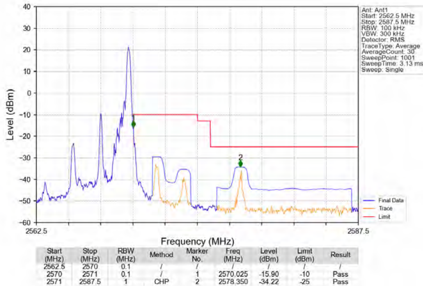
Band7_5MHz_QPSK_HCH_2567.5MHz_RB_1_24_NTNV
