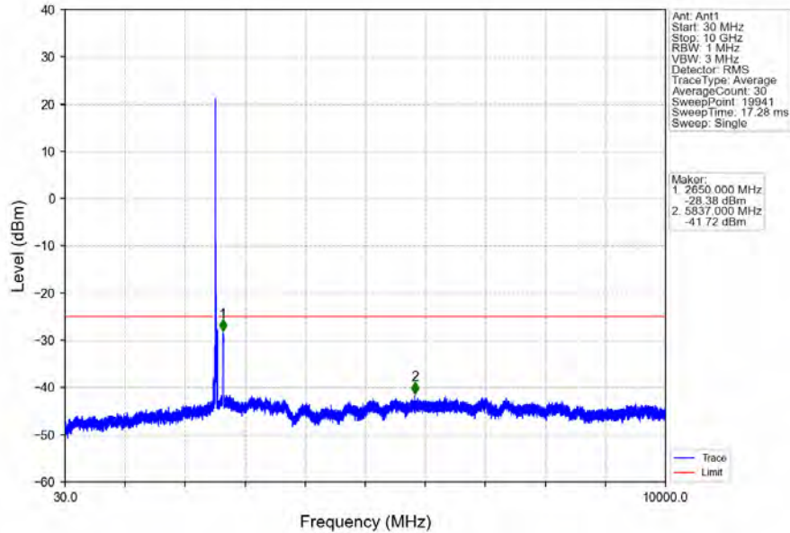
Band7_20MHz_16QAM_MCH_2535MHz_RB_1_0_NTNV
