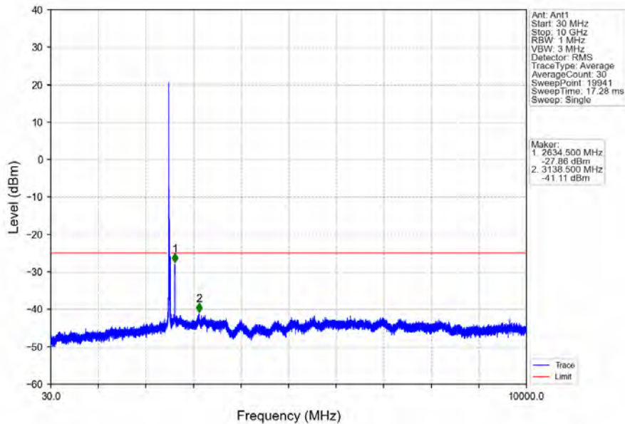
Band7_20MHz_64QAM_LCH_2510MHz_RB_1_0_NTNV
