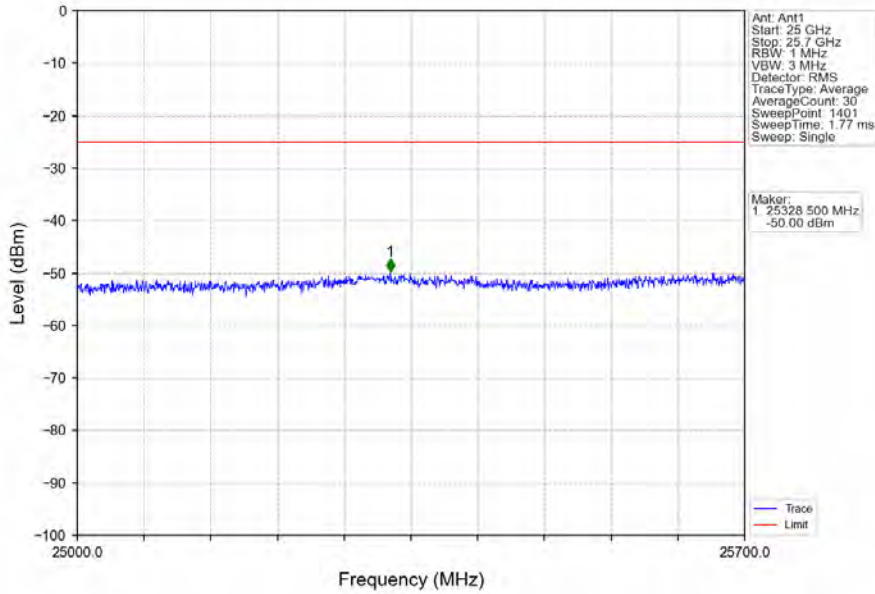
Band7_20MHz_QPSK_HCH_2560MHz_RB_1_99_NTNV
