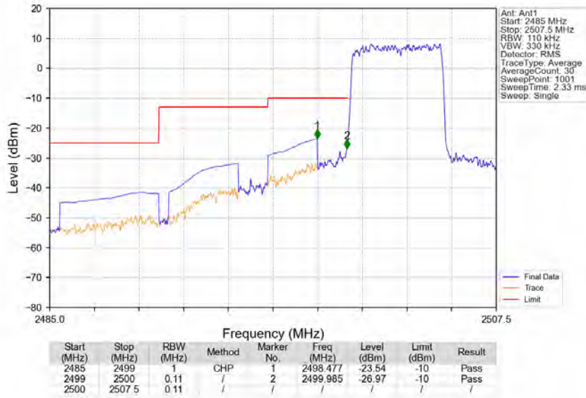
Band7_5MHz_QPSK_LCH_2502.5MHz_RB_25_0_NTNV
