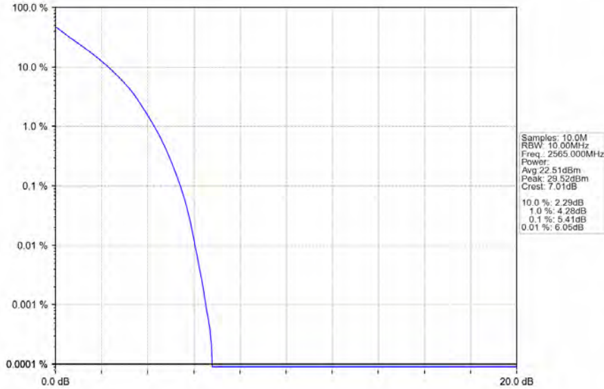
Band7_10MHz_QPSK_HCH_2565MHz_RB_50_0_NTNV
