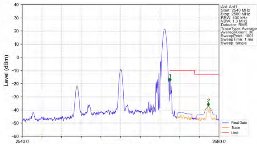
Band7_20MHz_64QAM_HCH_2560MHz_RB_1_99_NTNV
