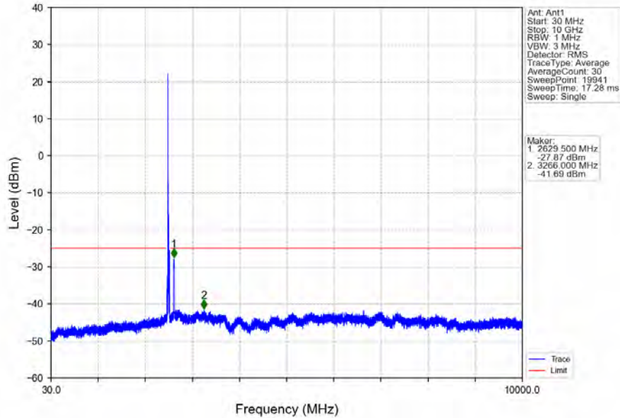
Band7_20MHz_16QAM_LCH_2510MHz_RB_1_0_NTNV
