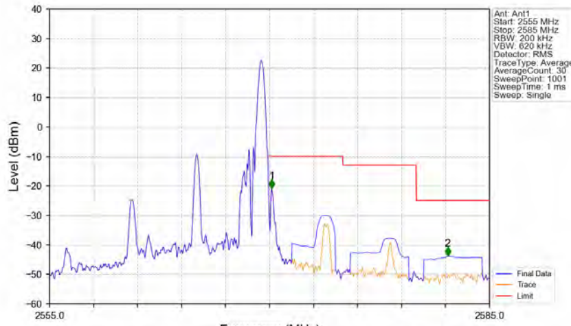
Band7_10MHz_QPSK_HCH_2565MHz_RB_1_49_NTNV
