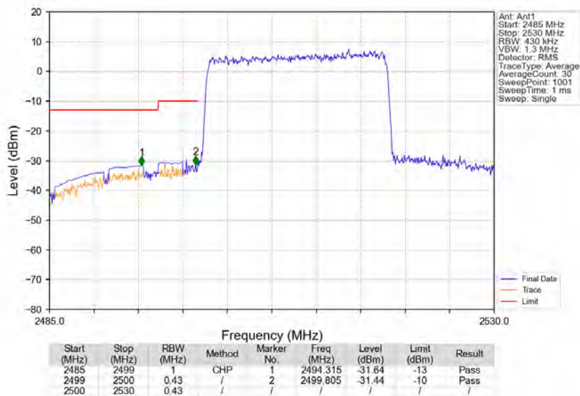
Band7_20MHz_64QAM_LCH_2510MHz_RB_100_0_NTNV
