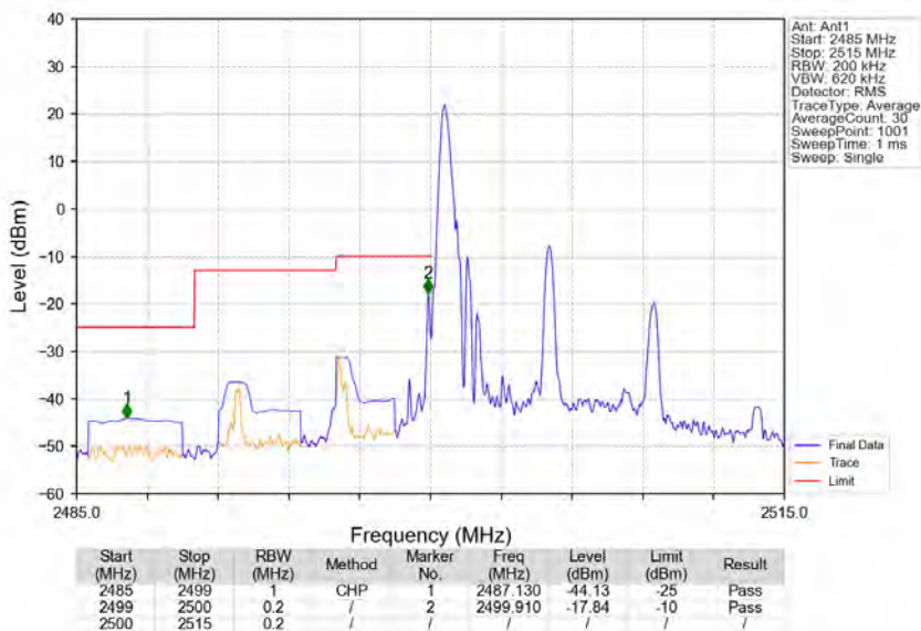
Band7_10MHz_16QAM_LCH_2505MHz_RB_1_0 NTN
