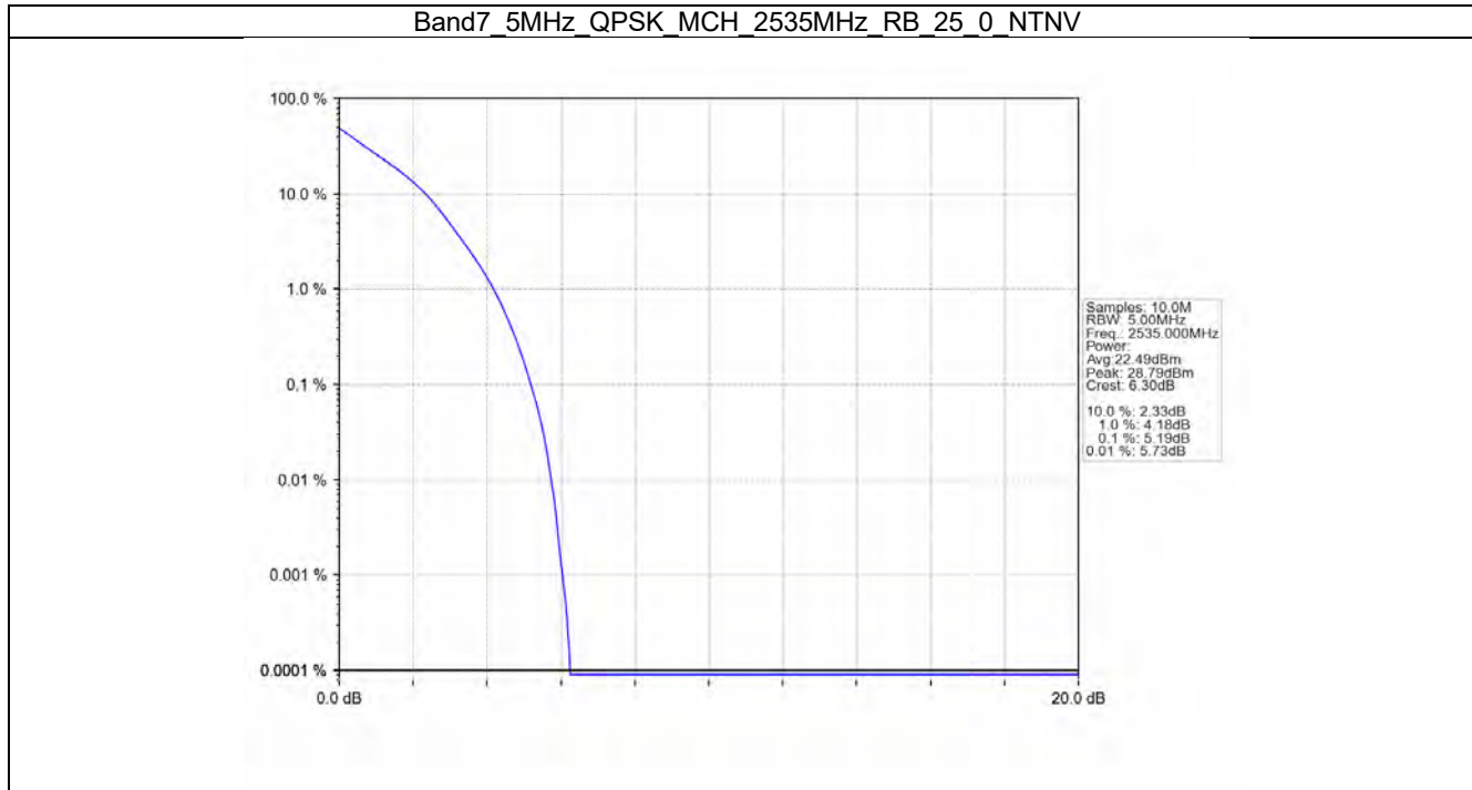
Band7_5MHz_QPSK_MCH_2535MHz_RB_25_0_NTNV
