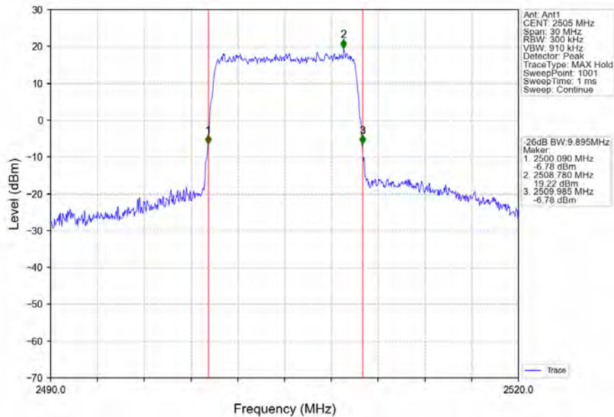
Band7_10MHz_QPSK_LCH_2505MHz_RB_50_0_NTNV
