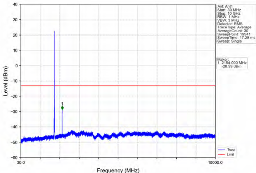
Band4_10MHz_QPSK_HCH_1750MHz_RB_1_0_NTNV
