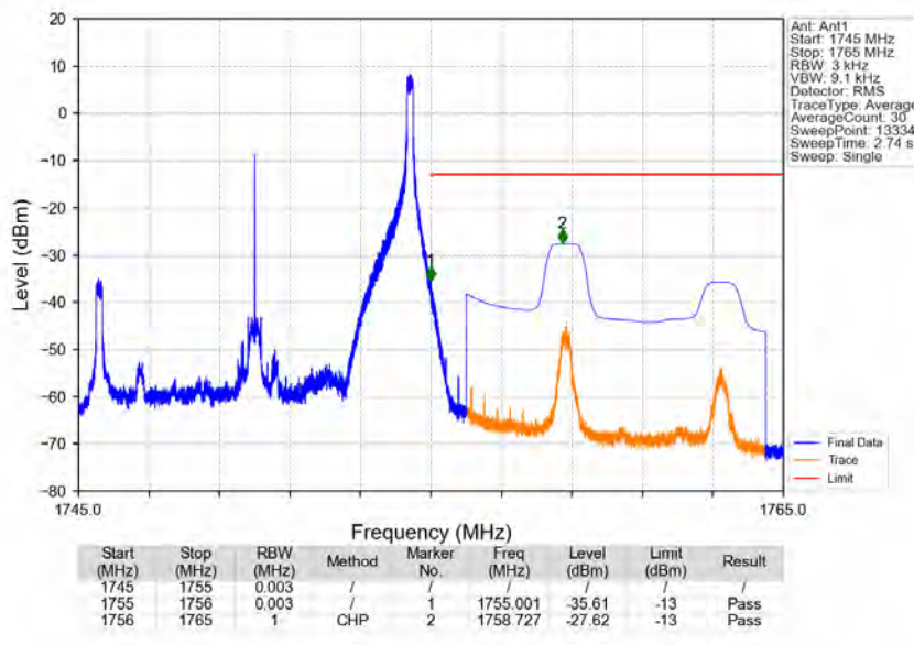
Band4_10MHz_QPSK_HCH_1750MHz_RB_50_0_NTNV
