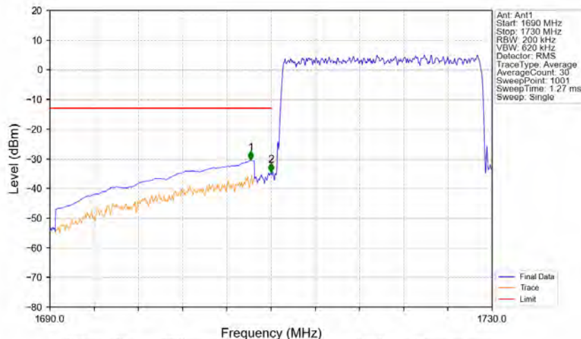
Band4_20MHz_16QAM_LCH_1720MHz_RB_100_0_NTNV
