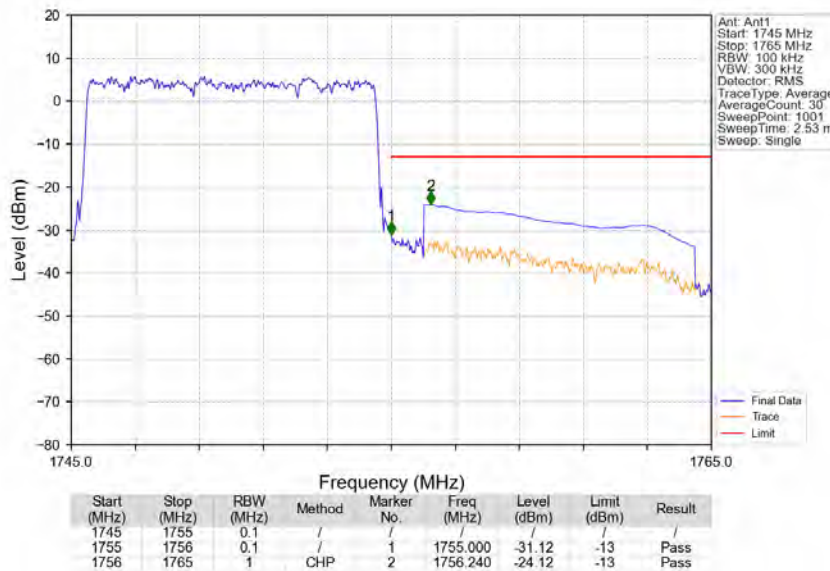
Band4_10MHz_QPSK_HCH_1750MHz_RB_50_0_NTNV
