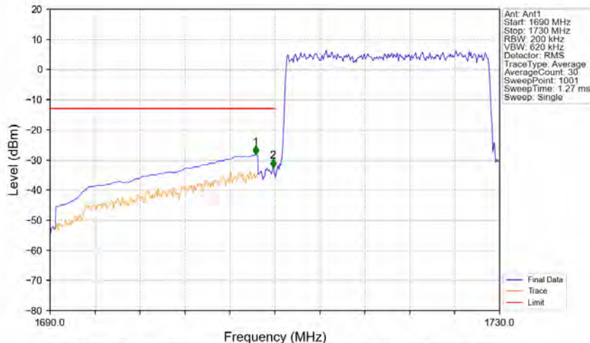
Band4_20MHz_QPSK_LCH_1720MHz_RB_100_0_NTNV
