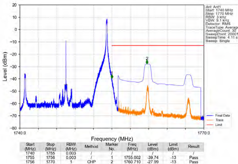
Band4_15MHz_QPSK_HCH_1747.5MHz_RB_1_74_NTNV
