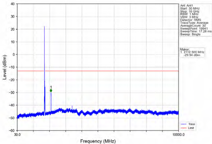
Band4_20MHz_16QAM_LCH_1720MHz_RB_1_0_NTNV
