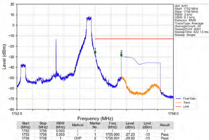
Band4_3MHz_QPSK_HCH_1753.5MHz_RB_1_14_NTNV
