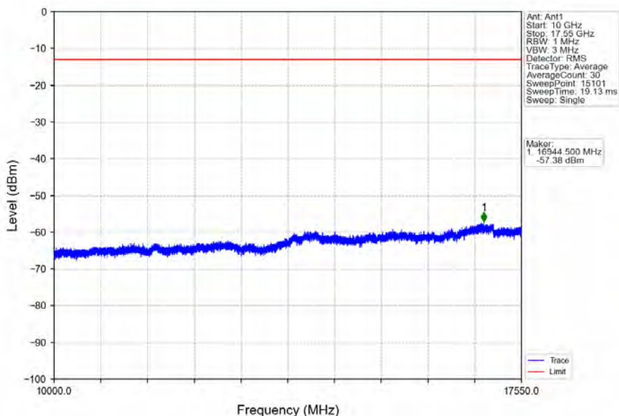
Band4_20MHz_16QAM_LCH_1720MHz_RB_100_0_NTNV
