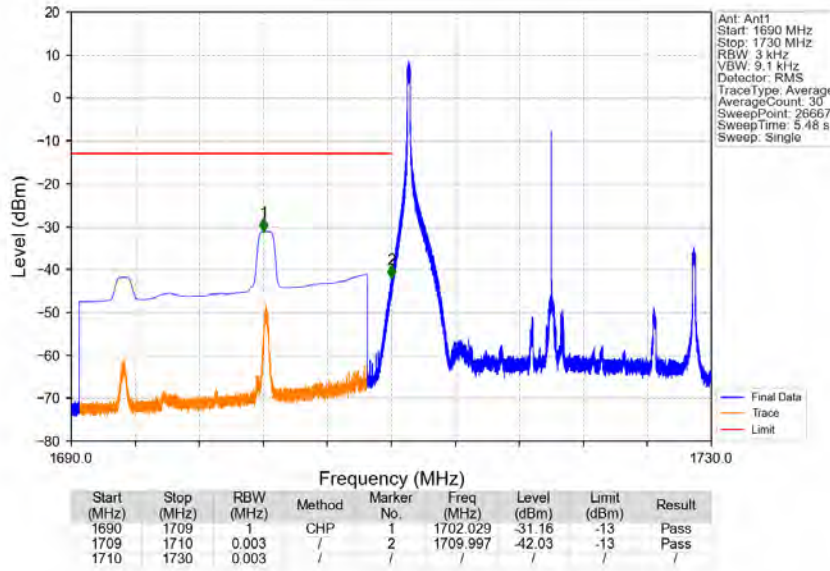
Band4_20MHz_16QAM_LCH_1720MHz_RB_1_0_NTNV
