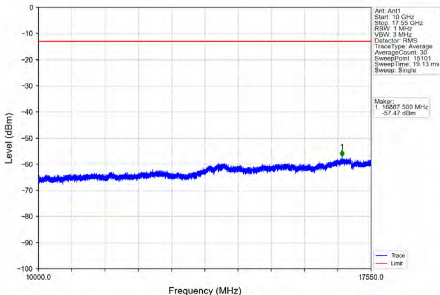
Band4_20MHz_QPSK_LCH_1720MHz_RB_100_0_NTNV
