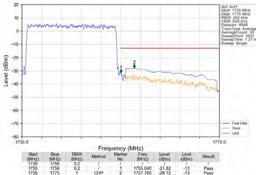
Band4_20MHz_QPSK_HCH_1745MHz_RB_100_0_NTNV
