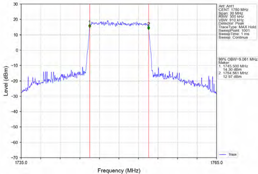
Band4_10MHz_QPSK_HCH_1750MHz_RB_50_0_NTNV
