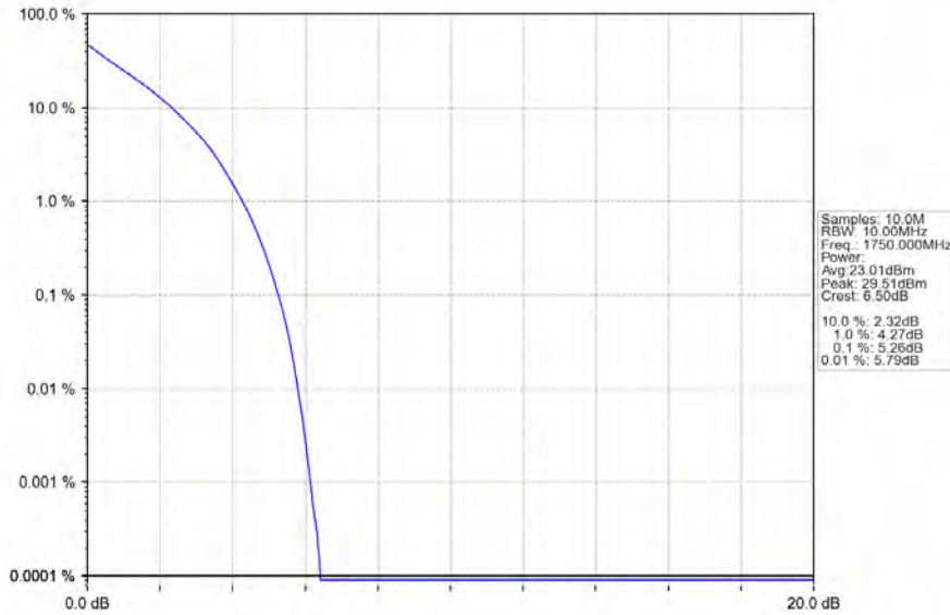
Band4_10MHz_QPSK_HCH_1750MHz_RB_50_0_NTNV
