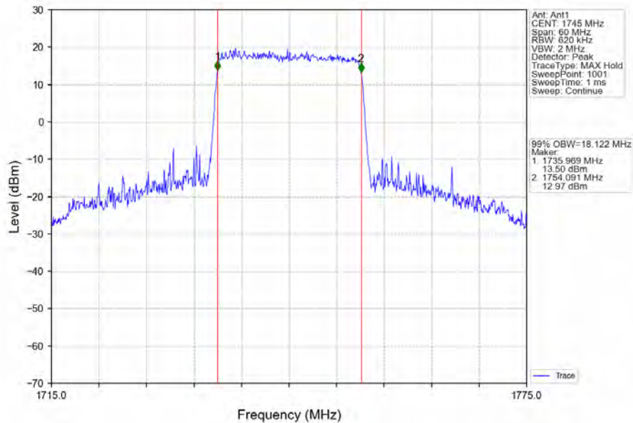
Band4_20MHz_QPSK_HCH_1745MHz_RB_100_0_NTNV
