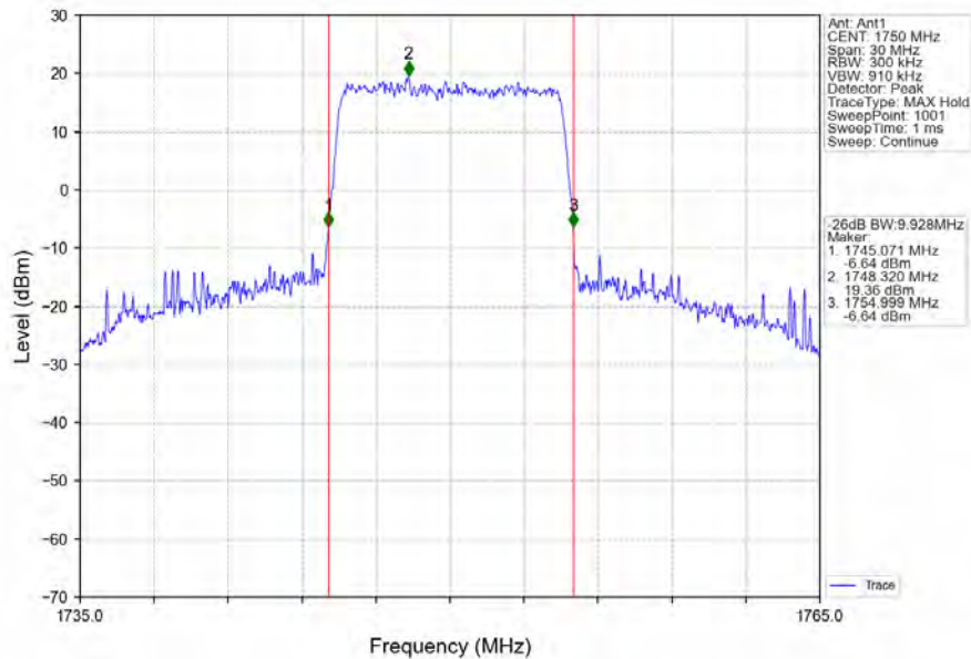
Band4_10MHz_QPSK_HCH_1750MHz_RB_50_0_NTNV
