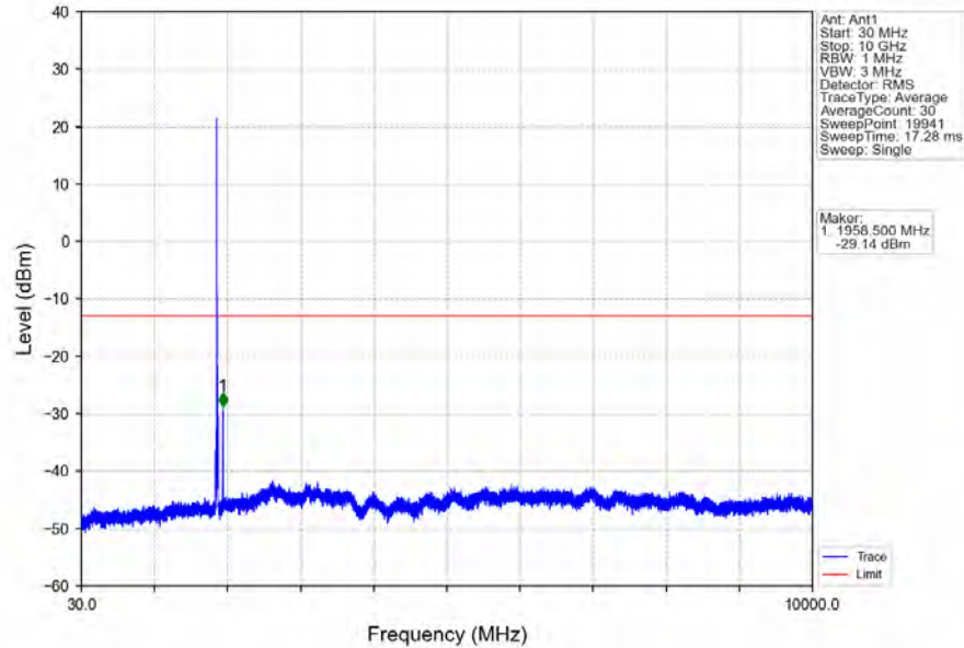
Band2_10MHz_16QAM_MCH_1880MHz_RB_1_0_NTNV
