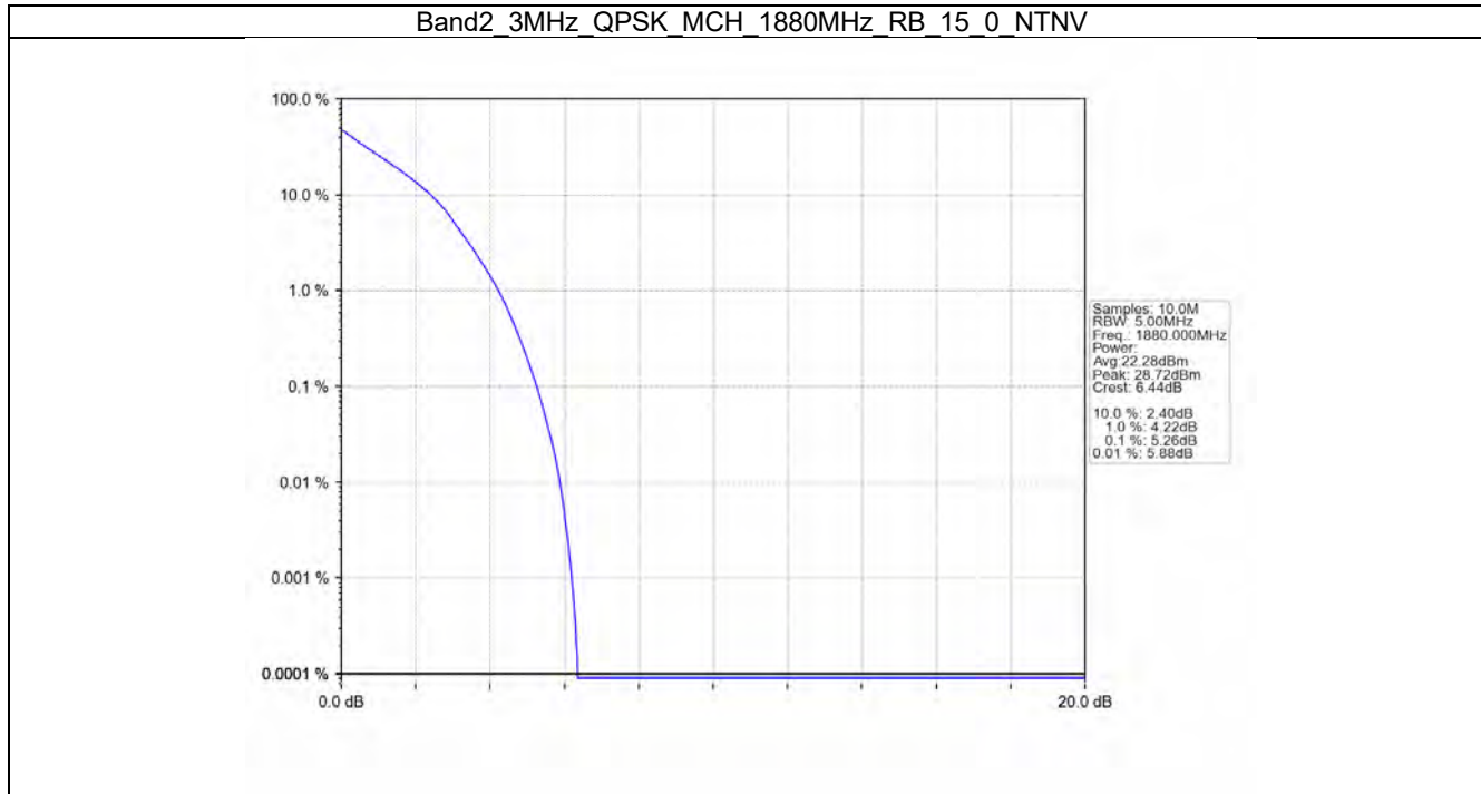
Band2_3MHz_QPSK_MCH_1880MHz_RB_15_0_NTNV
