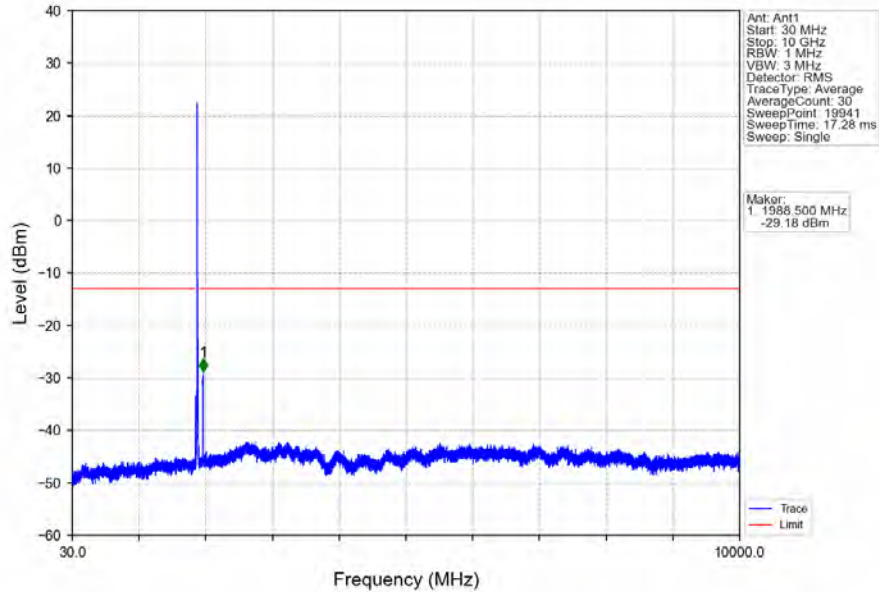
Band2_15MHz_QPSK_HCH_1902.5MHz_RB_1_0_NTNV
