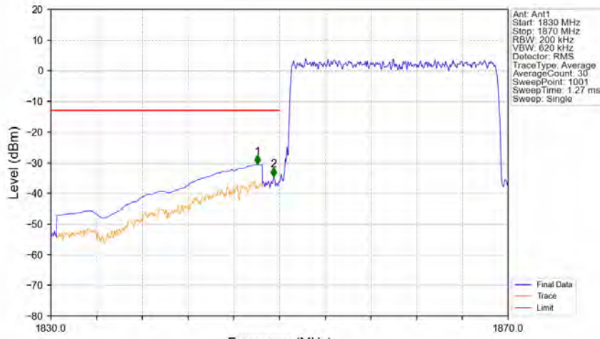
Band2_20MHz_16QAM_LCH_1860MHz_RB_100_0_NTNV
