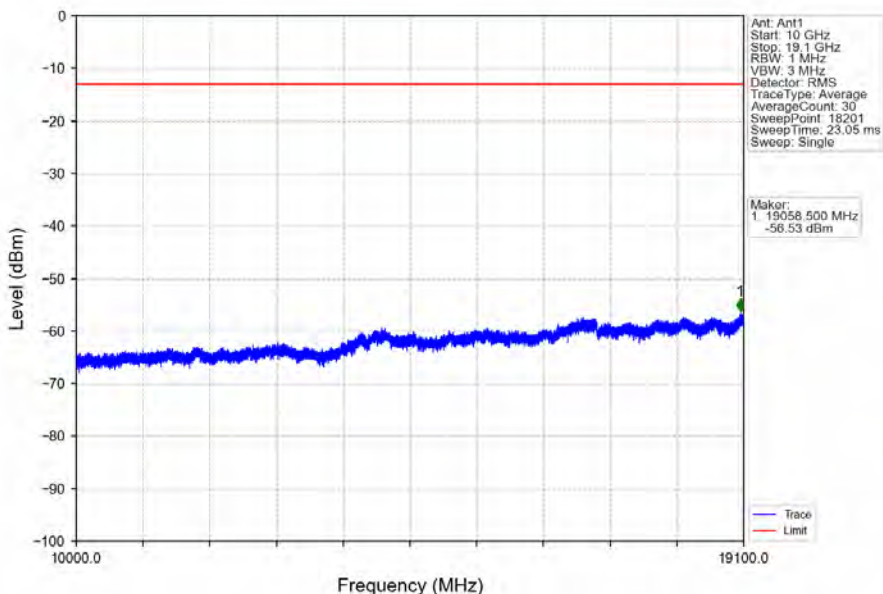
Band2_20MHz_64QAM_MCH_1880MHz_RB_1_0_NTNV
