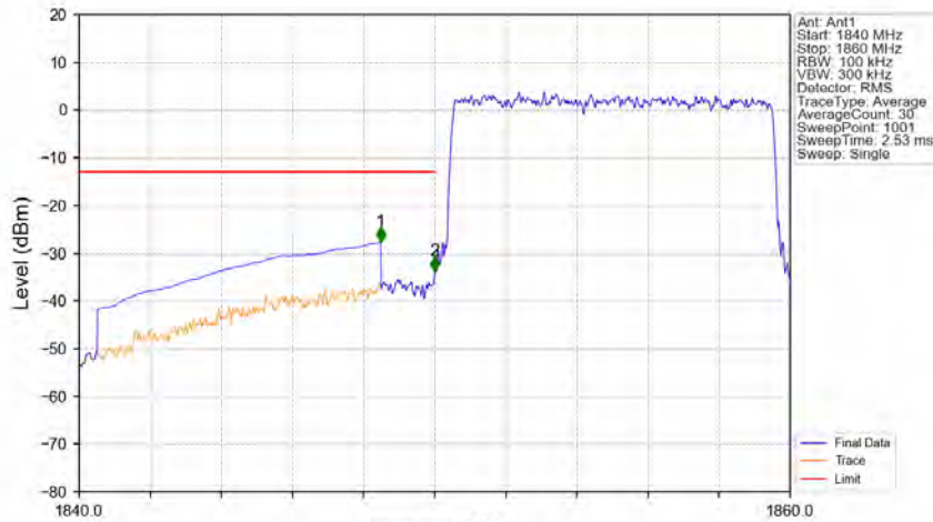
Band2_10MHz_16QAM_LCH_1855MHz_RB_50_0_NTNV
