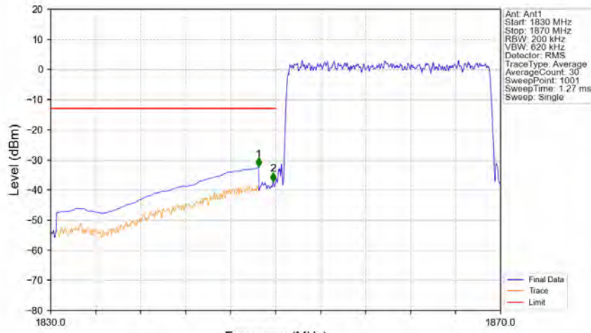
Band2_20MHz_64QAM_LCH_1860MHz_RB_100_0_NTNV
