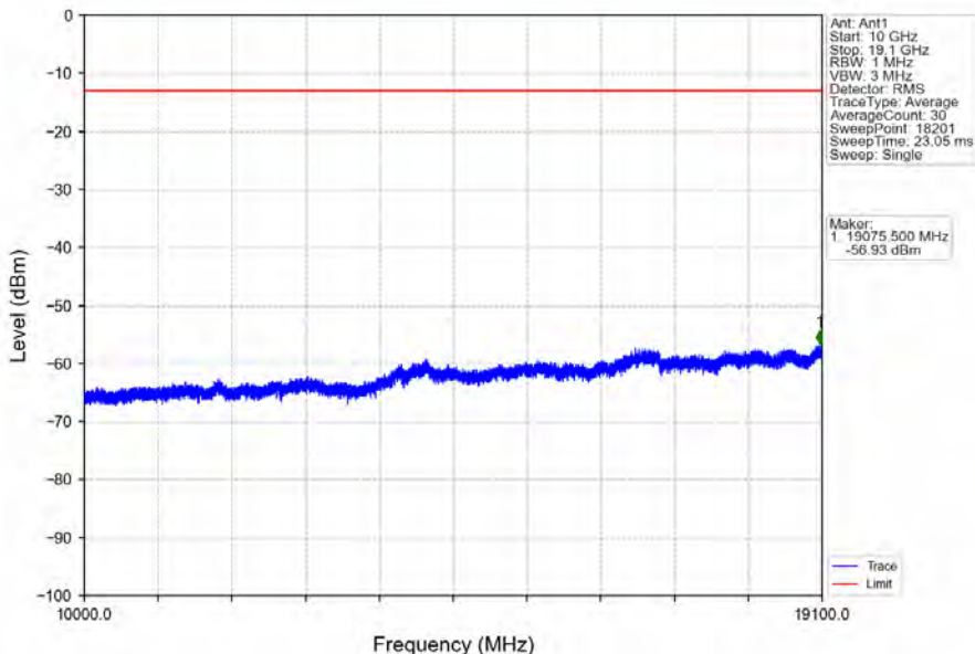
Band2_5MHz_QPSK_MCH_1880MHz_RB_1_0_NTNV
