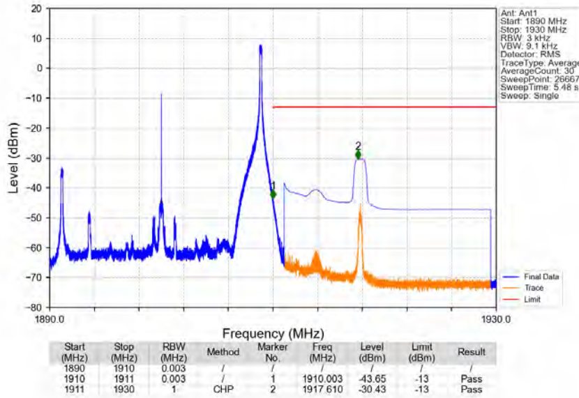
Band2_20MHz_QPSK_HCH_1900MHz_RB_1_99_NTNV
