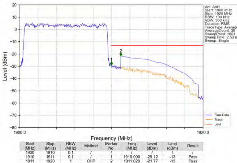
Band2_10MHz_QPSK_HCH_1905MHz_RB_50_0_NTNV
