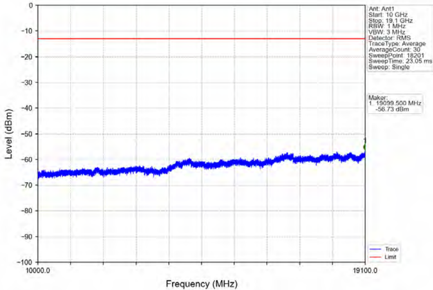
Band2_10MHz_64QAM_LCH_1855MHz_RB_50_0_NTNV
