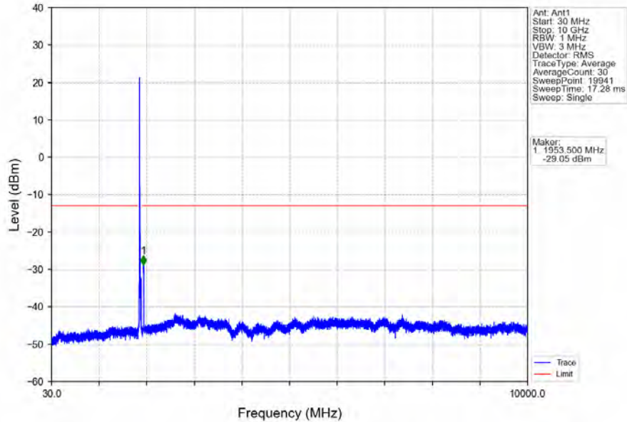
Band2_20MHz_16QAM_MCH_1880MHz_RB_1_0_NTNV
