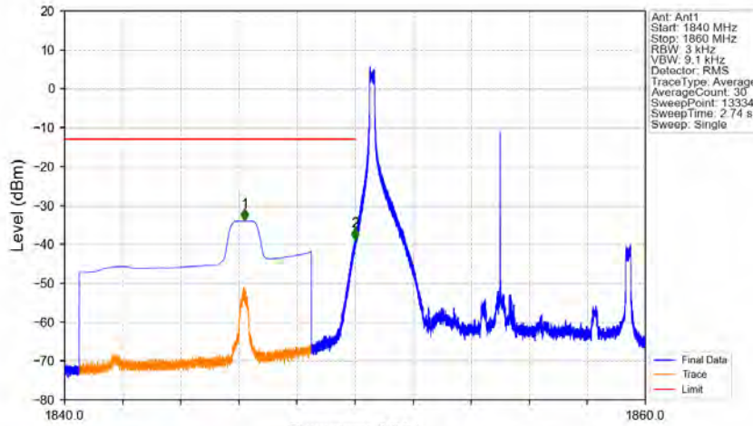
Band2_10MHz_64QAM_LCH_1855MHz_RB_1_0_NTNV
