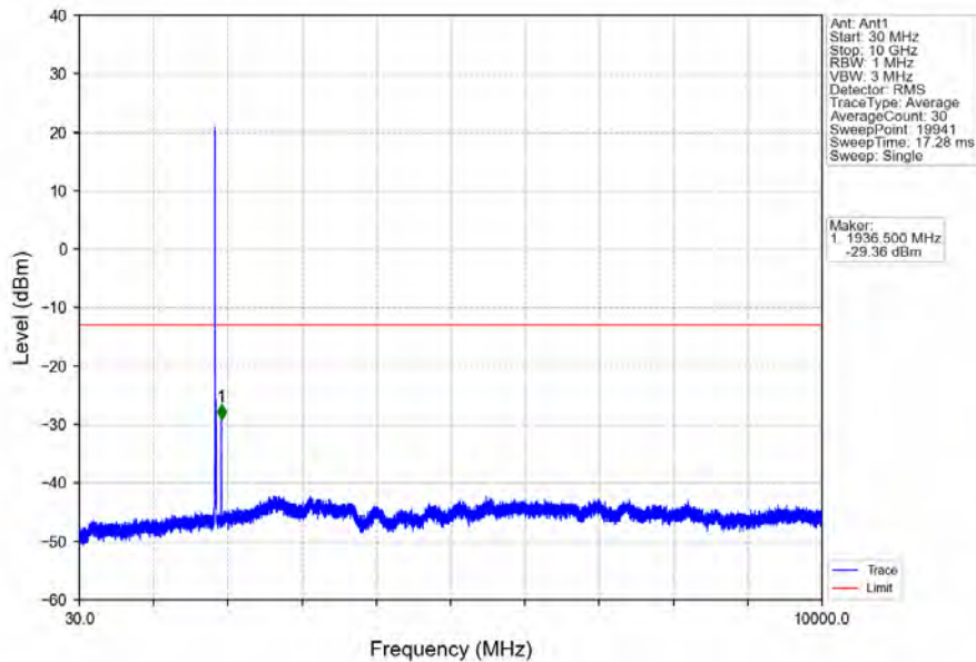
Band2_10MHz_64QAM_LCH_1855MHz_RB_1_0_NTNV
