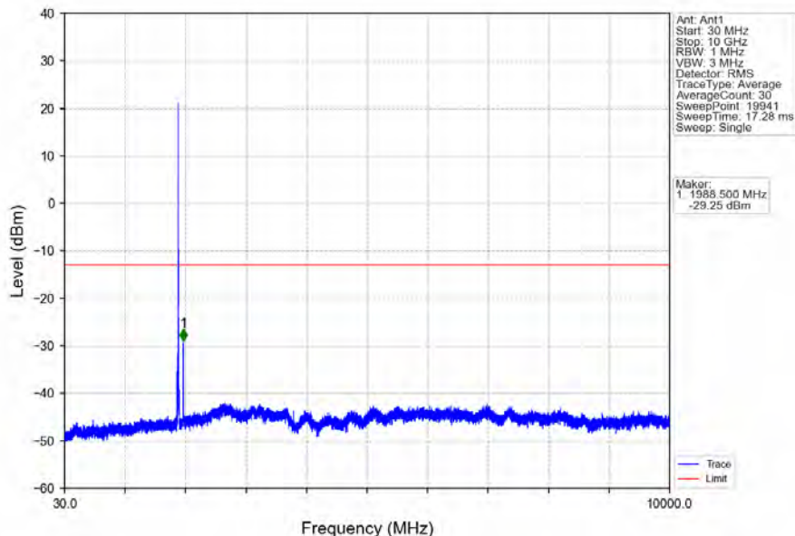
Band2_10MHz_16QAM_HCH_1905MHz_RB_1_0_NTNV
