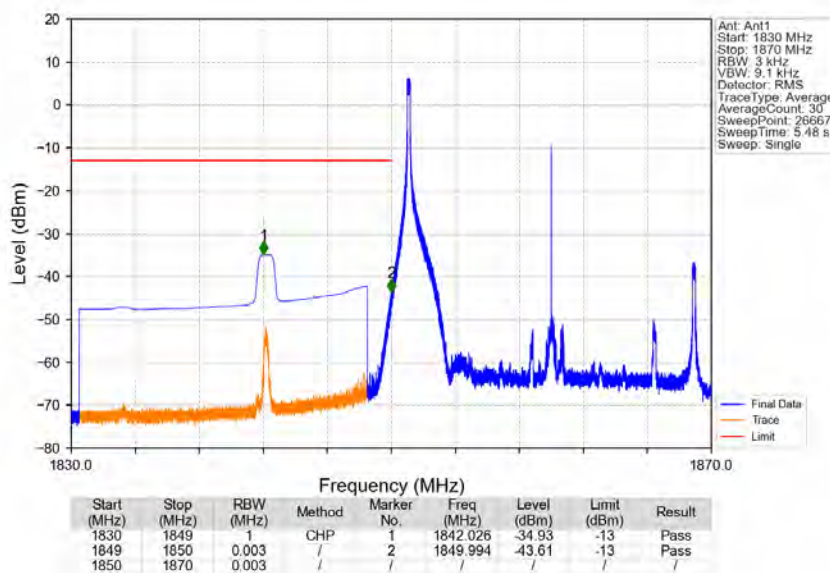
Band2_20MHz_16QAM_LCH_1860MHz_RB_1_0_NTNV
