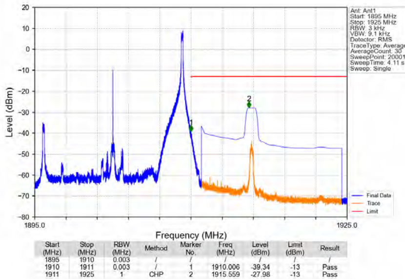
Band2_15MHz_QPSK_HCH_1902.5MHz_RB_1_74_NTNV
