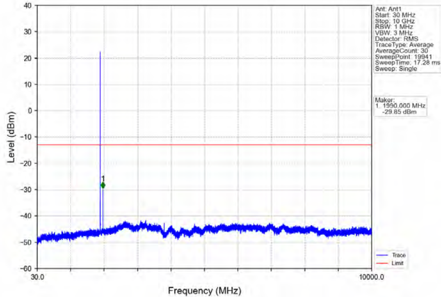
Band2_3MHz_QPSK_HCH_1908.5MHz_RB_1_0_NTNV
