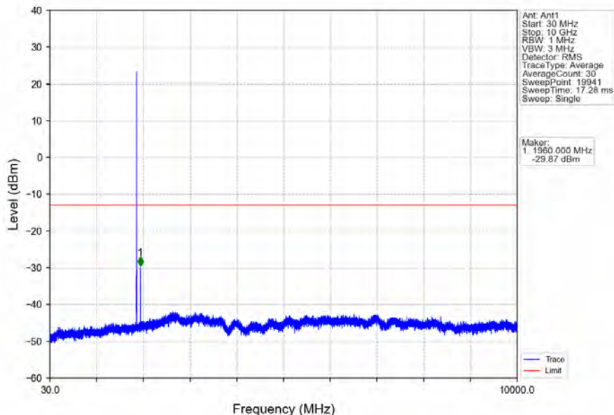
Band2_3MHz_QPSK_MCH_1880MHz_RB_1_0_NTNV
