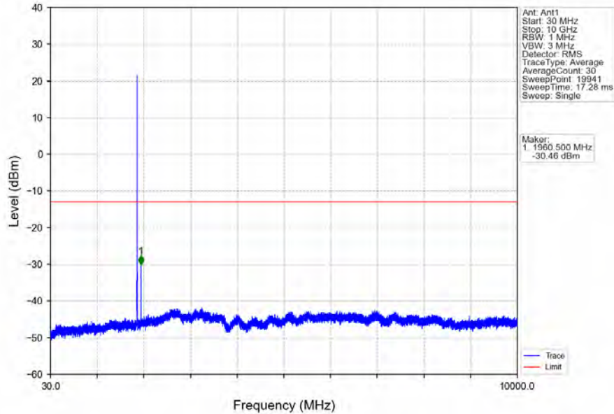
Band2_3MHz_16QAM_MCH_1880MHz_RB_1_0_NTNV
