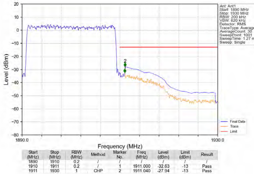
Band2_20MHz_16QAM_HCH_1900MHz_RB_100_0_NTNV
