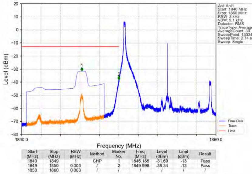
Band2_10MHz_16QAM_LCH_1855MHz_RB_1_0_NTNV
