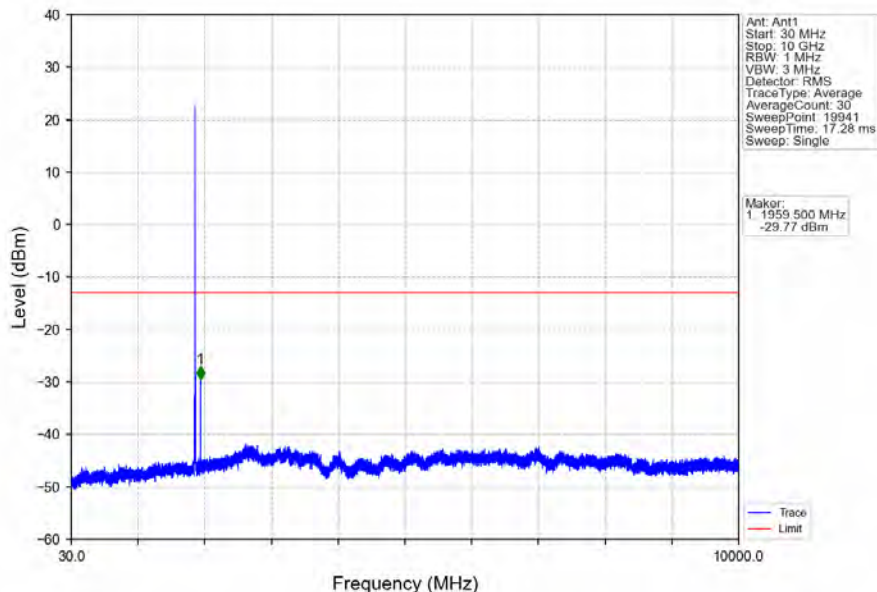
Band2_5MHz_QPSK_MCH_1880MHz_RB_1_0_NTNV
