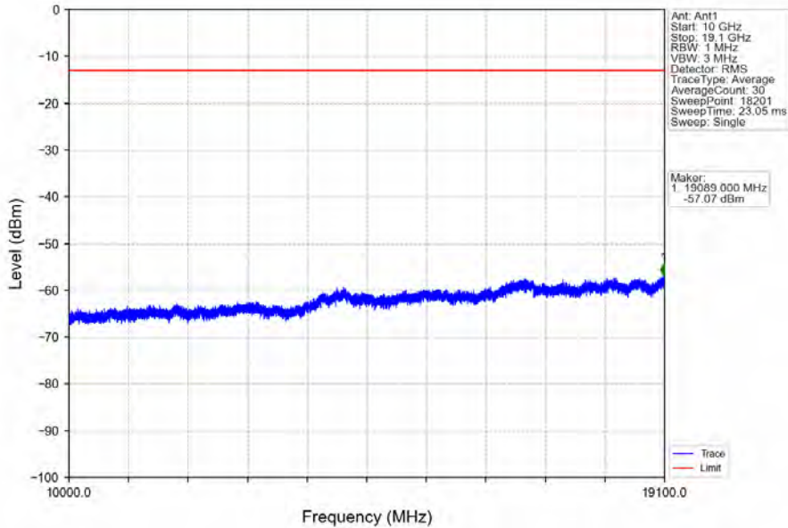
Band2_20MHz_64QAM_LCH_1860MHz_RB_100_0_NTNV
