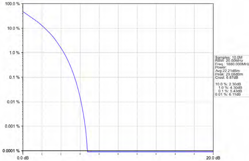
Band2_20MHz_QPSK_MCH_1880MHz_RB_100_0_NTNV
