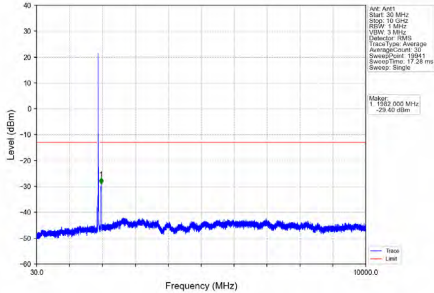
Band2_20MHz_16QAM_HCH_1900MHz_RB_1_0_NTNV
