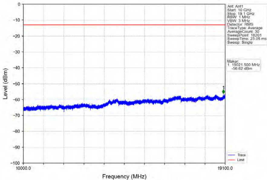
Band2_20MHz_16QAM_HCH_1900MHz_RB_1_0_NTNV
