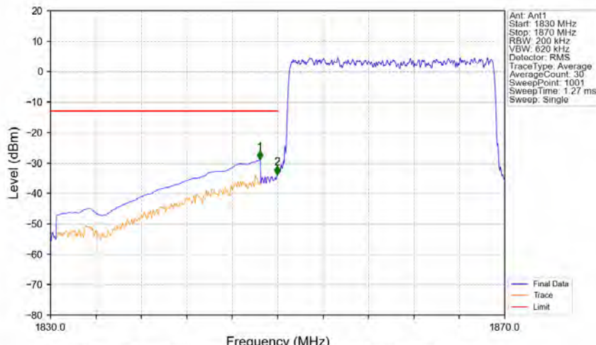
Band2_20MHz_QPSK_LCH_1860MHz_RB_100_0_NTNV
