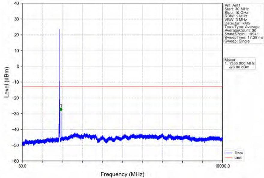
Band2_15MHz_QPSK_MCH_1880MHz_RB_1_0_NTNV
