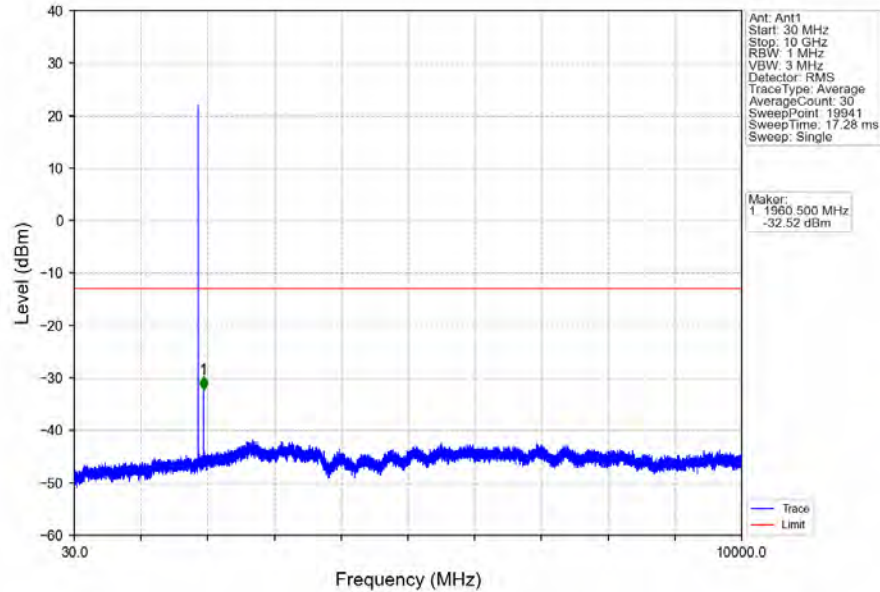
Band2_1.4MHz_QPSK_MCH_1880MHz_RB_1_0_NTNV
