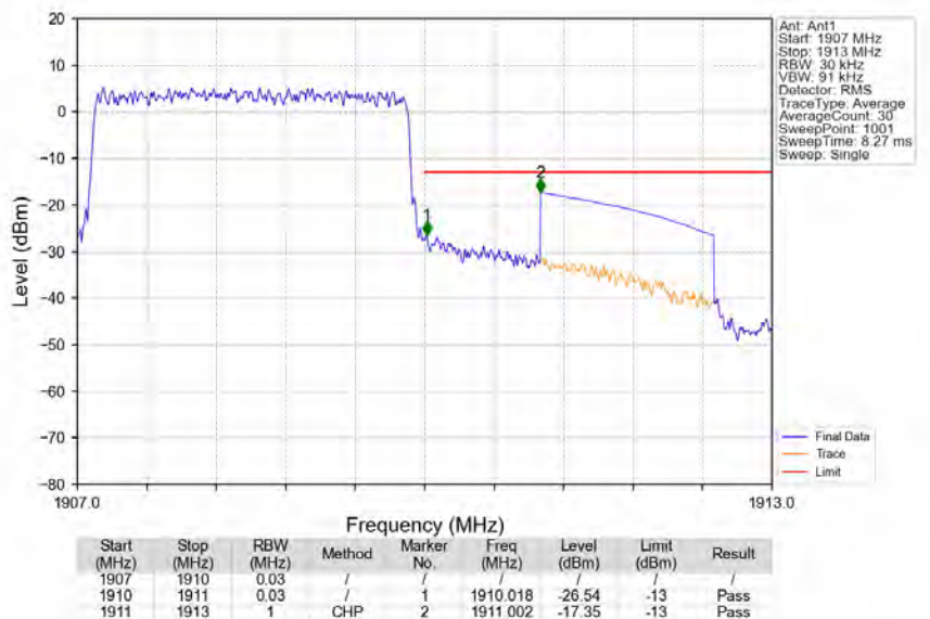
Band2_3MHz_QPSK_HCH_1908.5MHz_RB_15_0_NTNV
