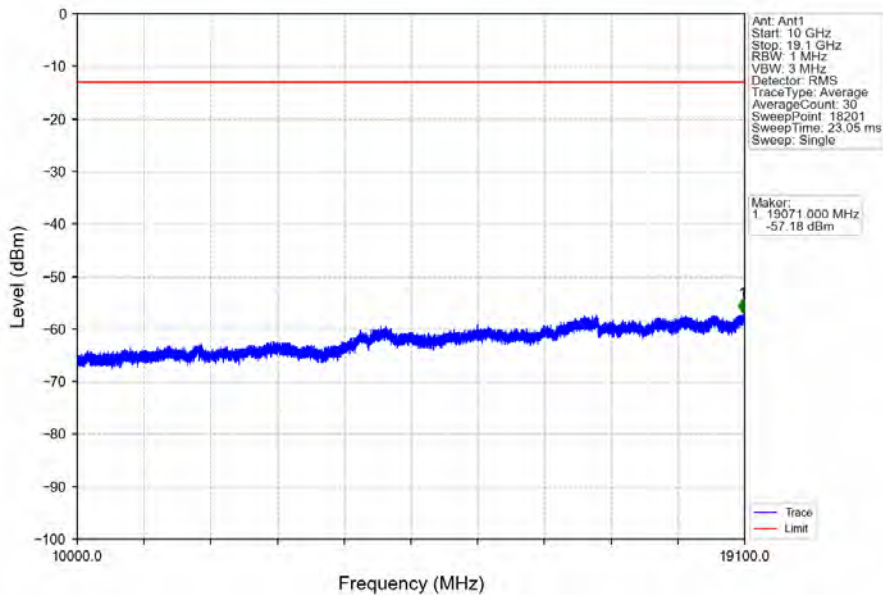
Band2_3MHz_16QAM_MCH_1880MHz_RB_1_0_NTNV
