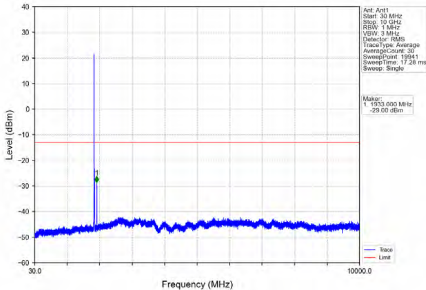
Band2_10MHz_16QAM_LCH_1855MHz_RB_1_0_NTNV
