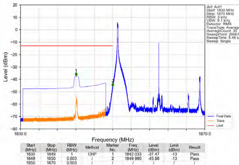
Band2_20MHz_64QAM_LCH_1860MHz_RB_1_0_NTNV
