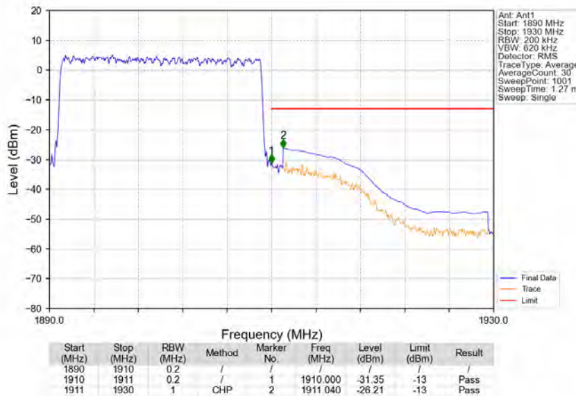
Band2_20MHz_QPSK_HCH_1900MHz_RB_100_0_NTNV
