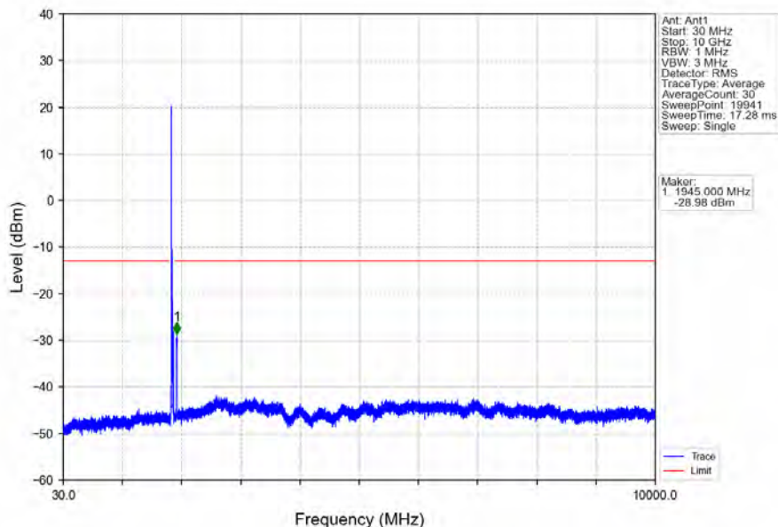
Band2_20MHz_64QAM_LCH_1860MHz_RB_1_0_NTNV
