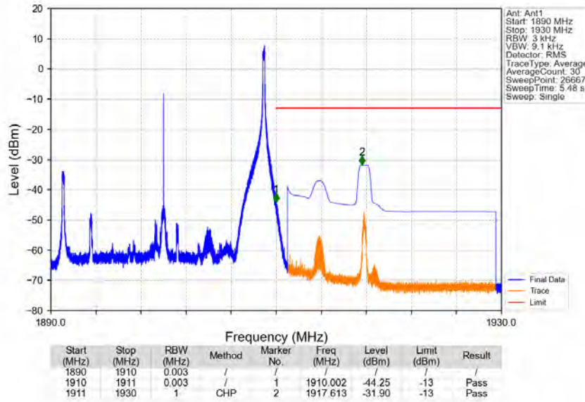
Band2_20MHz_16QAM_HCH_1900MHz_RB_1_99_NTNV
