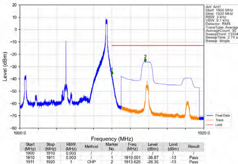
Band2_10MHz_QPSK_HCH_1905MHz_RB_1_49_NTNV
