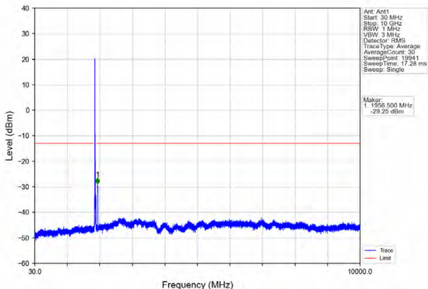
Band2_20MHz_64QAM_MCH_1880MHz_RB_1_0_NTNV
