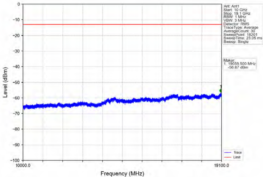
Band2_15MHz_QPSK_HCH_1902.5MHz_RB_1_0_NTNV
