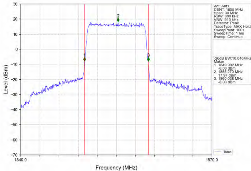
Band2_10MHz_QPSK_LCH_1855MHz_RB_50_0_NTNV
