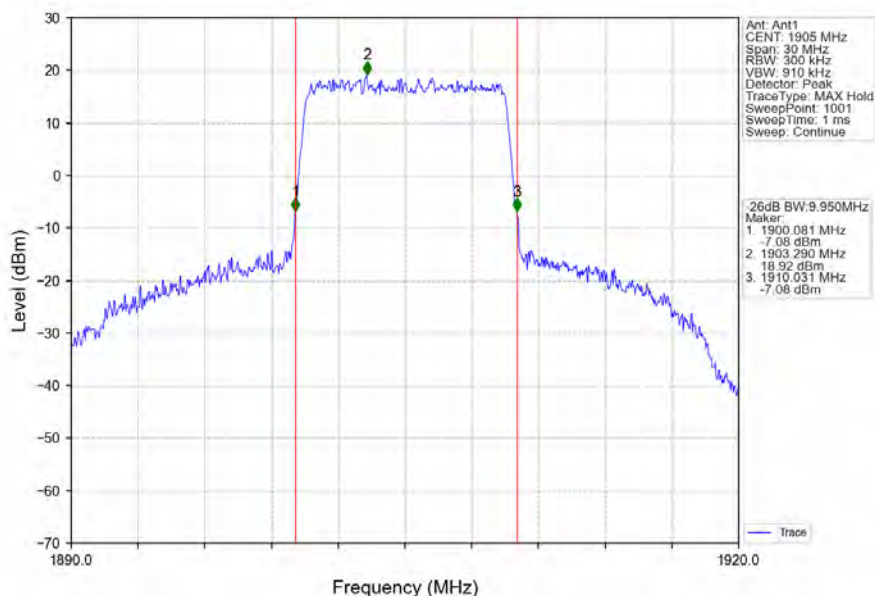
Band2_10MHz_QPSK_HCH_1905MHz_RB_50_0_NTNV
