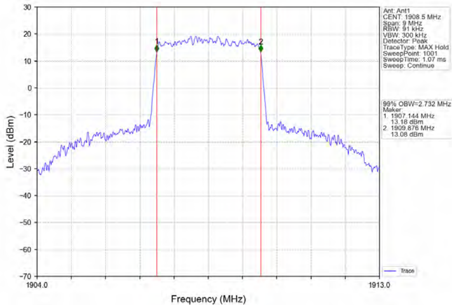
Band2_3MHz_QPSK_HCH_1908.5MHz_RB_15_0_NTNV
