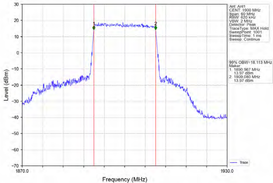
Band2_20MHz_QPSK_HCH_1900MHz_RB_100_0_NTNV
