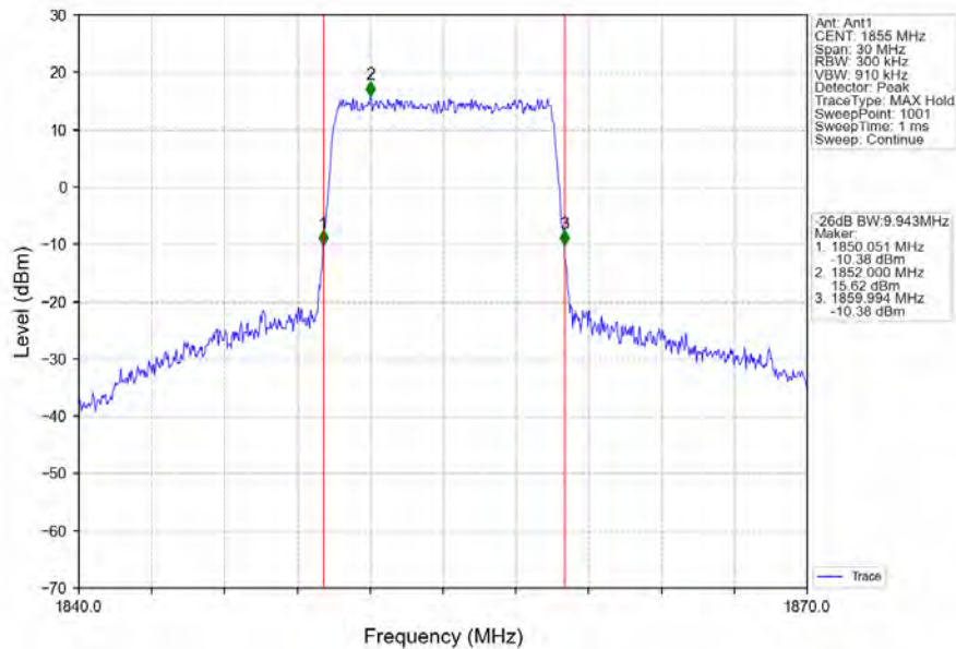
Band2_10MHz_64QAM_LCH_1855MHz_RB_50_0_NTNV
