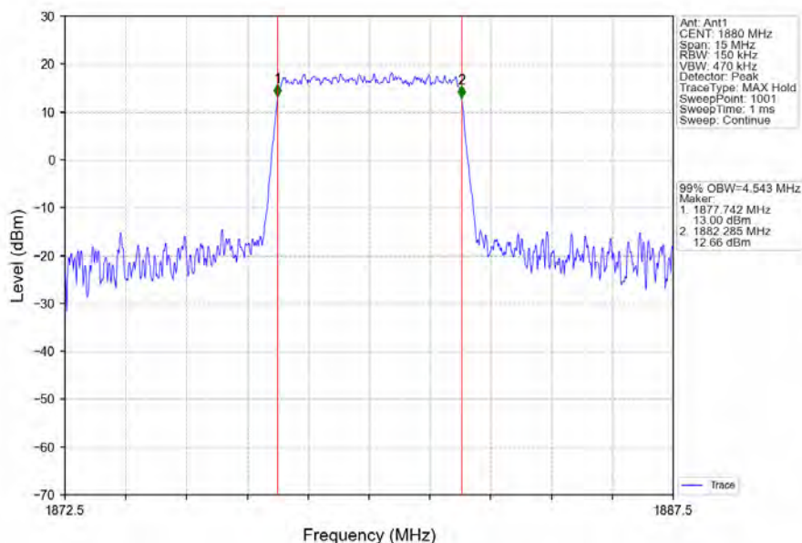
Band2_5MHz_QPSK_MCH_1880MHz_RB_25_0_NTNV
