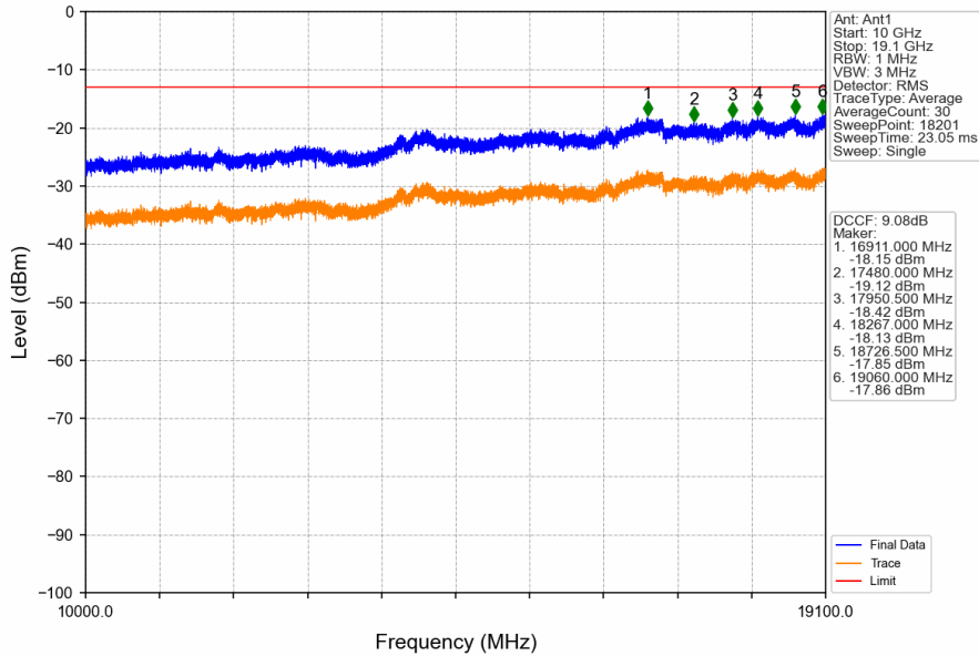
PCS1900_GSM_HCH_1909.8MHz_GSM_NTNV
