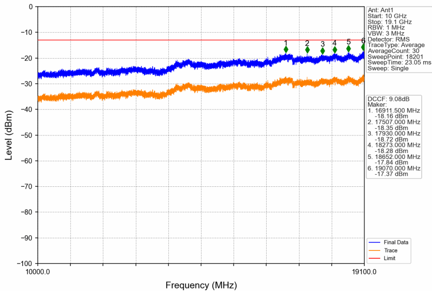
PCS1900_GSM_HCH_1909.8MHz_GSM_NTNV
