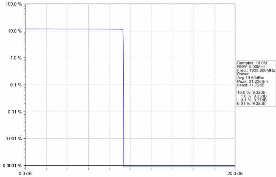
PCS1900_GSM_HCH_1909.8MHz_GSM_NTNV
