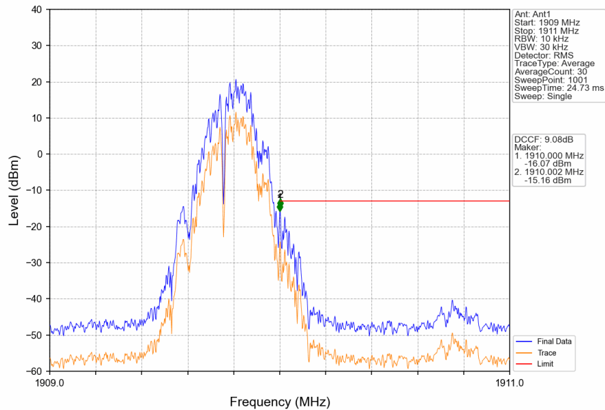
PCS1900_GSM_HCH_1909.8MHz_GSM_NTNV
