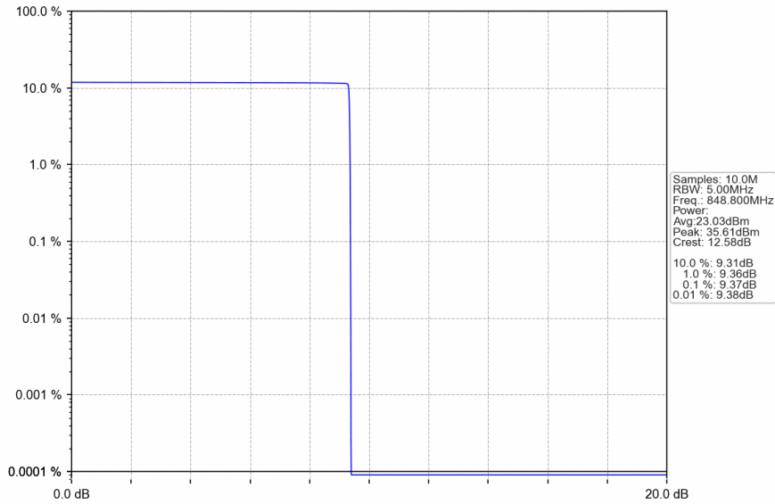
GSM850_GSM_HCH_848.8MHz_GSM_NTNV
