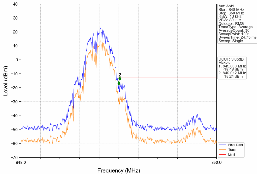
GSM850_GSM_HCH_848.8MHz_GSM_NTNV
