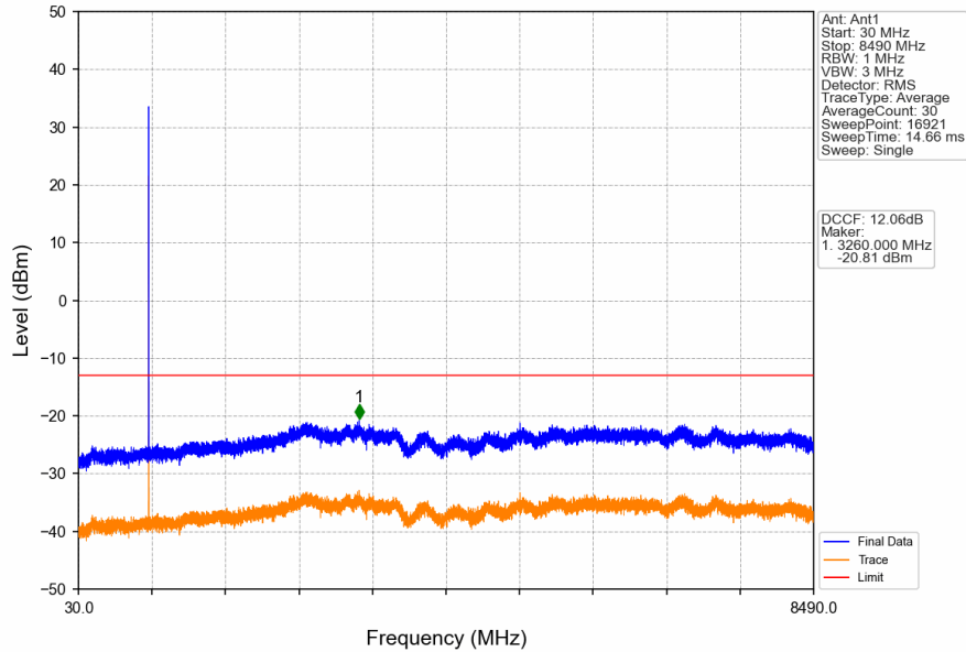
GSM850_GSM_HCH_848.8MHz_GSM_NTNV
