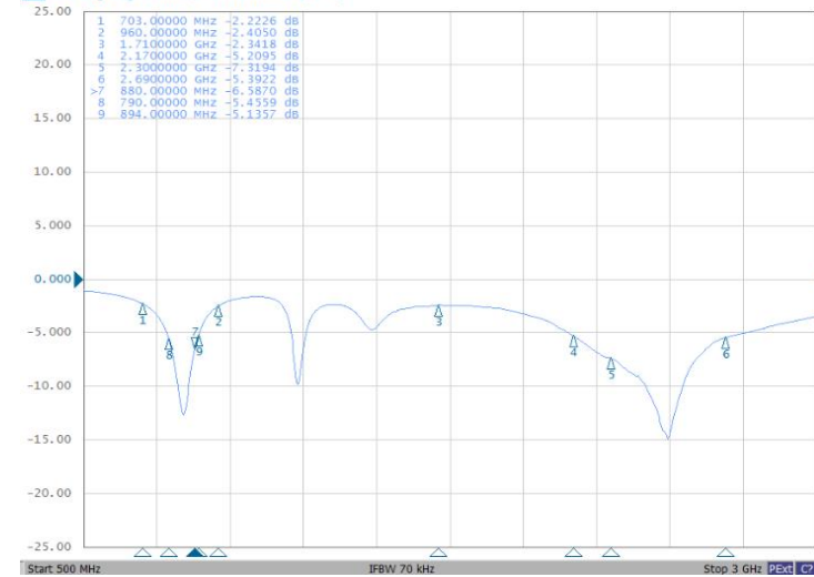
511 Log Mag 5.000dB/ Ref 0.000dB [F1 M]
