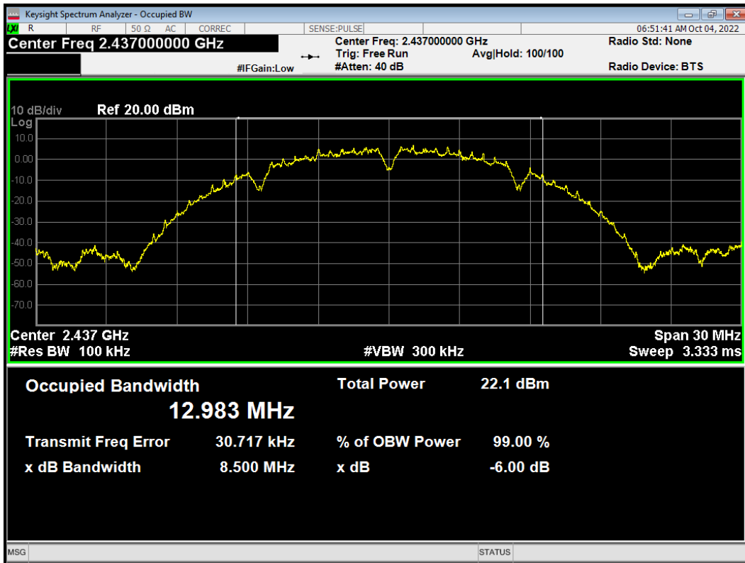
-6dB Bandwidth 802.11b 2437MHz
