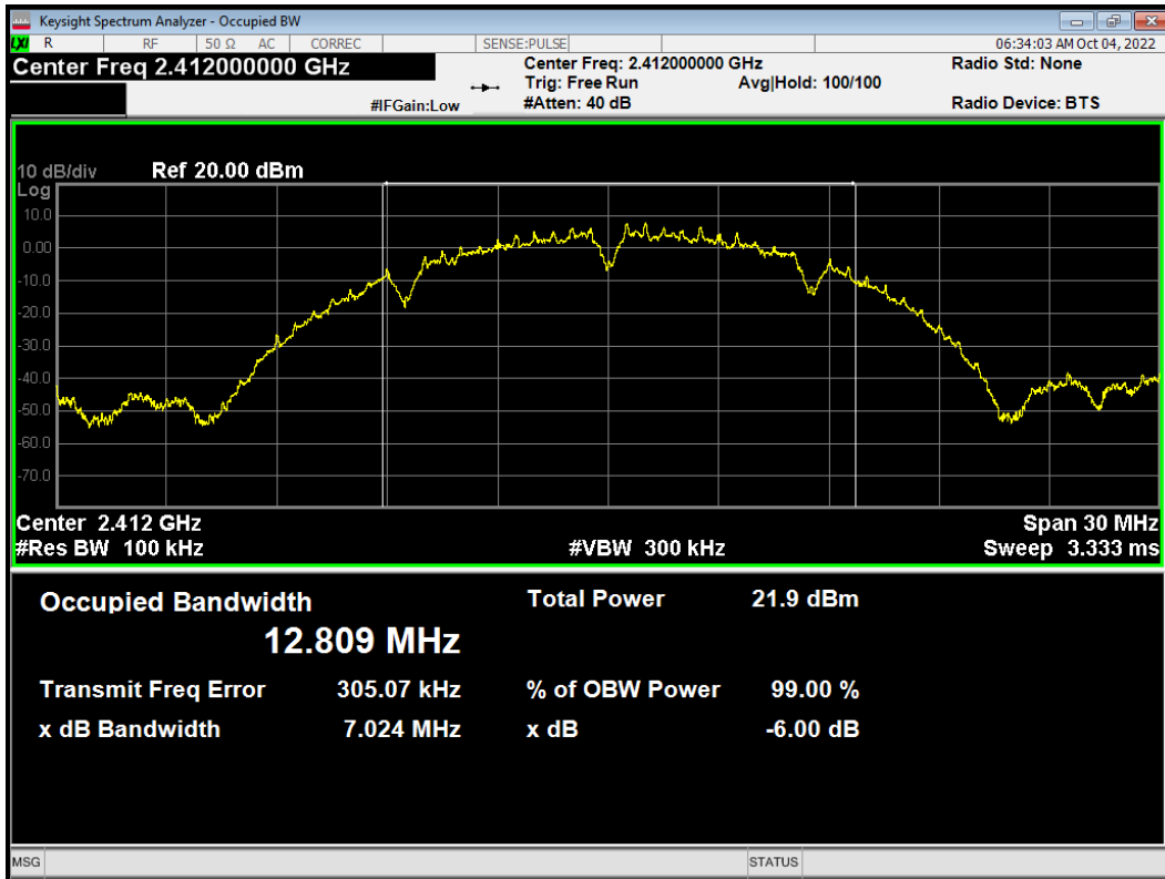
-6dB Bandwidth 802.11b 2412MHz
