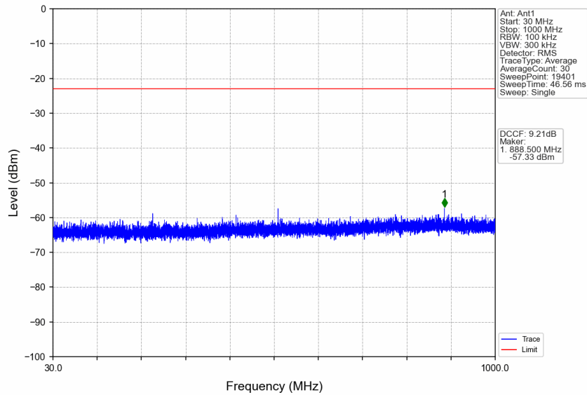
n77d_15kHz_SISO_NTNV_20MHz_CP-OFDM QPSK_3499.995MHz_Edge_1RB_Left
