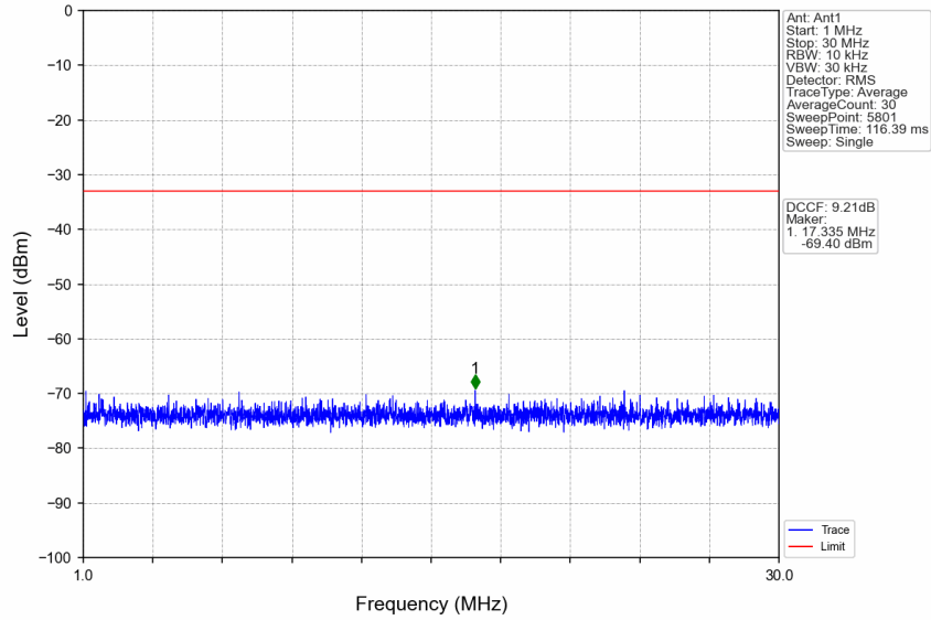
n77d_15kHz_SISO_NTNV_20MHz_CP-OFDM QPSK_3499.995MHz_Edge_1RB_Left
