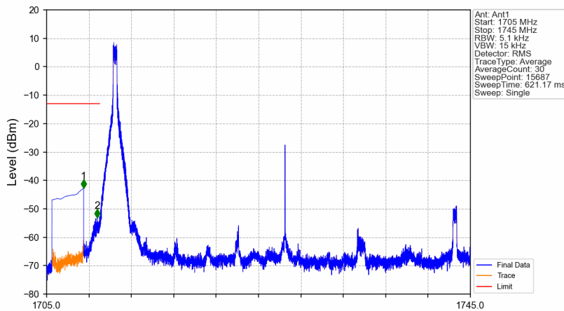
n66_30kHz_SISO_NTNV_35MHz_CP-OFDM QPSK_1727.5MHz_Inner_1RB_Left
