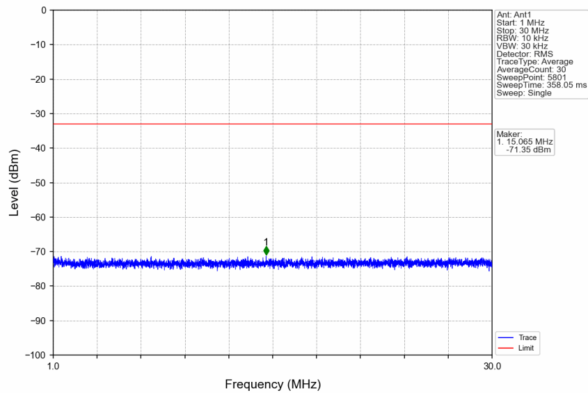
n66_30kHz_SISO_NTNV_20MHz_CP-OFDM QPSK_1745MHz_Edge_1RB_Left
