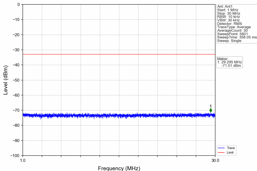
n66_30kHz_SISO_NTNV_20MHz_CP-OFDM QPSK_1720MHz_Edge_1RB_Left
