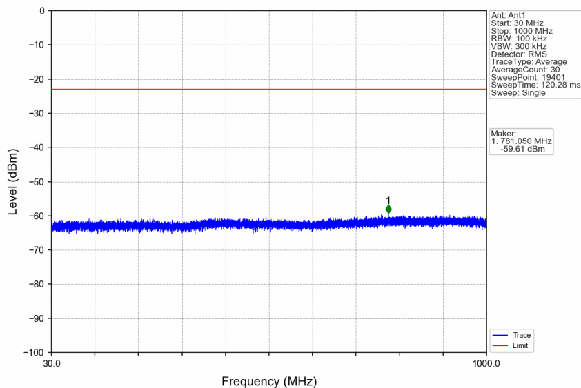
n66_30kHz_SISO_NTNV_20MHz_CP-OFDM QPSK_1720MHz_Edge_1RB_Left
