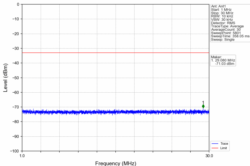
n66_30kHz_SISO_NTNV_20MHz_DFT-s-OFDM QPSK_1720MHz_Edge_1RB_Left
