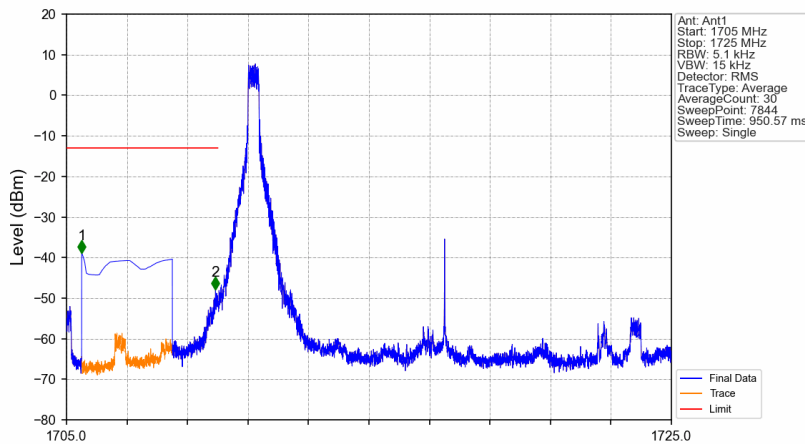
n66_30kHz_SISO_NTNV_15MHz_CP-OFDM QPSK_1717.5MHz_Inner_1RB_Left
