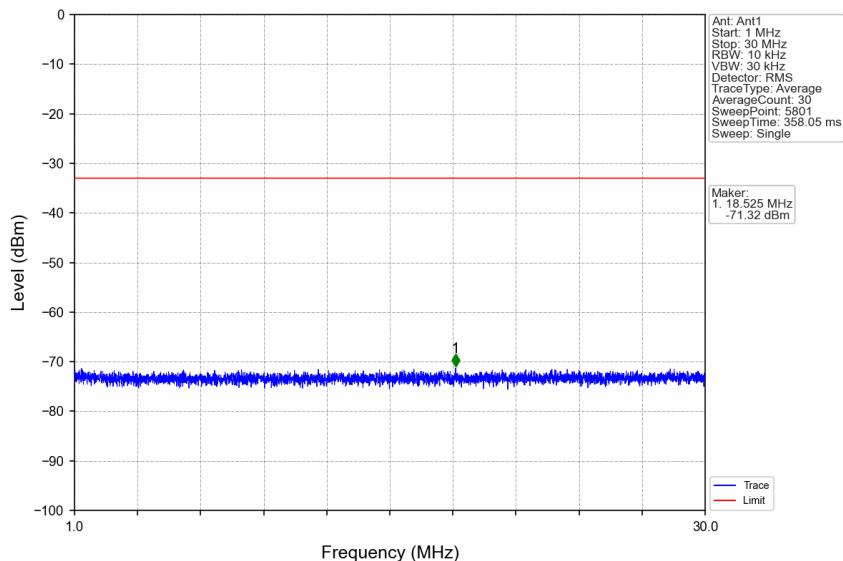
n66_15kHz_SISO_NTNV_20MHz_DFT-s-OFDM QPSK_1720MHz_Edge_1RB_Left
