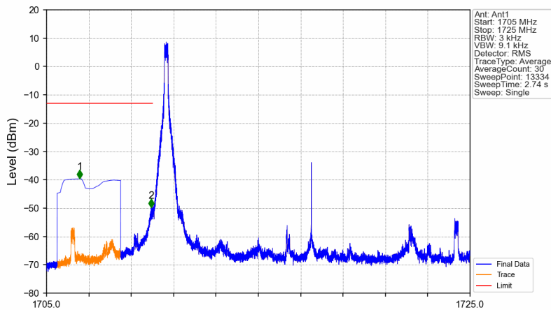
n66_15kHz_SISO_NTNV_15MHz_CP-OFDM QPSK_1717.5MHz_Inner_1RB_Left
