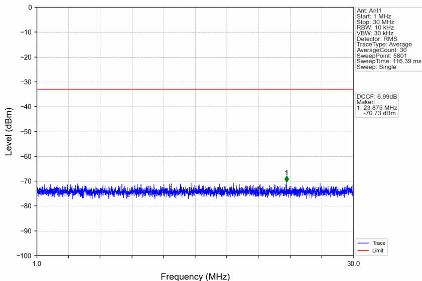
n41_30kHz_SISO_NTNV_90MHz_CP-OFDM QPSK_2541MHz_Edge_1RB_Left
