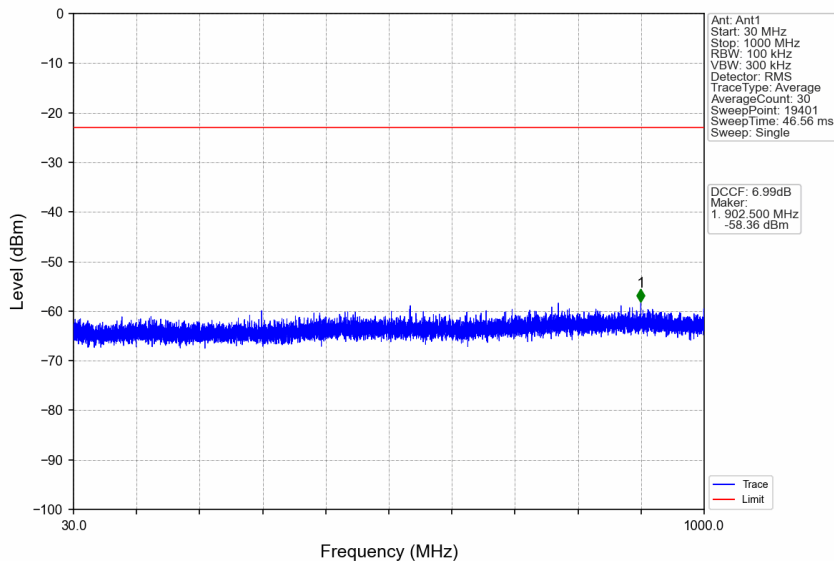
n41_30kHz_SISO_NTNV_90MHz_CP-OFDM QPSK_2541MHz_Edge_1RB_Left
