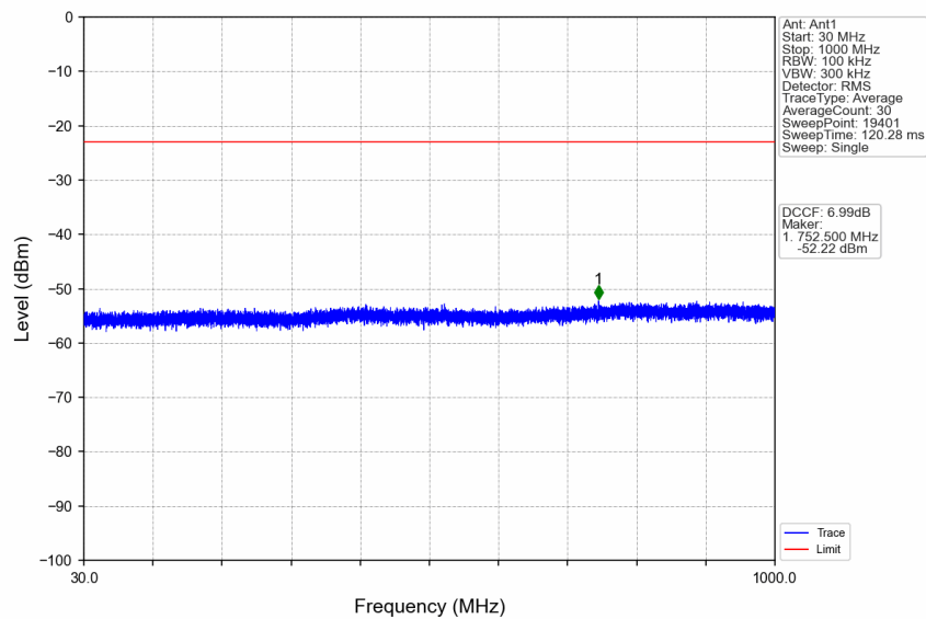
n41_30kHz_SISO_NTNV_70MHz_CP-OFDM QPSK_2531.01MHz_Edge_1RB_Left
