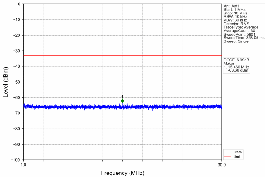
n41_30kHz_SISO_NTNV_70MHz_DFT-s-OFDM QPSK_2592.99MHz_Edge_1RB_Left
