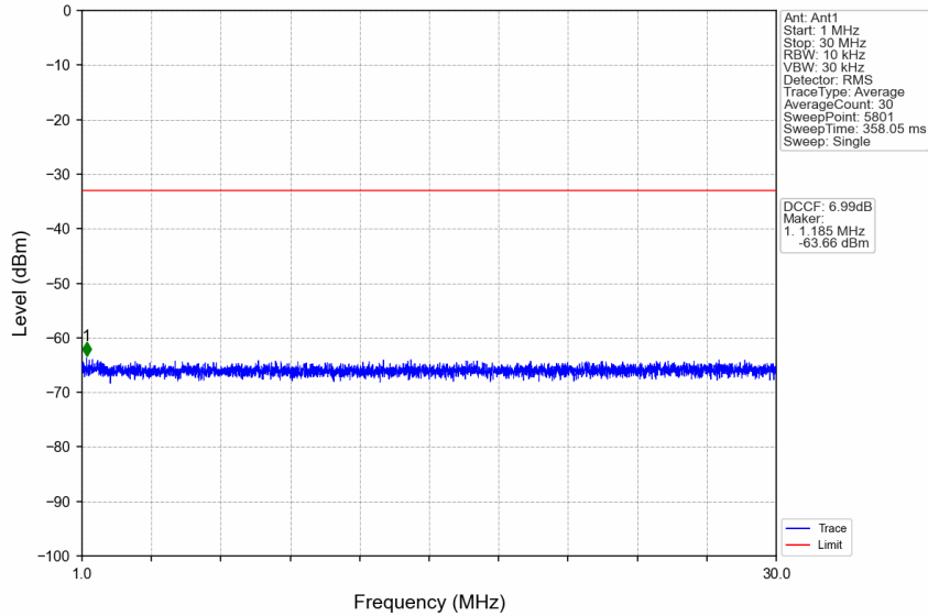
n41_30kHz_SISO_NTNV_70MHz_CP-OFDM QPSK_2592.99MHz_Edge_1RB_Left
