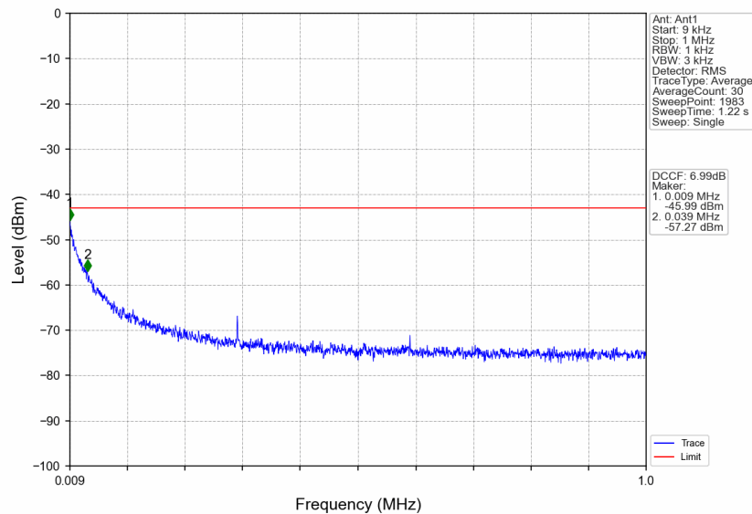
n41_30kHz_SISO_NTNV_70MHz_CP-OFDM QPSK_2655MHz_Edge_1RB_Right
