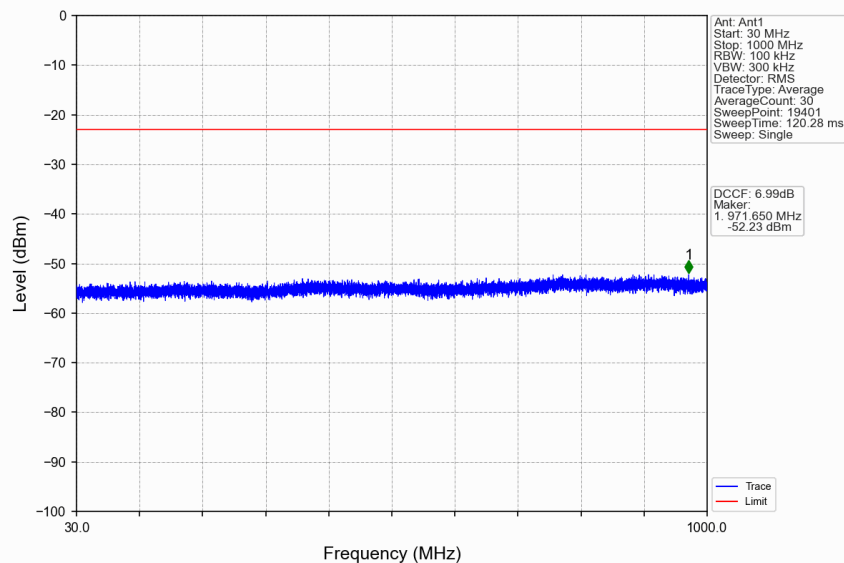
n41_30kHz_SISO_NTNV_60MHz_CP-OFDM QPSK_2526MHz_Edge_1RB_Left
