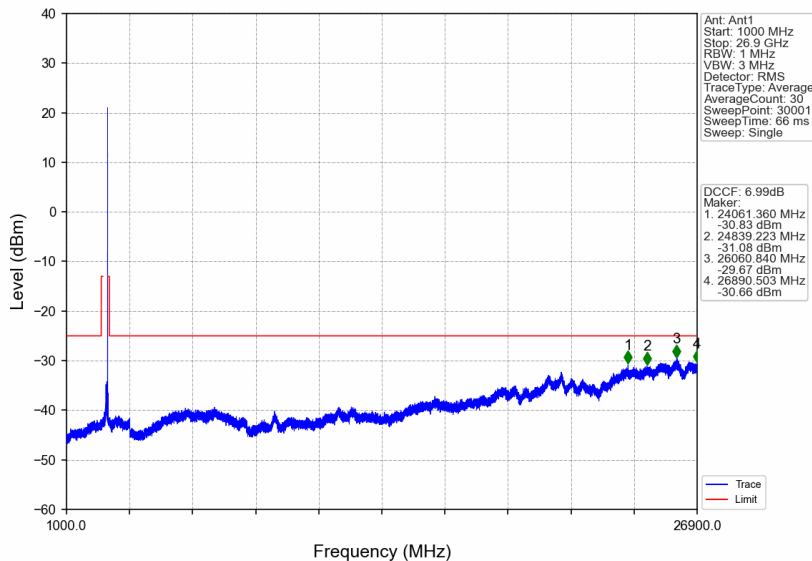
n41_30kHz_SISO_NTNV_70MHz_CP-OFDM QPSK_2655MHz_Edge_1RB_Right
