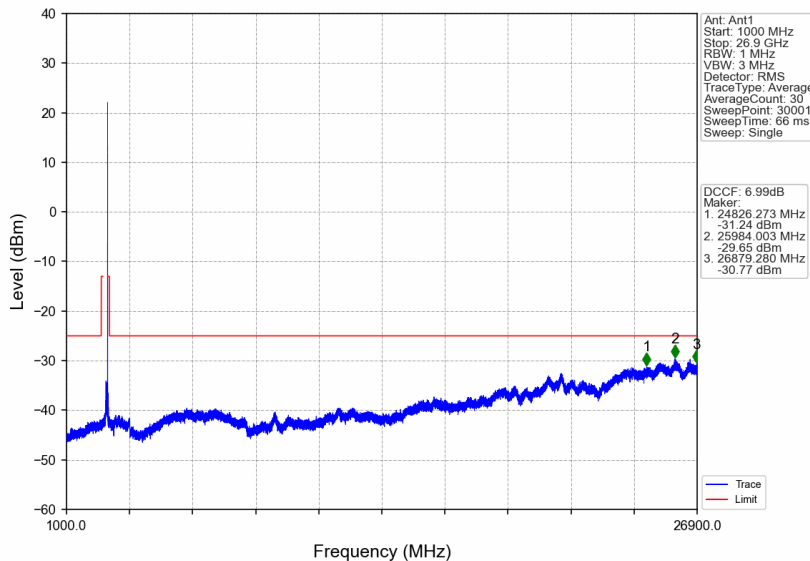
n41_30kHz_SISO_NTNV_70MHz_DFT-s-OFDM_QPSK_2655MHz_Edge_1RB_Right
