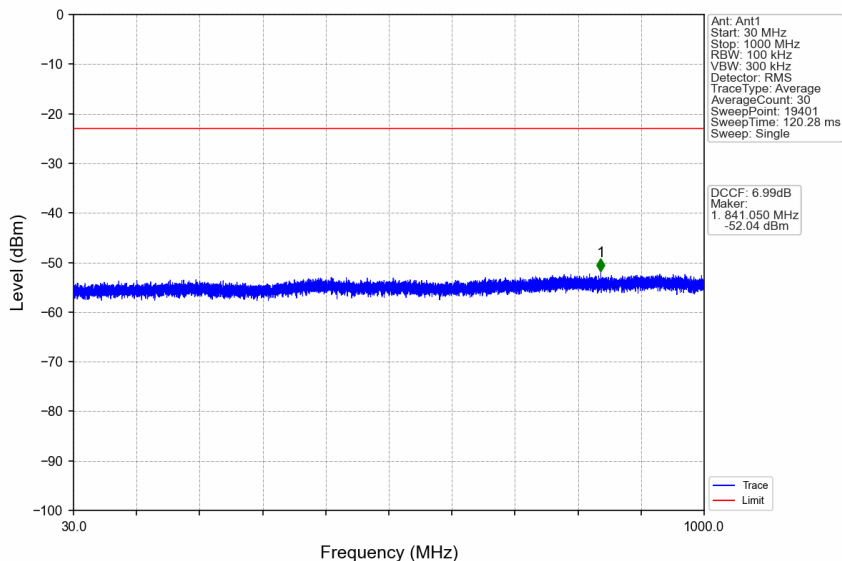
n41_30kHz_SISO_NTNV_70MHz_DFT-s-OFDM_QPSK_2655MHz_Edge_1RB_Right
