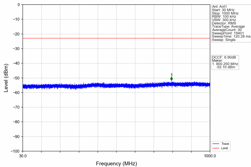
n41_30kHz_SISO_NTNV_60MHz_DFT-s-OFDM QPSK_2592.99MHz_Edge_1RB_Left
