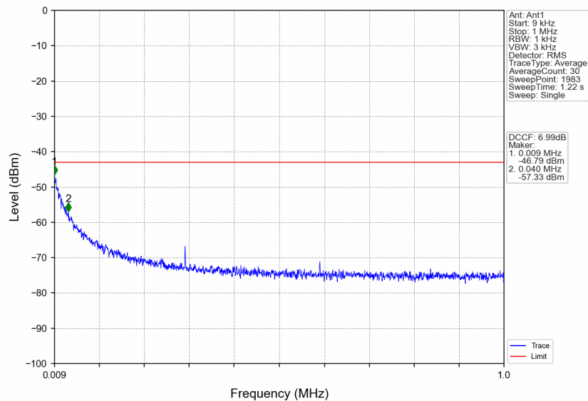
n41_30kHz_SISO_NTNV_70MHz_DFT-s-OFDM QPSK_2655MHz_Edge_1RB_Right
