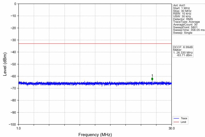
n41_30kHz_SISO_NTNV_70MHz_DFT-s-OFDM QPSK_2655MHz_Edge_1RB_Right
