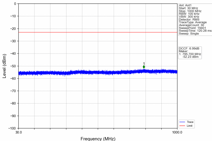
n41_30kHz_SISO_NTNV_70MHz_CP-OFDM QPSK_2655MHz_Edge_1RB_Right
