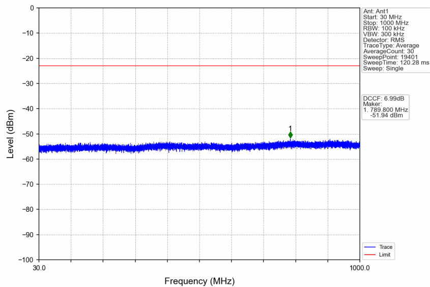
n41_30kHz_SISO_NTNV_70MHz_DFT-s-OFDM QPSK_2531.01MHz_Edge_1RB_Left
