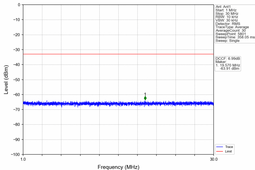
n41_30kHz_SISO_NTNV_70MHz_CP-OFDM QPSK_2655MHz_Edge_1RB_Right
