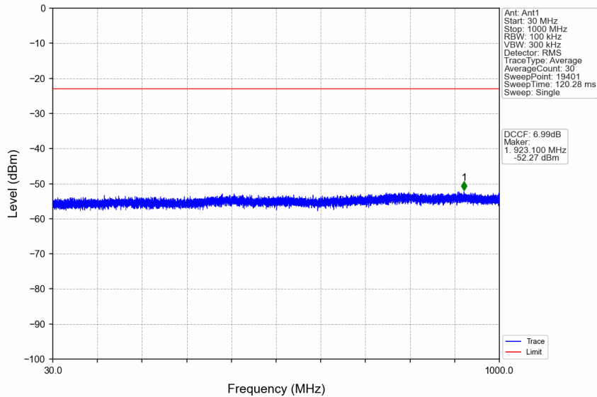
n41_30kHz_SISO_NTNV_25MHz_DFT-s-OFDM PI/2 BPSK_2508.51MHz_Edge_1RB_Left
