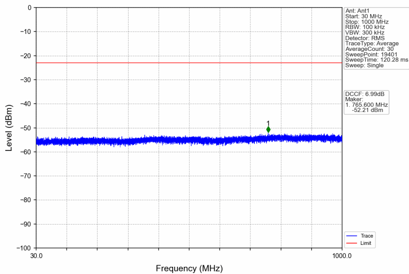
n41_30kHz_SISO_NTNV_20MHz_CP-OFDM QPSK_2506.02MHz_Edge_1RB_Left
