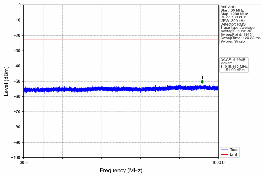
n41_30kHz_SISO_NTNV_25MHz_CP-OFDM QPSK_2508.51MHz_Edge_1RB_Left
