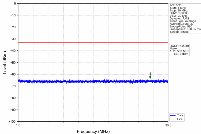
n41_30kHz_SISO_NTNV_20MHz_DFT-s-OFDM QPSK_2506.02MHz_Edge_1RB_Left
