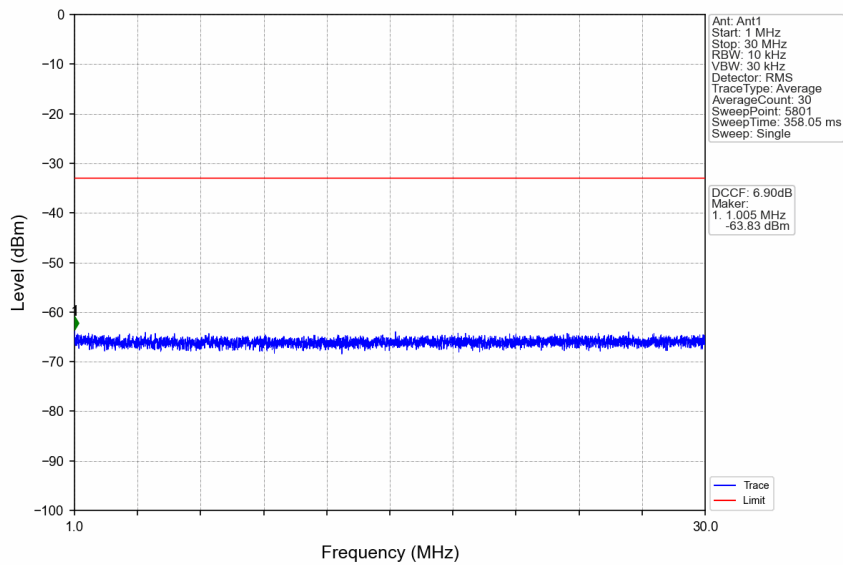
n41_30kHz_SISO_NTNV_25MHz_DFT-s-OFDM QPSK_2508.51MHz_Edge_1RB_Left
