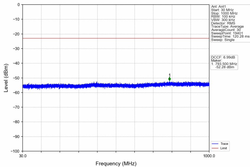
n41_30kHz_SISO_NTNV_20MHz_CP-OFDM QPSK_2592.99MHz_Edge_1RB_Left
