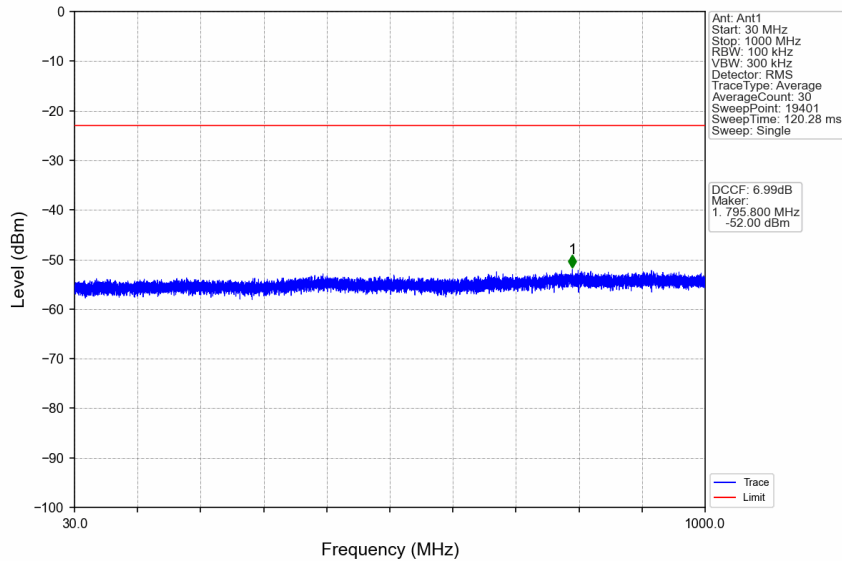
n41_15kHz_SISO_NTNV_50MHz_DFT-s-OFDM PI/2 BPSK_2593.005MHz_Edge_1RB_Left
