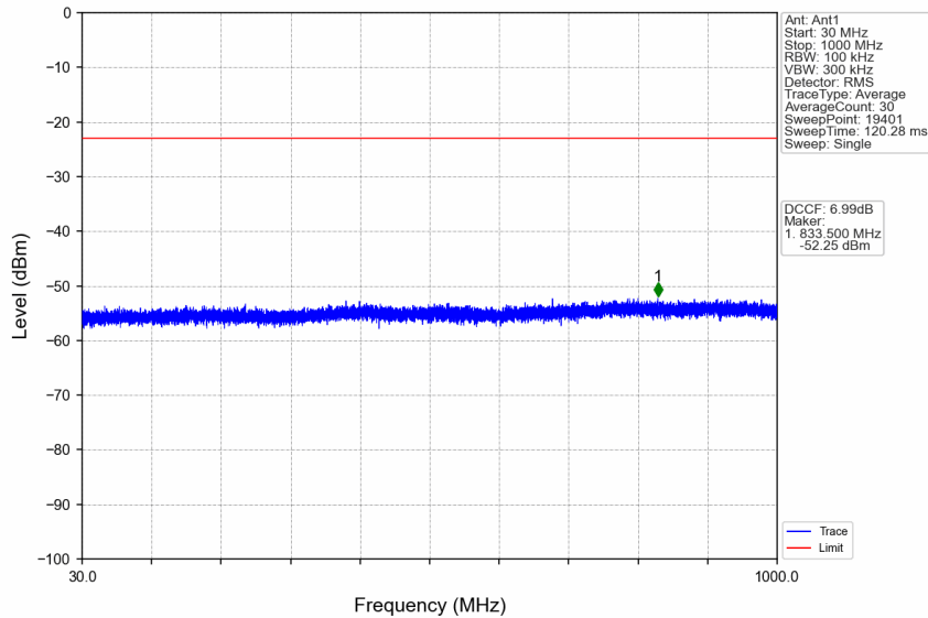
n41_15kHz_SISO_NTNV_50MHz_CP-OFDM QPSK_2521.005MHz_Edge_1RB_Left
