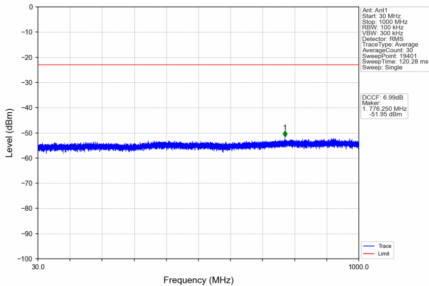
n41_15kHz_SISO_NTNV_50MHz_DFT-s-OFDM QPSK_2521.005MHz_Edge_1RB_Left
