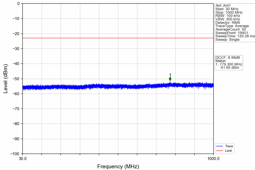
n41_15kHz_SISO_NTNV_40MHz_CP-OFDM QPSK_2593.005MHz_Edge_1RB_Left
