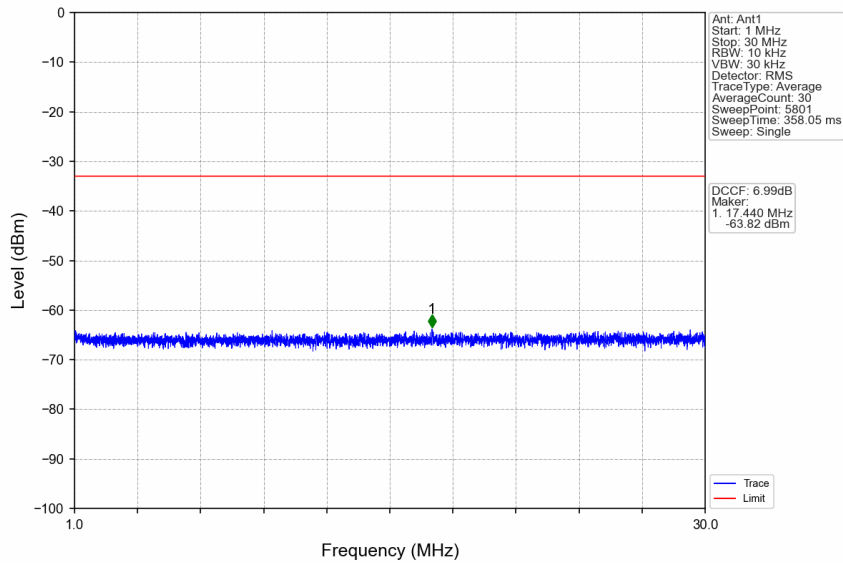
n41_15kHz_SISO_NTNV_30MHz_CP-OFDM QPSK_2593.005MHz_Edge_1RB_Left
