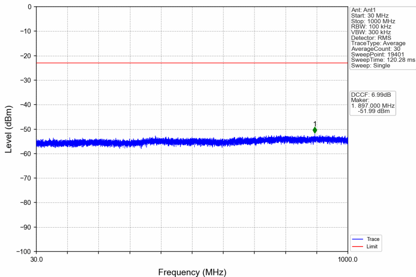
n41_15kHz_SISO_NTNV_30MHz_CP-OFDM QPSK_2511MHz_Edge_1RB_Left
