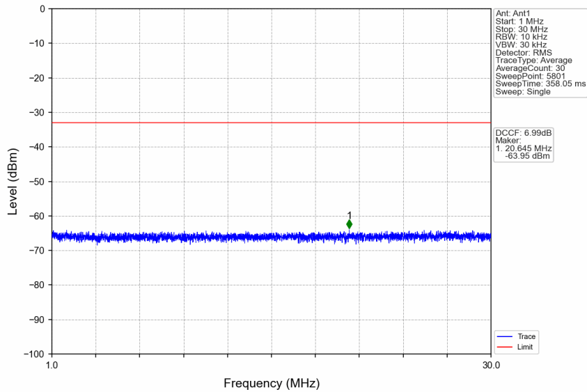
n41_15kHz_SISO_NTNV_25MHz_DFT-s-OFDM QPSK_2508.51MHz_Edge_1RB_Left
