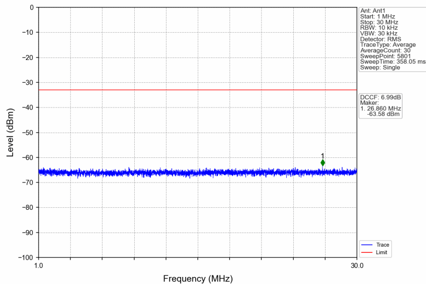
n41_15kHz_SISO_NTNV_20MHz_CP-OFDM QPSK_2506.005MHz_Edge_1RB_Left
