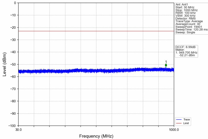
n41_15kHz_SISO_NTNV_25MHz_DFT-s-OFDM QPSK_2508.51MHz_Edge_1RB_Left
