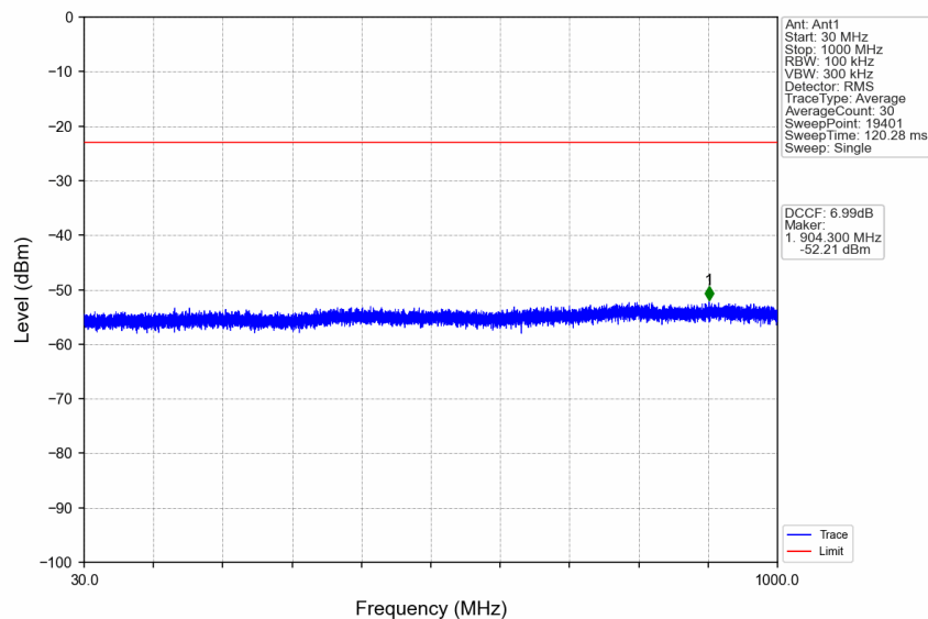
n41_15kHz_SISO_NTNV_25MHz_CP-OFDM QPSK_2593.005MHz_Edge_1RB_Left
