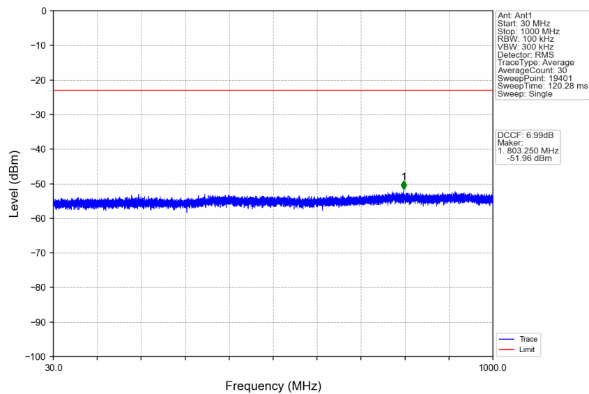
n41_15kHz_SISO_NTNV_25MHz_CP-OFDM QPSK_2508.51MHz_Edge_1RB_Left
