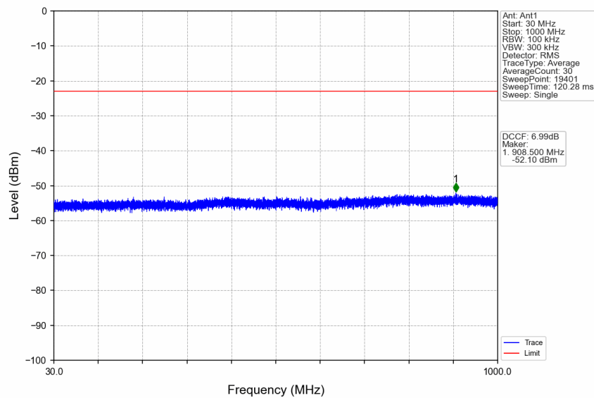
n41_15kHz_SISO_NTNV_20MHz_DFT-s-OFDM PI/2 BPSK_2506.005MHz_Edge_1RB_Left
