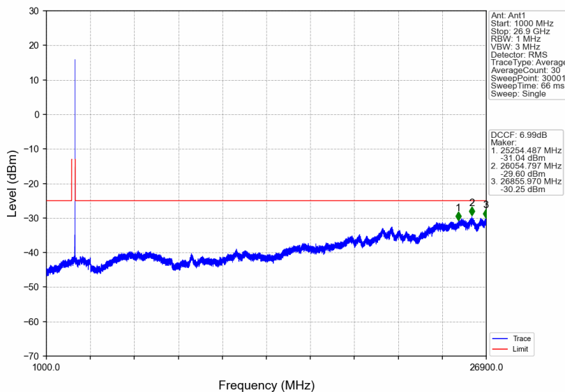
n41_15kHz_SISO_NTNV_10MHz_CP-OFDM QPSK_2685MHz_Edge_1RB_Right
