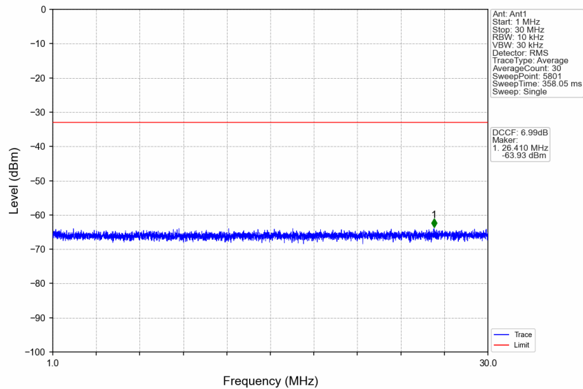
n41_15kHz_SISO_NTNV_10MHz_CP-OFDM QPSK_2685MHz_Edge_1RB_Right
