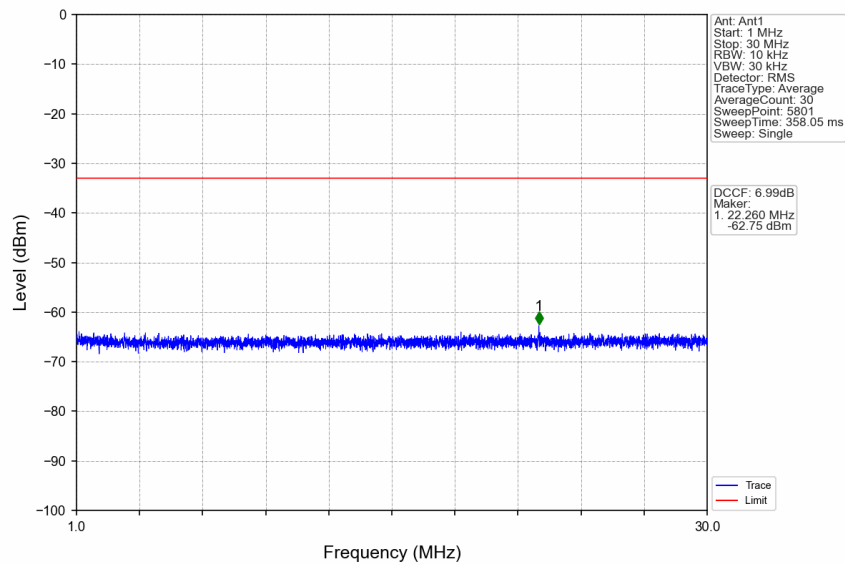
n41_15kHz_SISO_NTNV_20MHz_DFT-s-OFDM PI/2 BPSK_2593.005MHz_Edge_1RB_Left
