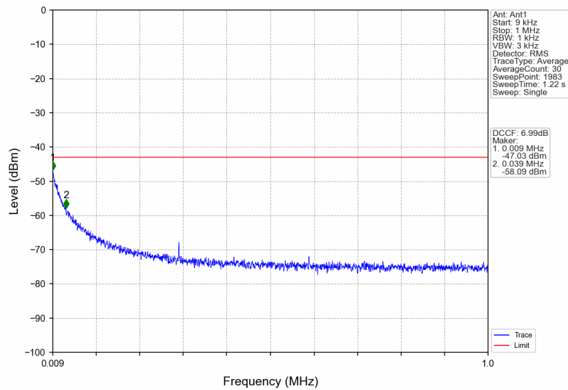
n41_15kHz_SISO_NTNV_10MHz_CP-OFDM QPSK_2685MHz_Edge_1RB_Right
