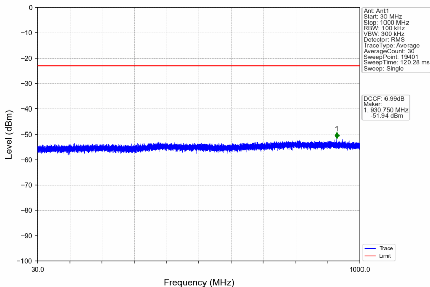
n41_15kHz_SISO_NTNV_10MHz_CP-OFDM QPSK_2685MHz_Edge_1RB_Right
