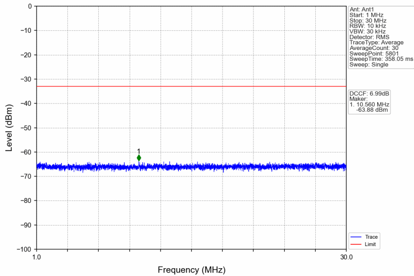
n41_15kHz_SISO_NTNV_10MHz_CP-OFDM QPSK_2593.005MHz_Edge_1RB_Left
