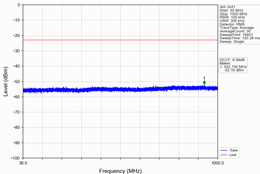
n41_15kHz_SISO_NTNV_10MHz_DFT-s-OFDM PI/2 BPSK_2593.005MHz_Edge_1RB_Left
