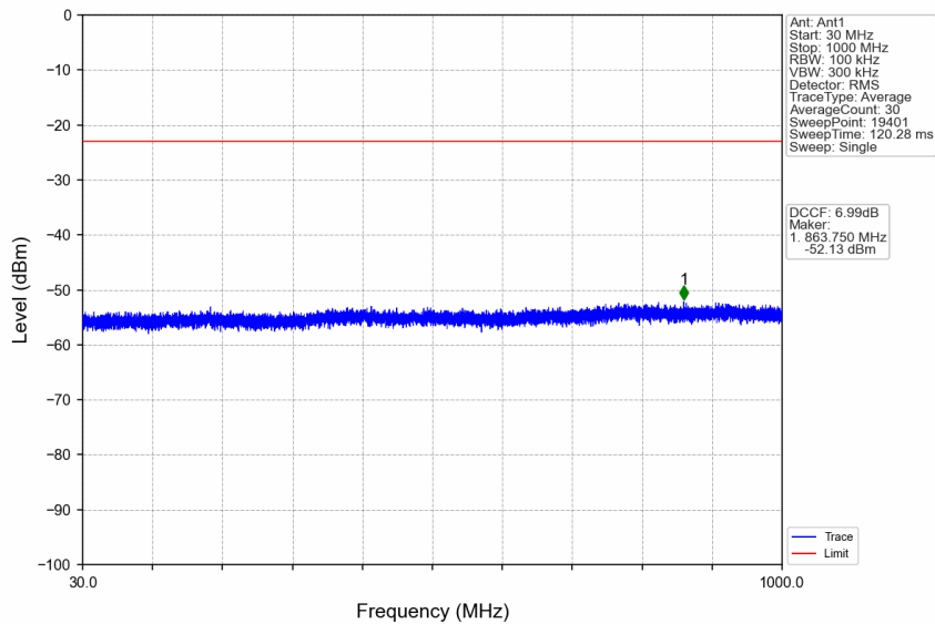
n41_15kHz_SISO_NTNV_10MHz_DFT-s-OFDM PI/2 BPSK_2501.01MHz_Edge_1RB_Left
