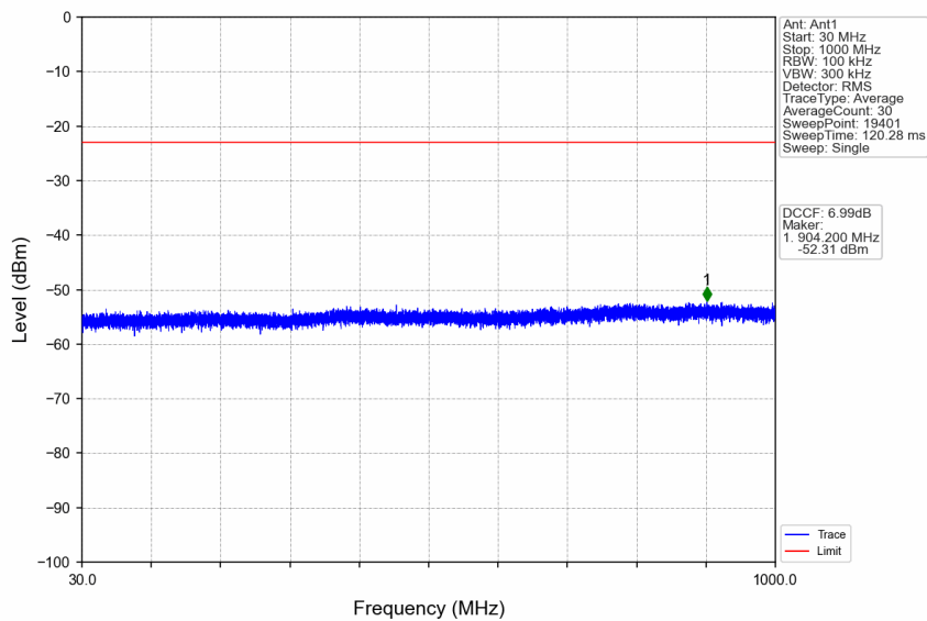
n41_15kHz_SISO_NTNV_10MHz_DFT-s-OFDM QPSK_2501.01MHz_Edge_1RB_Left
