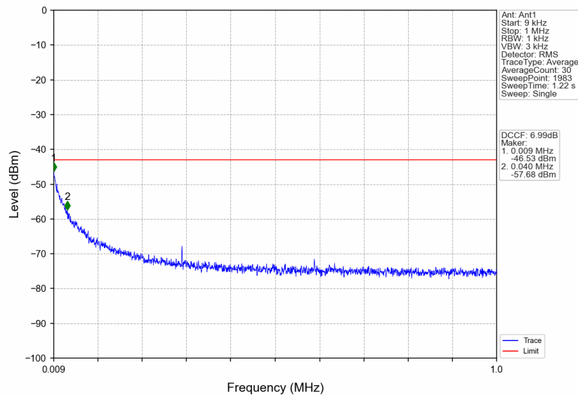
n41_15kHz_SISO_NTNV_10MHz_DFT-s-OFDM QPSK_2685MHz_Edge_1RB_Right
