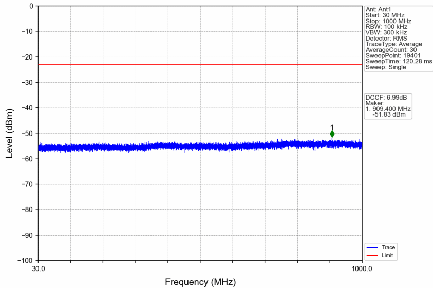
n41_15kHz_SISO_NTNV_10MHz_CP-OFDM QPSK_2593.005MHz_Edge_1RB_Left
