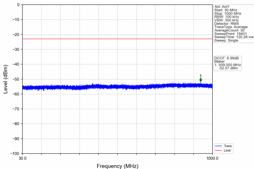
n38_30kHz_SISO_NTNV_40MHz_CP-OFDM QPSK_2590MHz_Edge_1RB_Left
