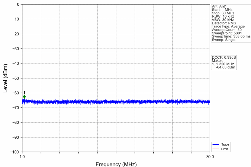
n38_30kHz_SISO_NTNV_40MHz_CP-OFDM QPSK_2590MHz_Edge_1RB_Left
