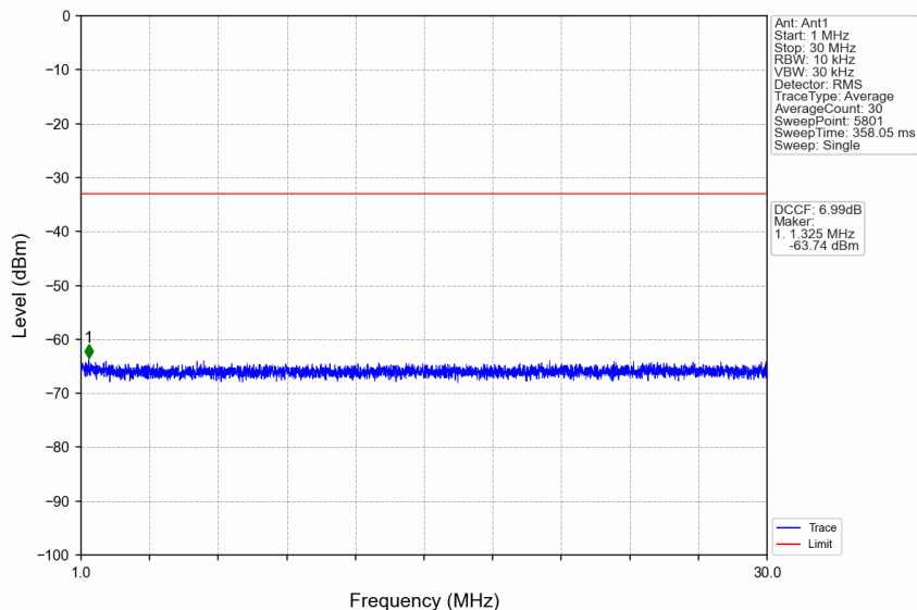
n38_30kHz_SISO_NTNV_40MHz_CP-OFDM QPSK_2595MHz_Edge_1RB_Left
