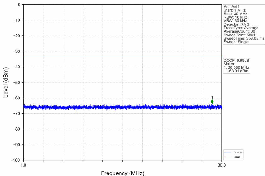
n38_30kHz_SISO_NTNV_40MHz_DFT-s-OFDM QPSK_2595MHz_Edge_1RB_Left
